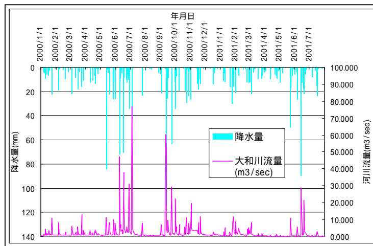
図 5-1-3 降水量および大和川流量(番条観測所)変動状況
