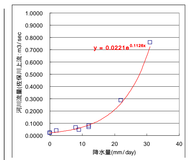
図 5-1-5 降水量と佐保川流量(上流側解析境界付近)の関係
