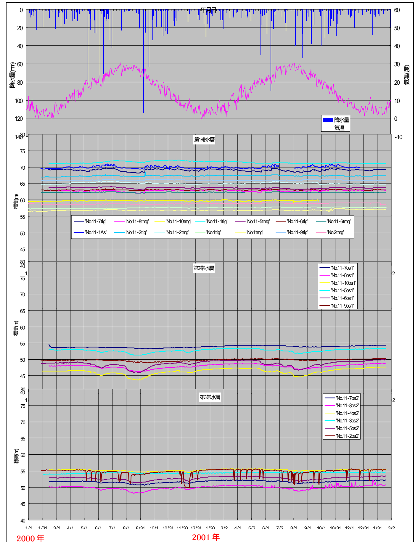
図 5-1-6 水位観測結果
