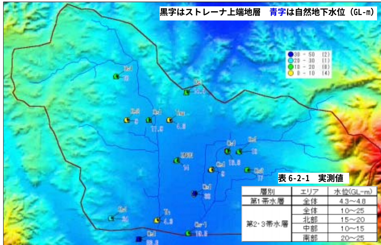
図 6-2-1 既存井戸初期水位（旧地質調査所「井戸じびき」より抜粋）
