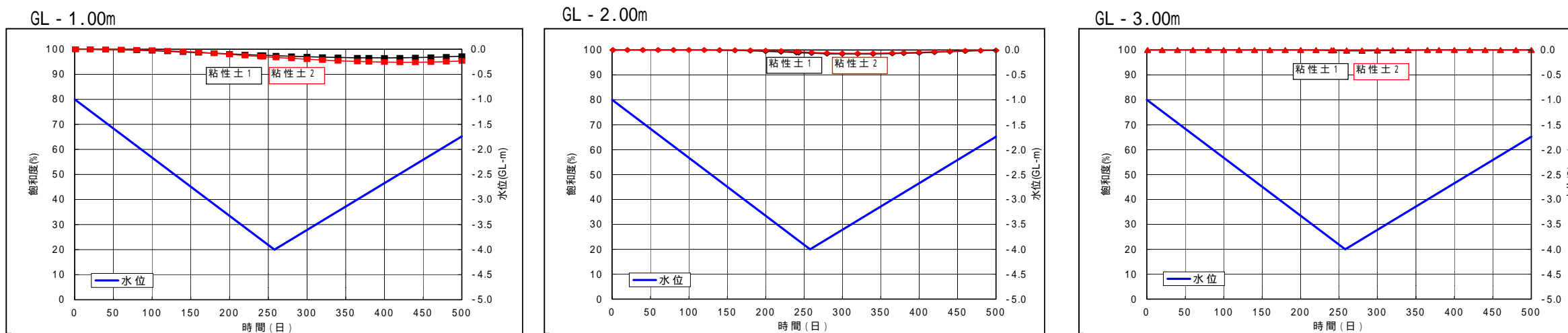
図 9-3-2 現地採取粘性土 (N011-10 地点) の飽和度変化
