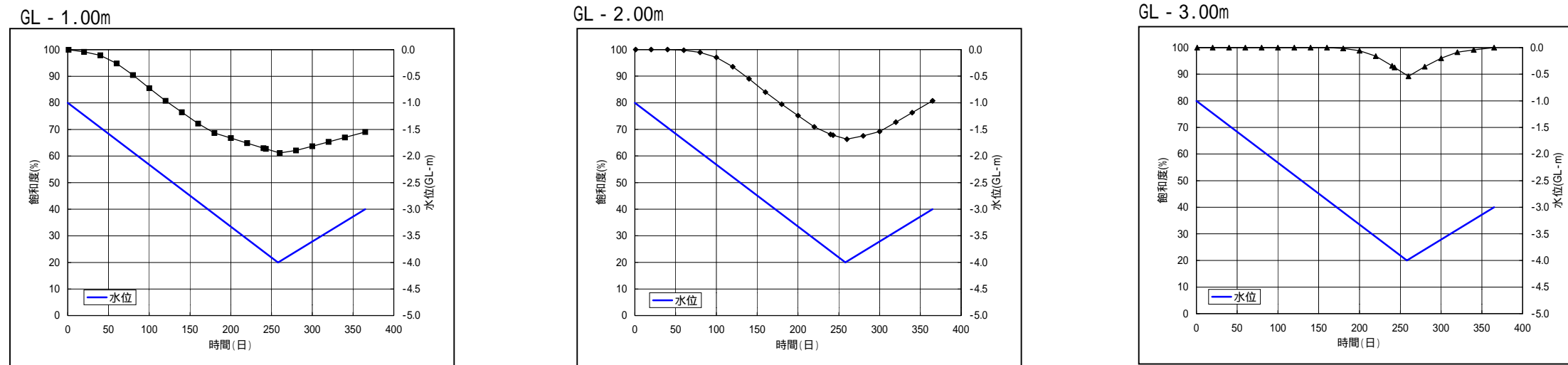
図 9-3-1 現地採取砂質土 (N02 地点) の飽和度変化
