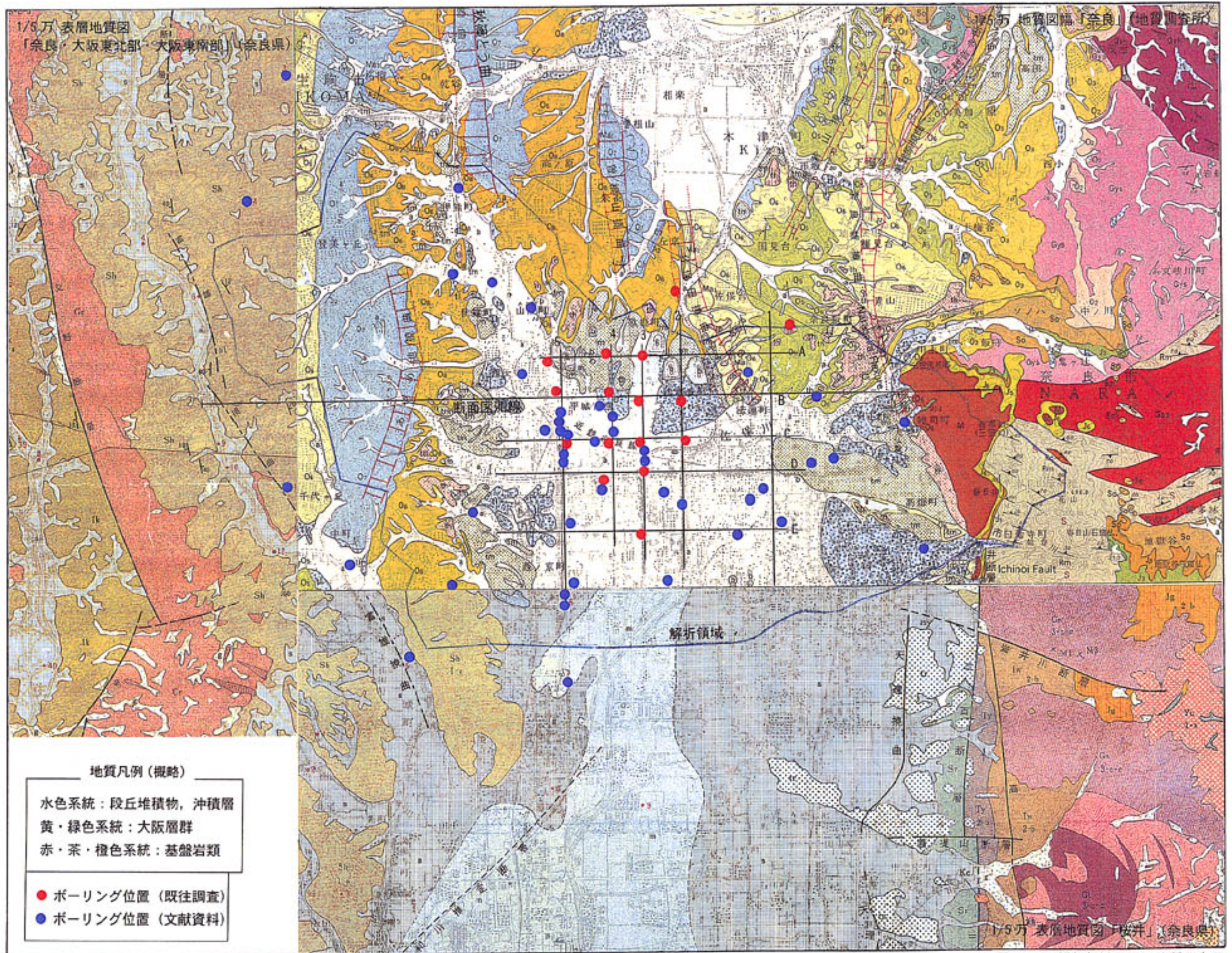
図4-4 解析領域周辺の地質分布図 (縮尺 1:50000)
