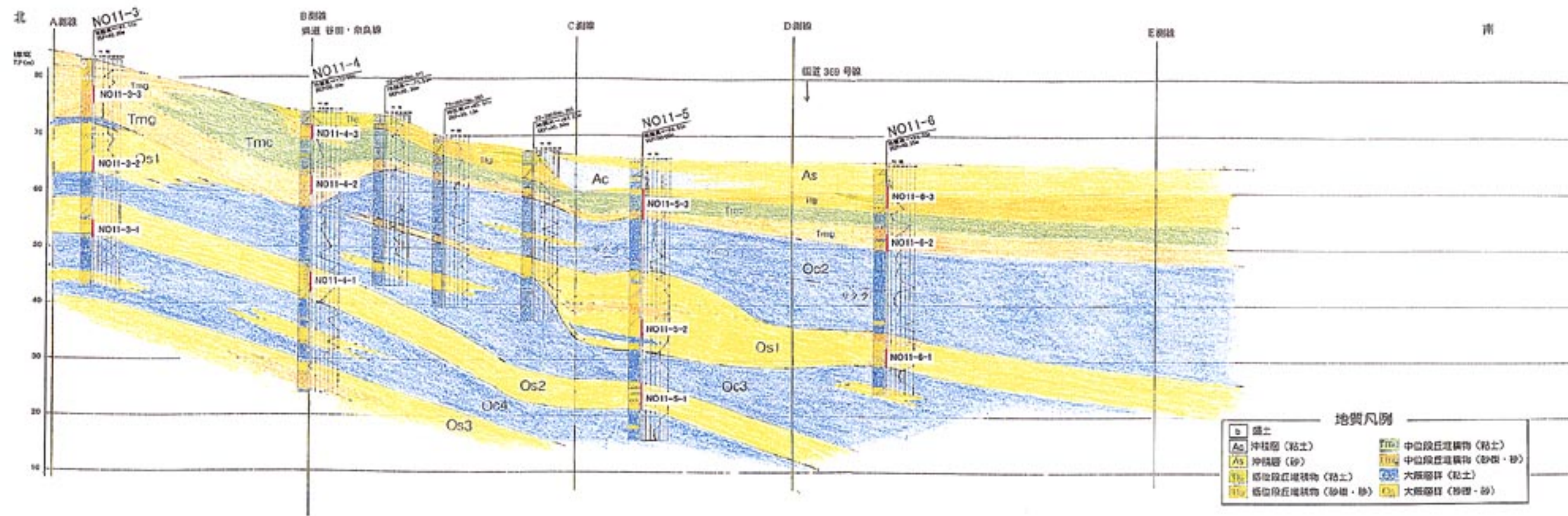
図 推定地質断面図(4測線) 縮尺 縦1:800 横1:10,000
