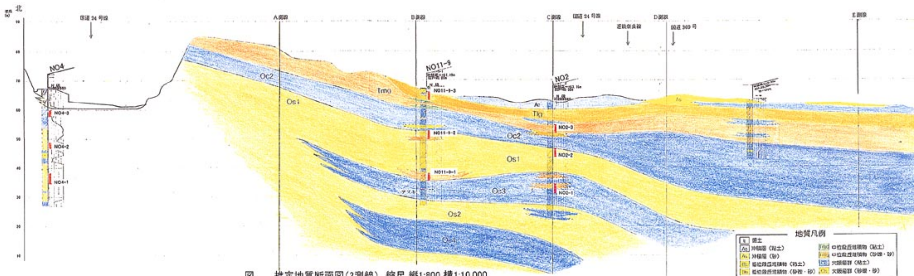
圖 推定地質断面圖(2測線) 縮尺 縱1:800 橫1:10,000
