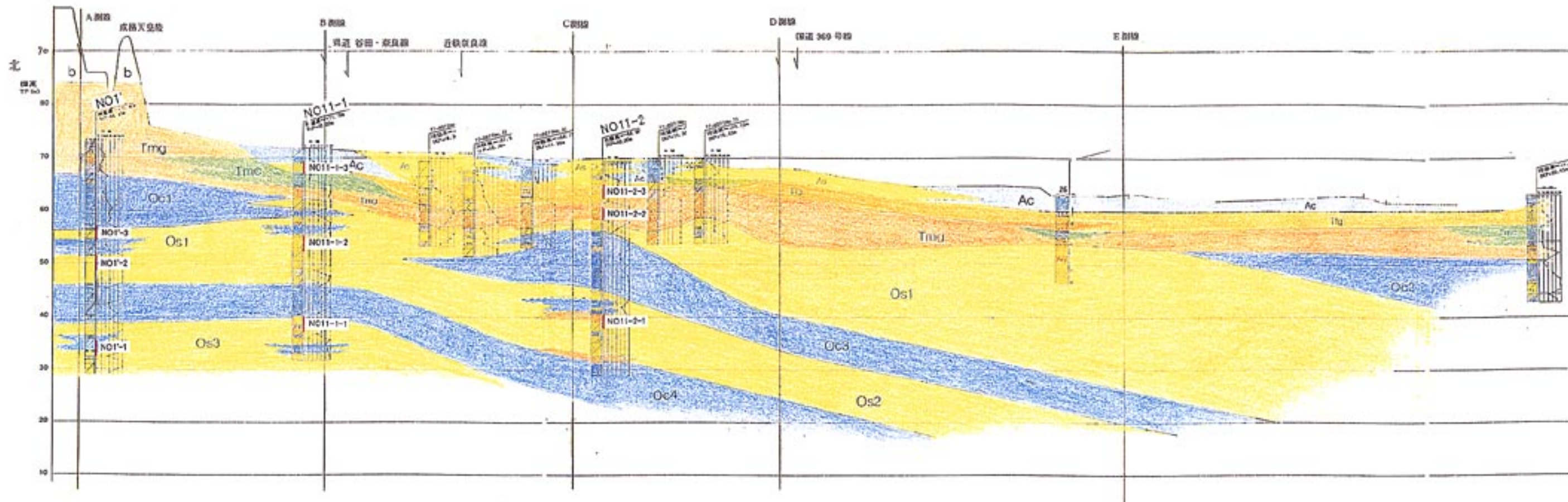
推定地質断面図(5測線) 縮尺 縦1:800 横1:10,000
