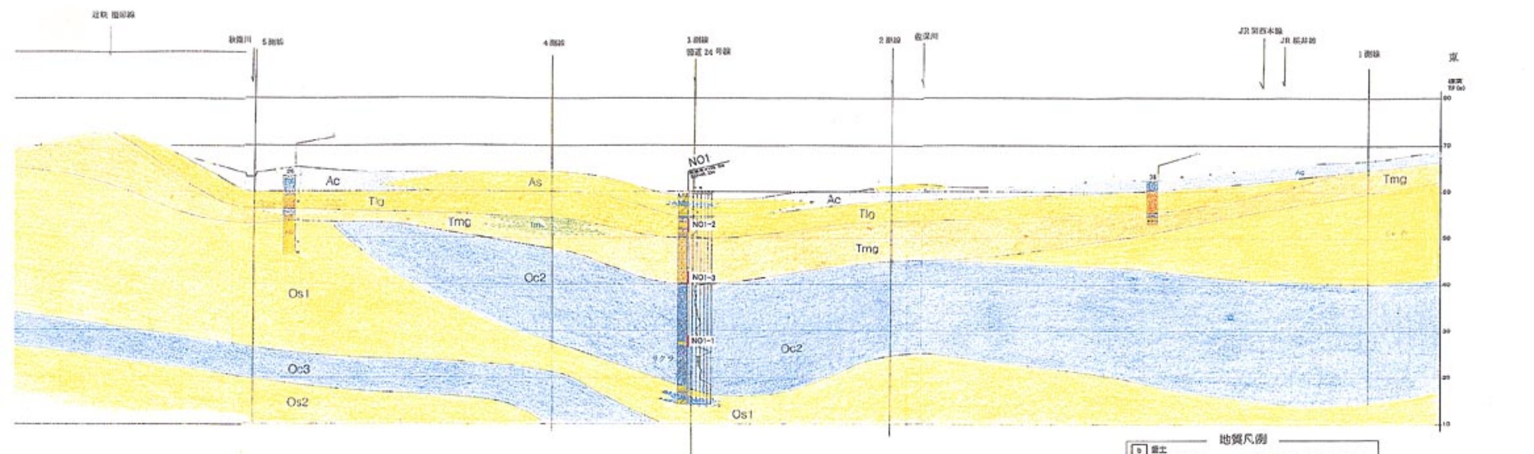
図 推定地質断面図(E測線) 縮尺 縦1:800 横1:10,000
