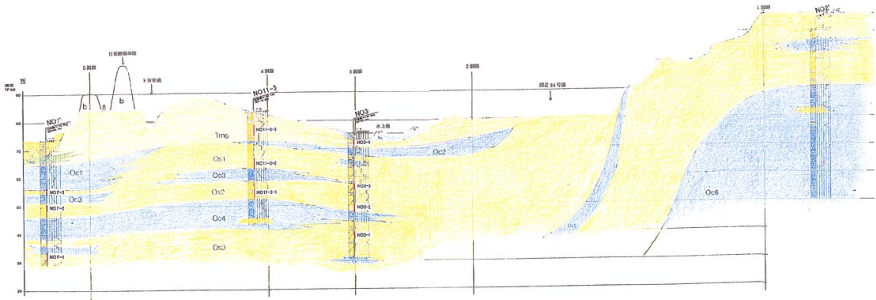
圖 推定地質断面圖(A測線) 縮尺 縱1:800 橫1:10,000
