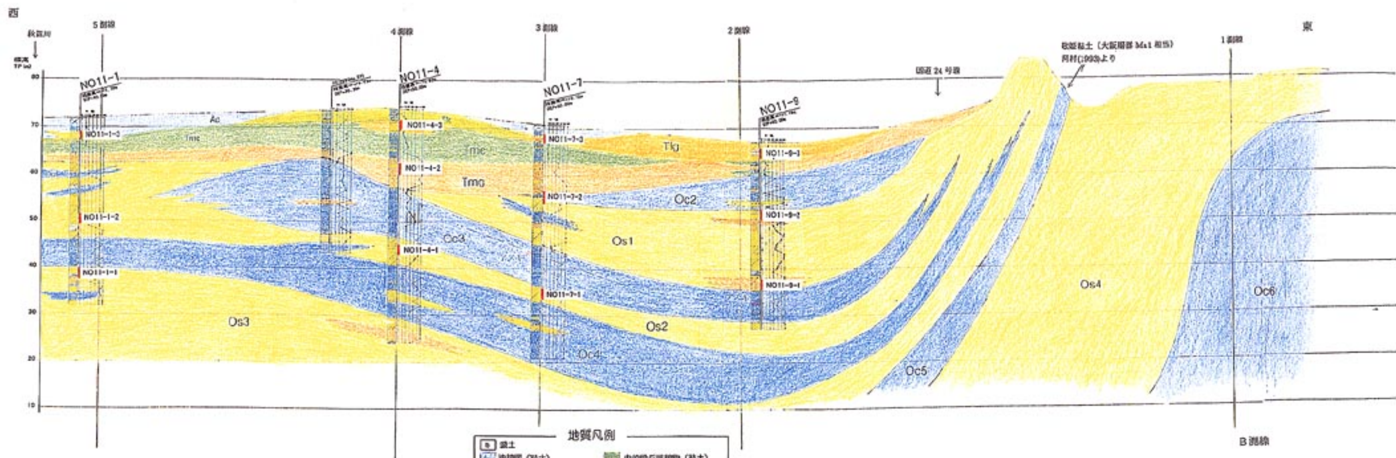
図 推定地質断面図(B測線) 縮尺 縦1:800 横1:10,000
