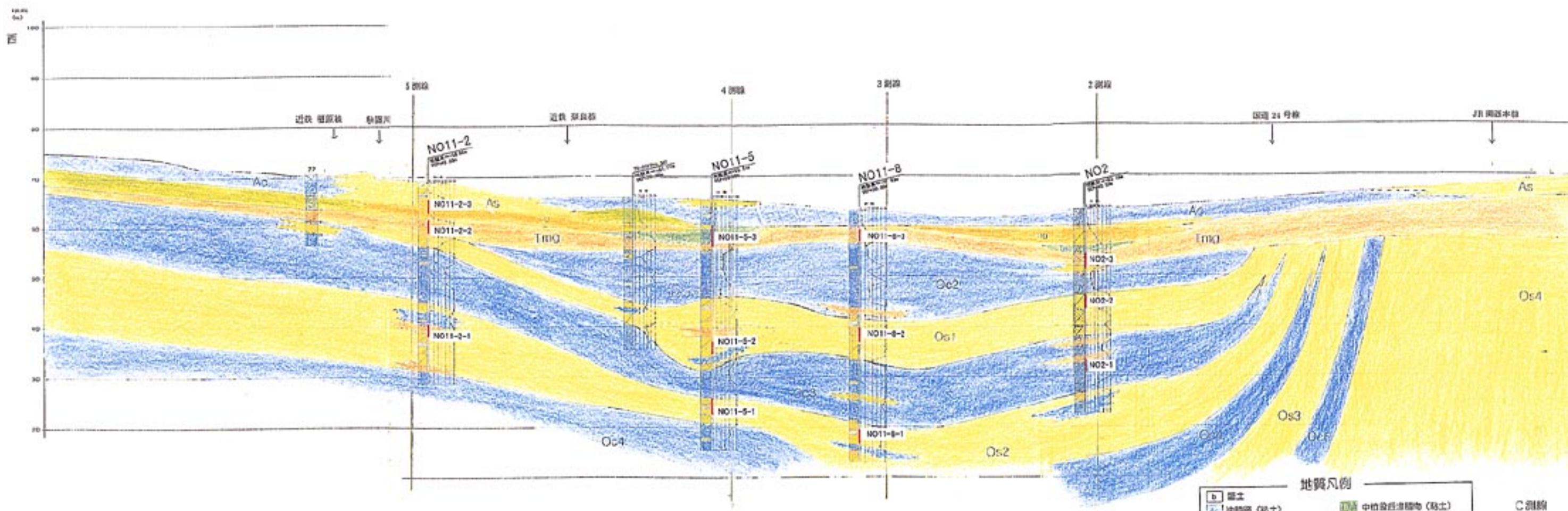
図 推定地質断面図(C測線) 縮尺 縦1:800 横1:10,000
