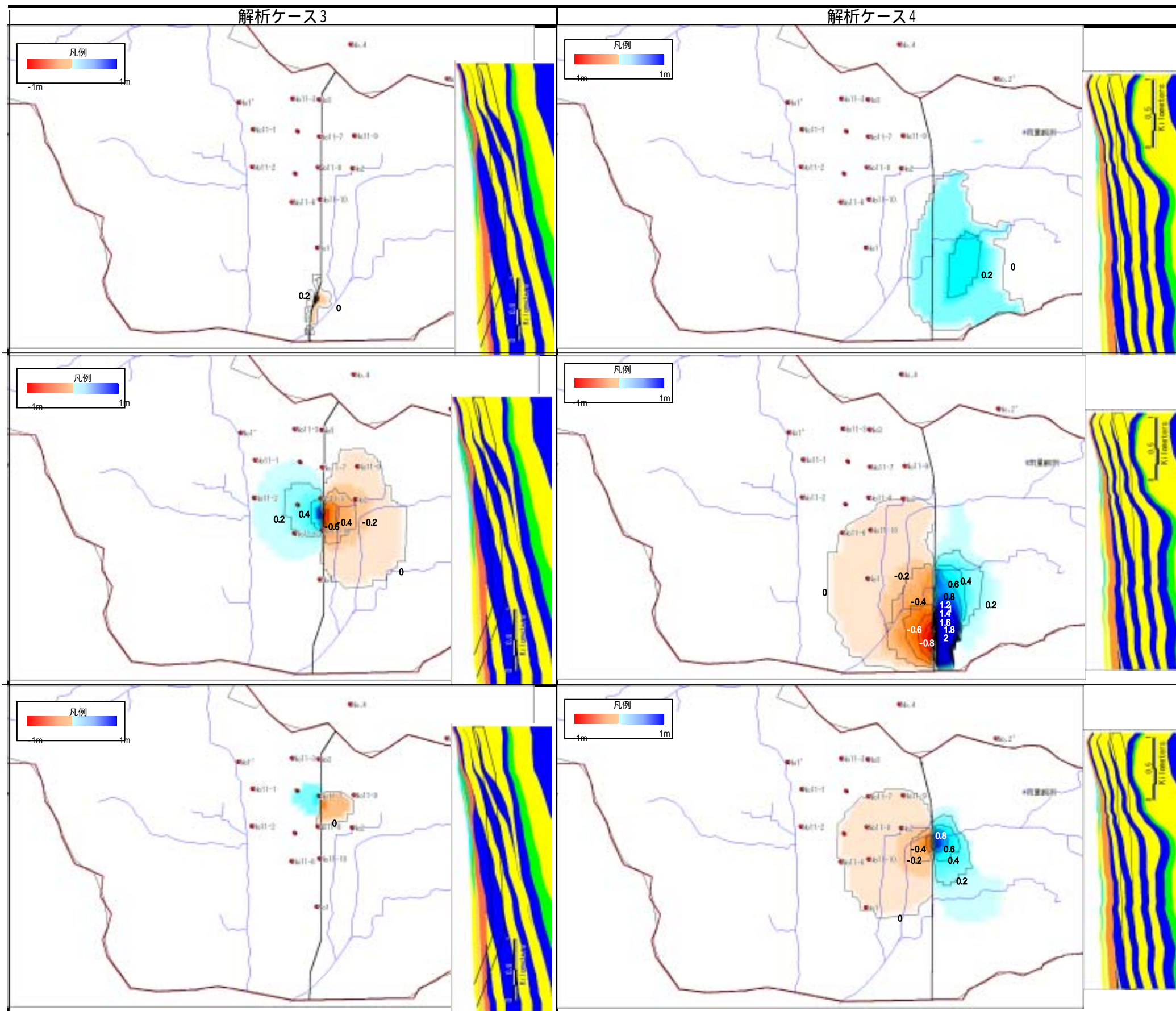
図5-3 構造物の有・無による地下水位の差
