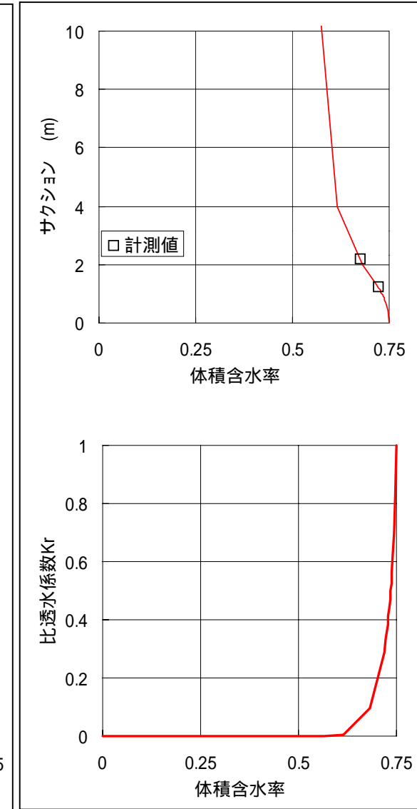
図 5-4 現地採取粘性土 2 (NO11-10 地点) の不飽和特性曲線
