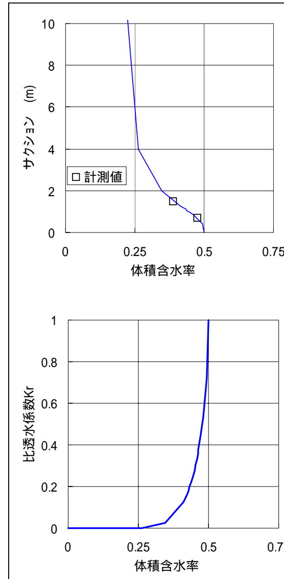
図 5-2 現地採取砂質土 (NO2 地点) の不飽和特性曲線
