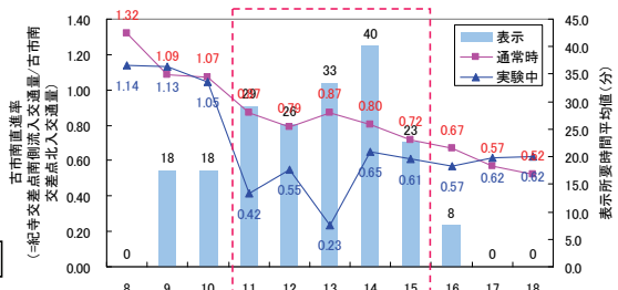
国道169号北行き交通量の変化と所要時間情報の関係
