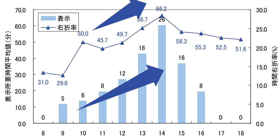
般若寺交差点提供情報と右折率
