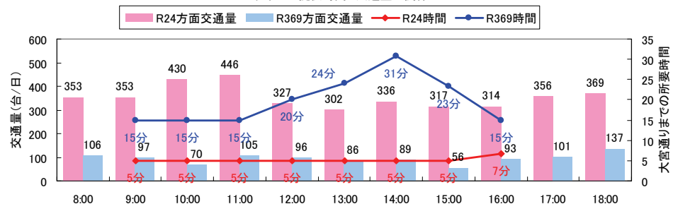
木津川IC提供時間と交通量の関係
