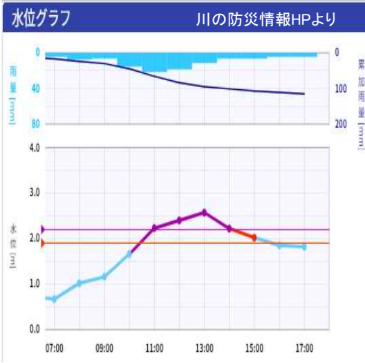
地蔵院川 下三橋 水位グラフ
