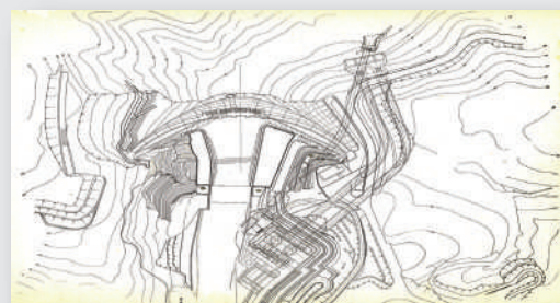
天ヶ瀬ダム平面図
