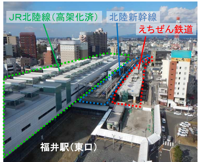
整備中(高架化)
