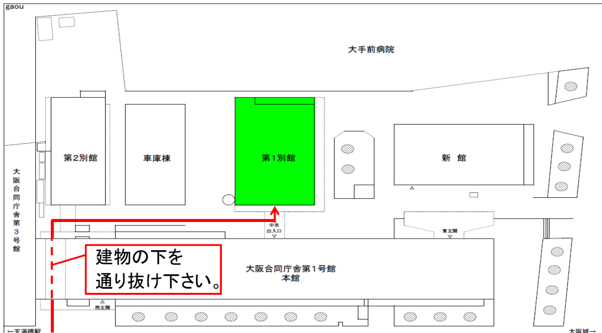
大阪合同庁舎第1号館 詳細図
