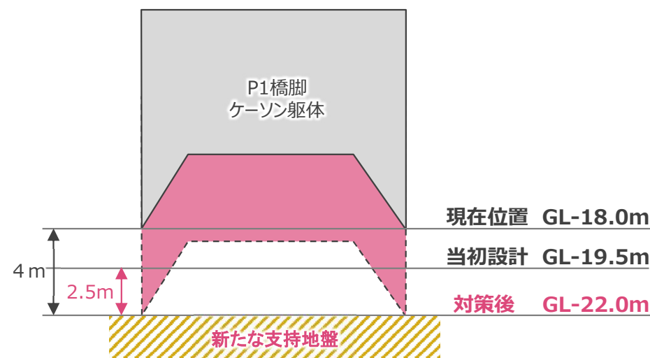
図 2 対策イメージ（ケーソン躯体の延伸）
