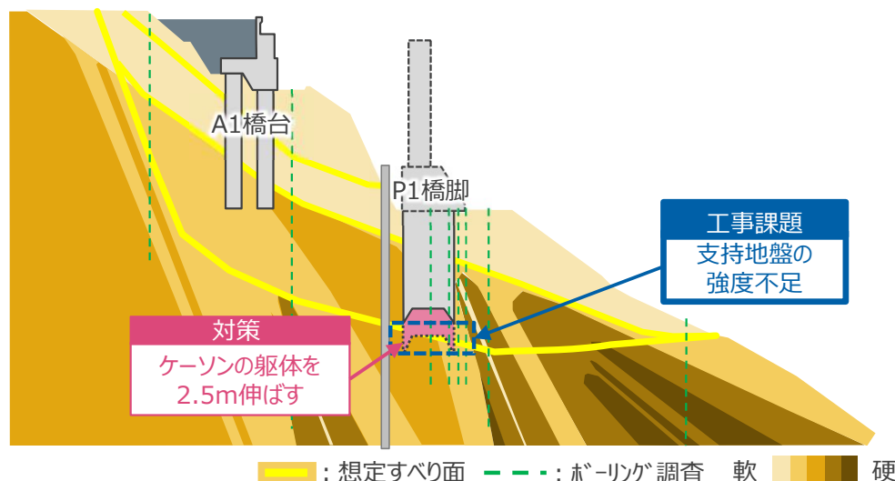
図 1 工事課題と対策
