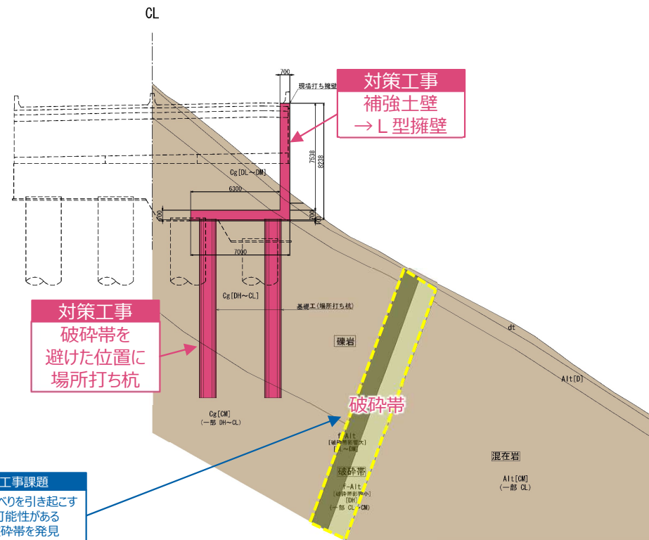
■ 図2 本設時の詳細設計結果
