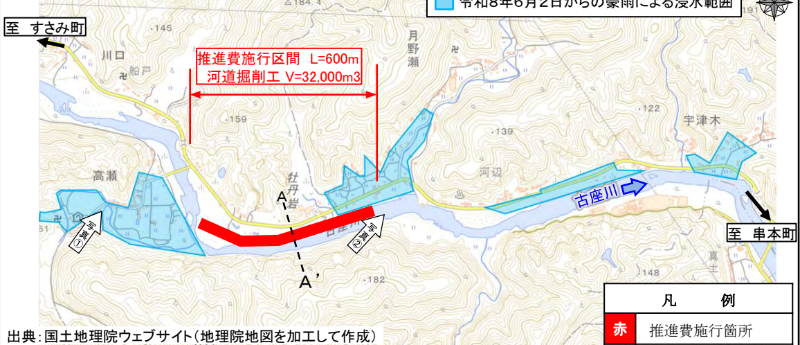
【平面図】
