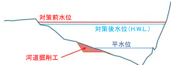
【断面図】
