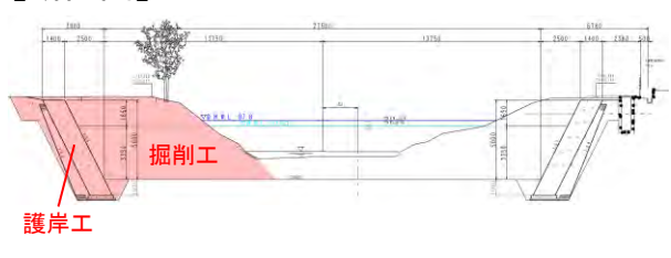
【断面図】
