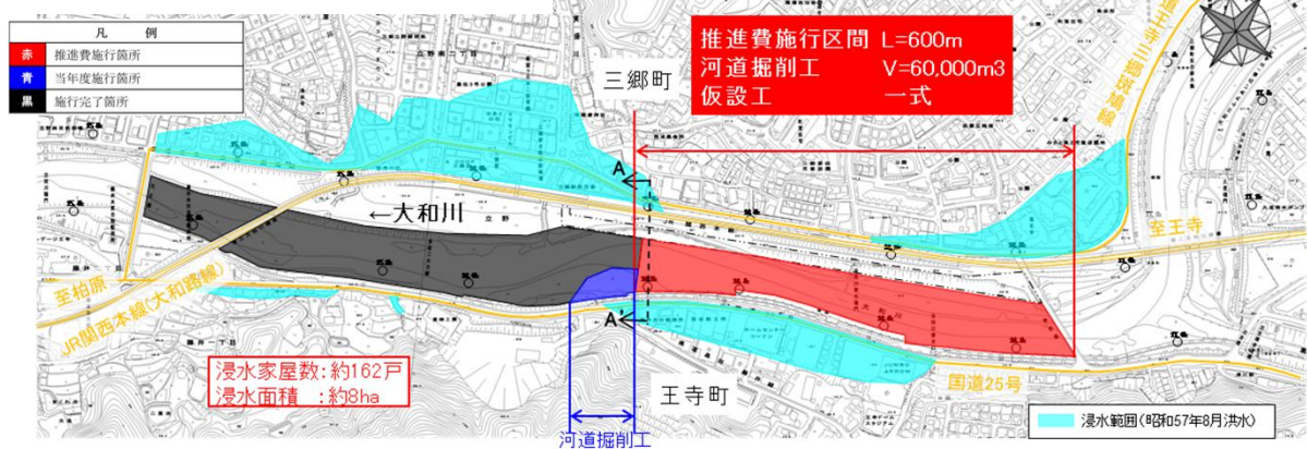
【平面図(立野・藤井地区)】
