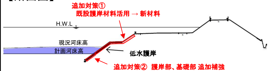
【断面図】
