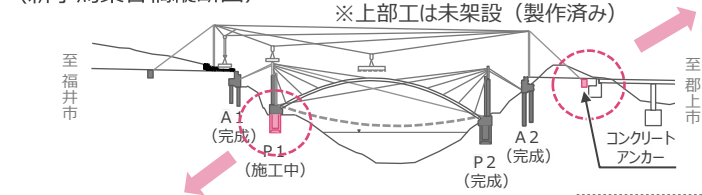
(新子馬巢谷橋縦断面図)
