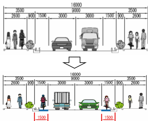
■深井73号線 現況断面
