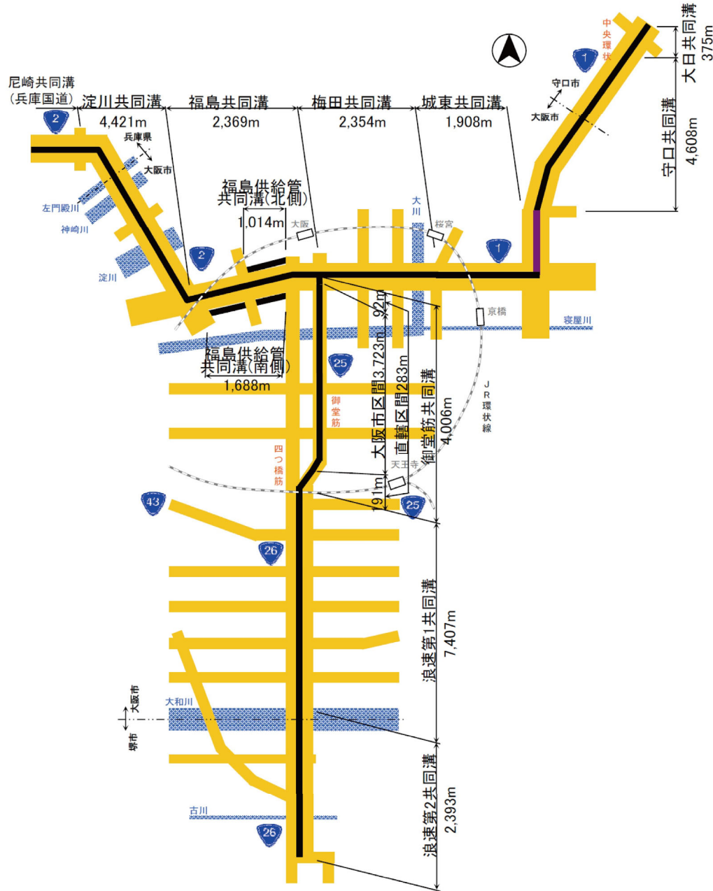
国道1号、2号、25号、26号（大阪市～泉北地域）共同溝
