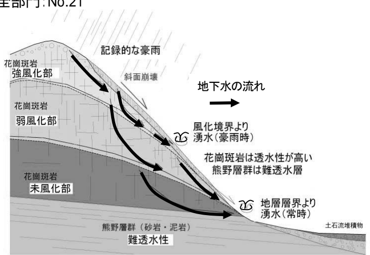
図-8 熊野層群・花崗斑岩層界付近の崩壊機構概念図
