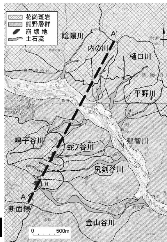
図-2 那智川中流域地質平面図
