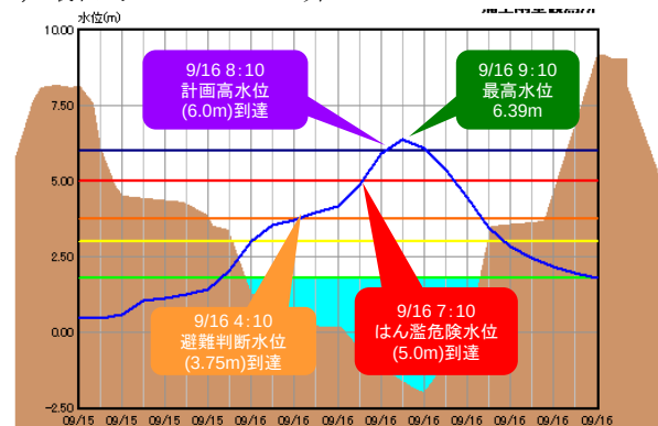
図2 日野川安吉橋の水位グラフ (2013年9月15~16日)
