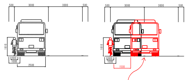
図-7 自転車と自動車の走行部分と追い抜くときの状態
