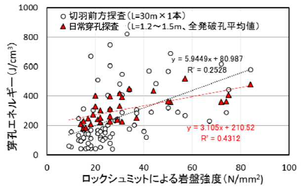
図-18 穿孔エネルギーと岩盤強度の関係
