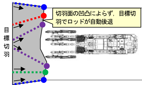
図5 オートリターン機能 概要図
