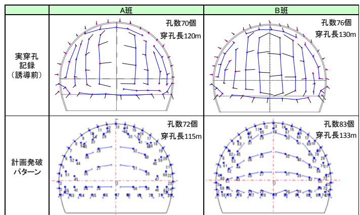
図-15 実穿孔記録と計画発破パターン (II N パターン)
