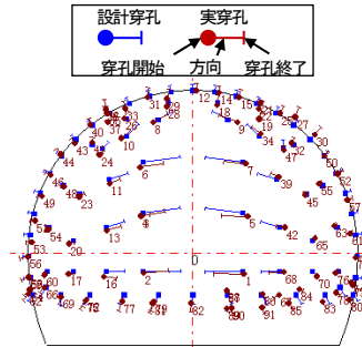
図-7 実穿孔記録表示例
