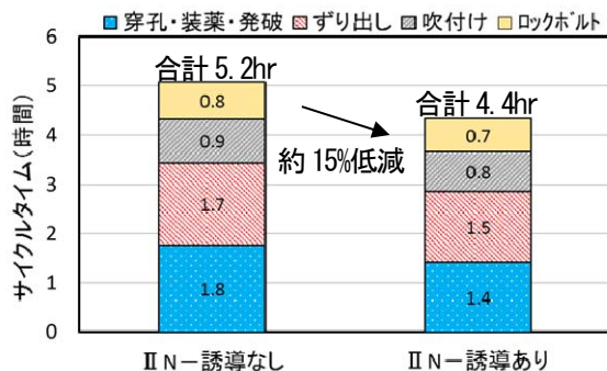
図-12 サイクルタイム測定結果 (II N パターン)
