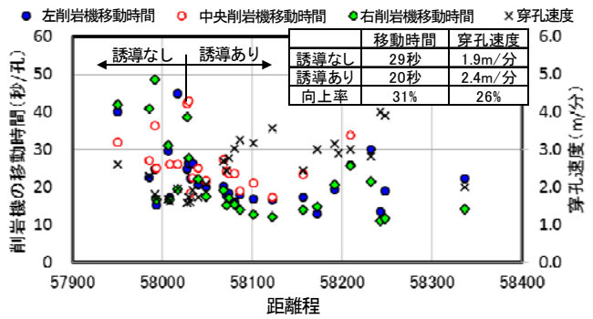
図-13 穿孔速度測定結果
