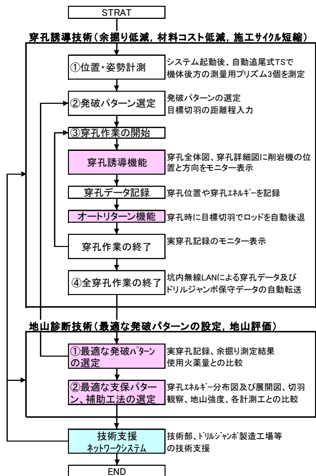
図-1 全断面追尾式穿孔誘導システム「ドリルNAVI」の概要
