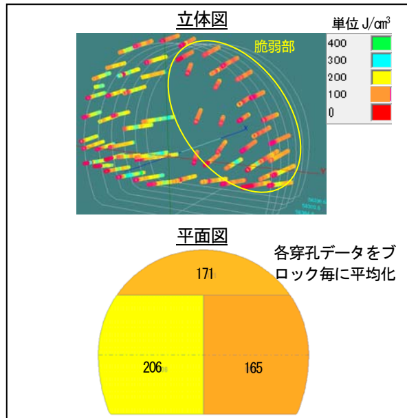
図-8 穿孔エネルギー分布図
