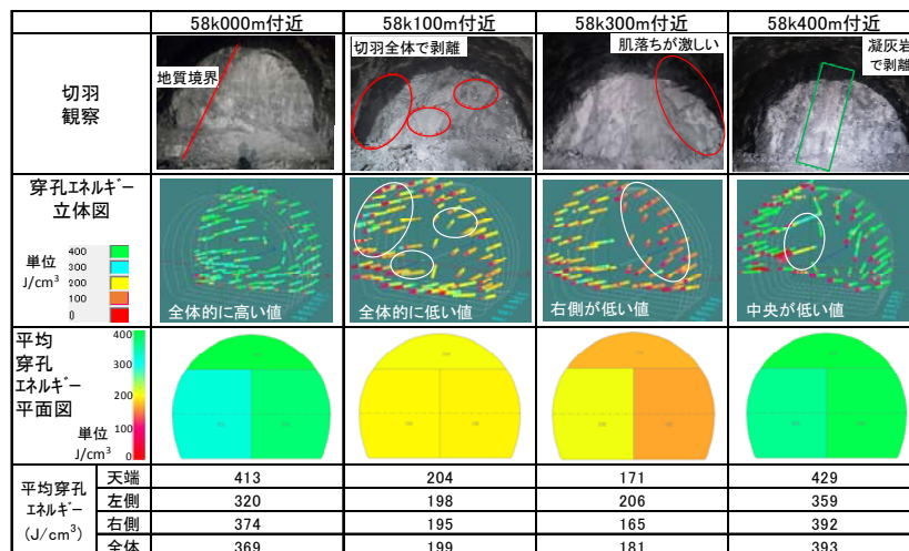
図-17 切羽観察記録と穿孔エネルギーの関係
