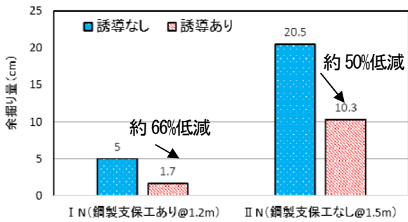
図-11 余掘り測定結果
