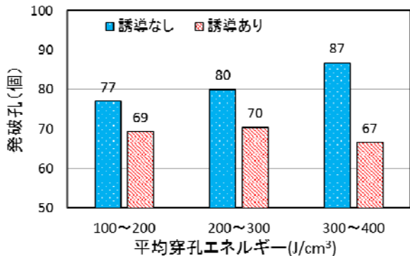
図-14 発破孔数測定結果 (II N パターン)
