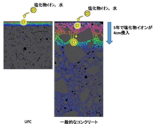
図-5 塩化物浸透試験
