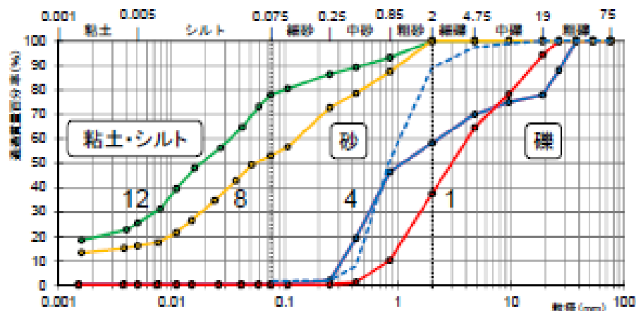
粒度分布図
