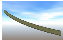
コンクリートブロック張 3次元設計データ
