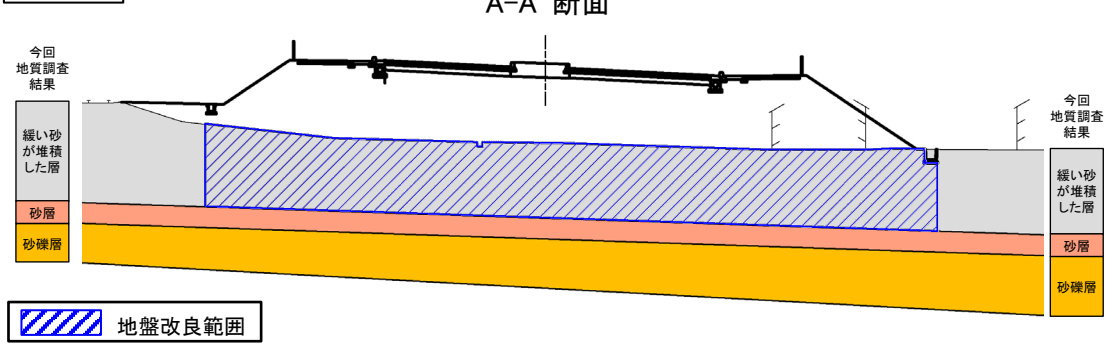
横断面図
