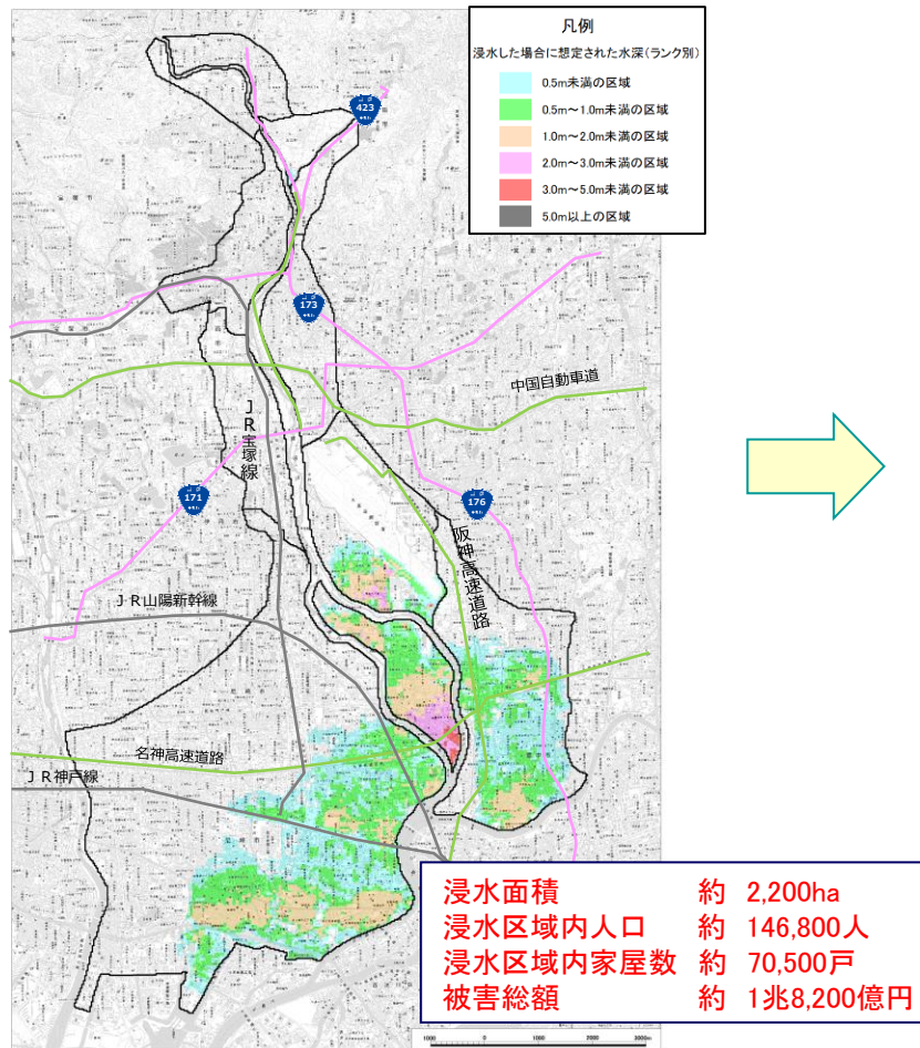
現況河道（R8時点）の氾濫想定 （昭和35年洪水×1.1）
