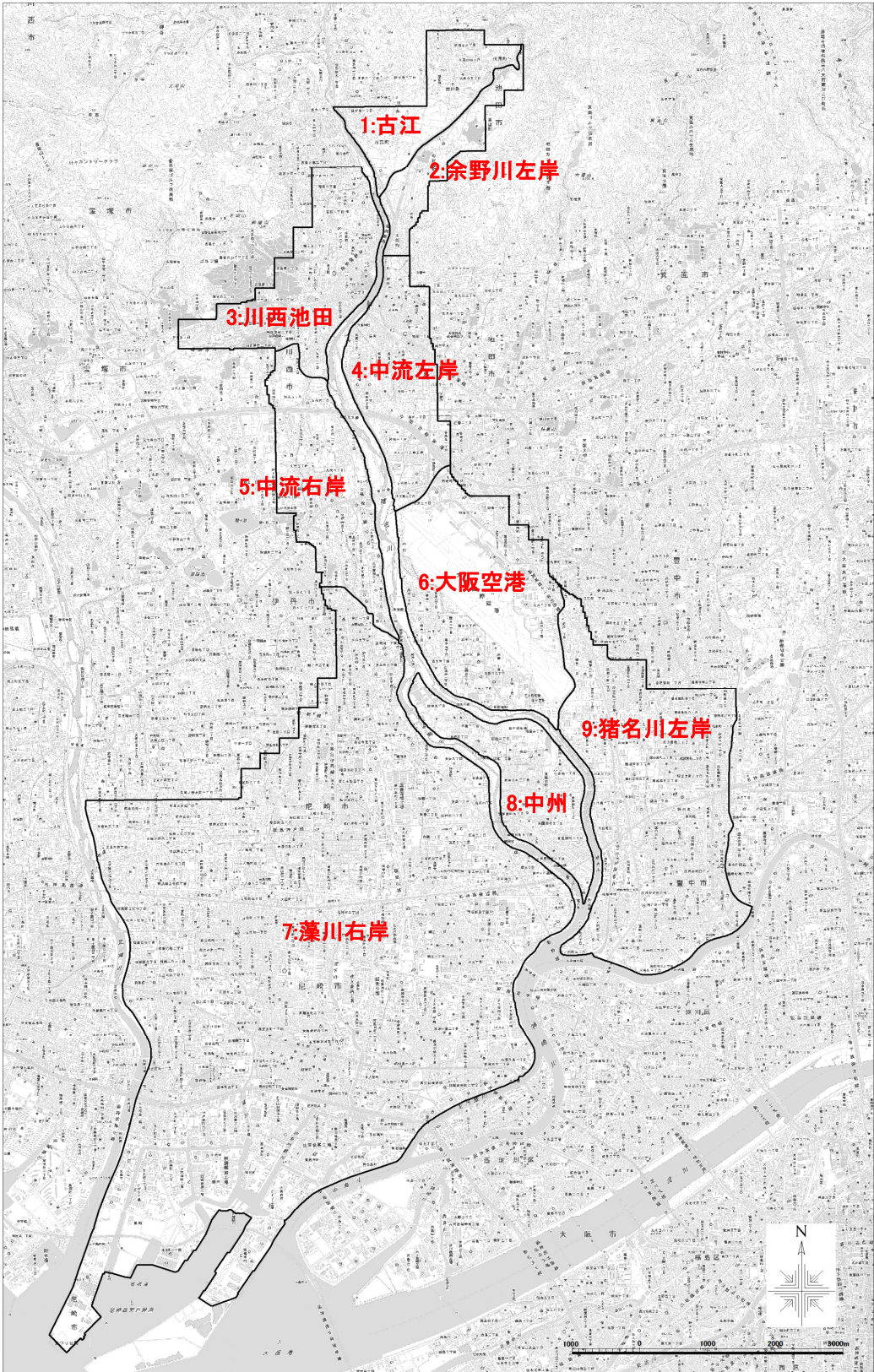
様式－１ 氾濫ブロック分割図
