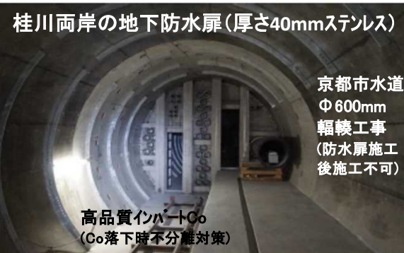
桂川両岸の地下防水扉(厚さ40mmステンレス) 京都市水道 Φ600mm 輻輳工事 (防水扉施工後施工不可) 高品質インポートCo (Co落下時不分離対策)
