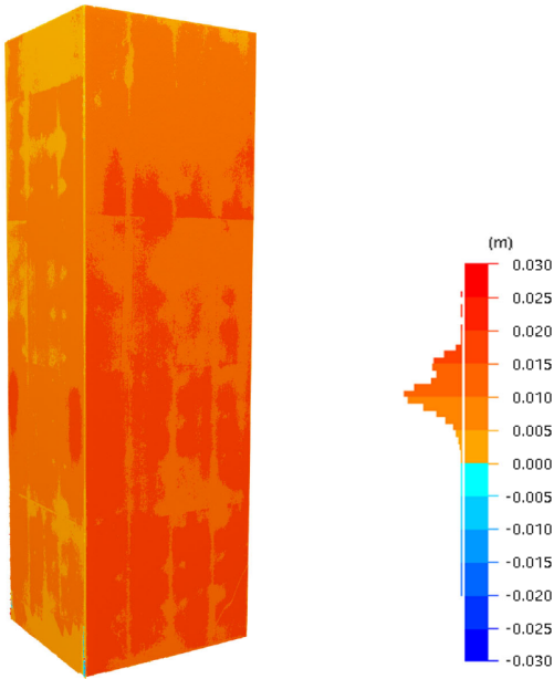
3次元測量データと設計値の比較
