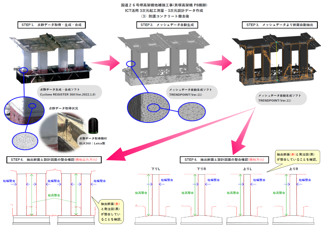
3次元測量データと設計値の比較
