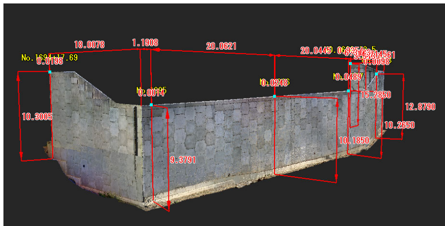
補強土壁出来形（レーザースキャナによる測定）
