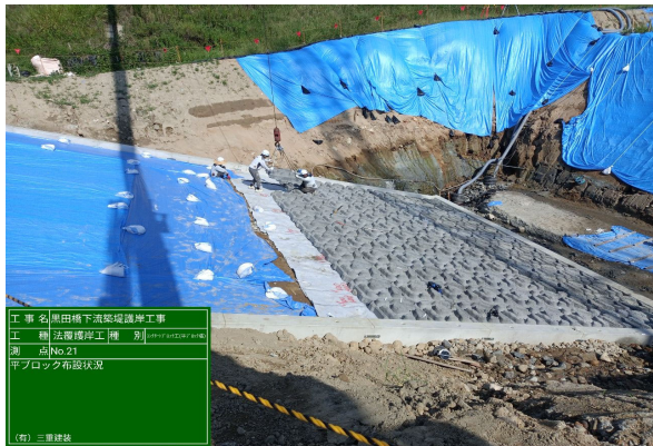
■黒田地区引堤区間 名張大橋延伸条件護岸 L=13m (平ブロック張の施工状況)
