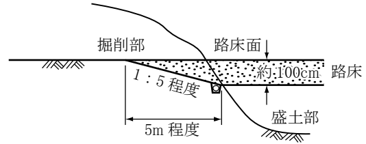
(c) 現地盤がすり付け区間を長くすることが不経済となる場合
