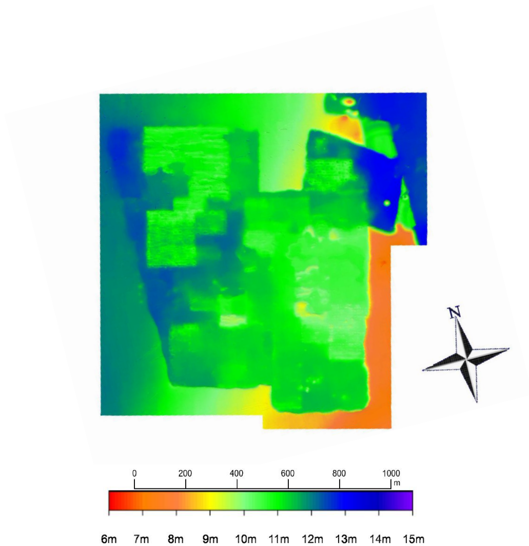
図 54 水深図（測量日：令和 6 年 1 月 17、18、22 日）
