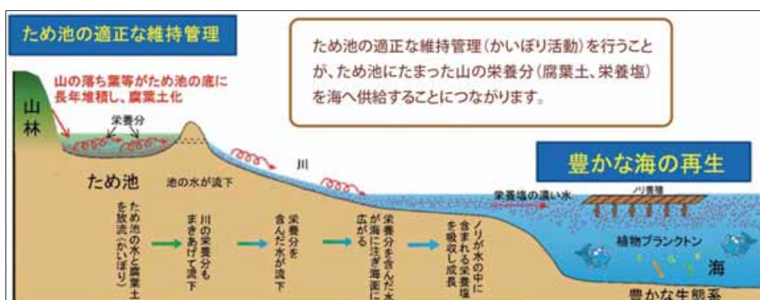
図 1-51 ため池の池干し（かいぼり）のイメージ
