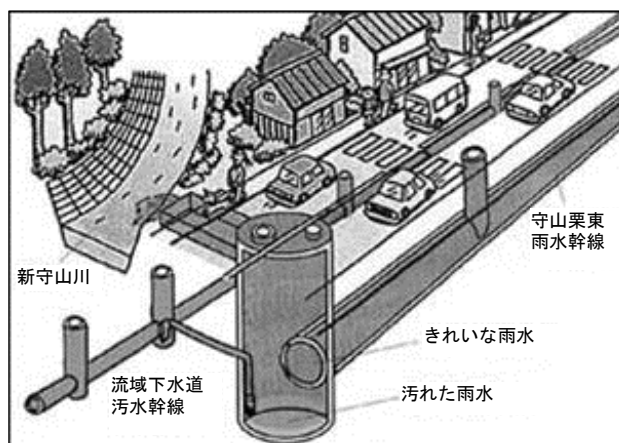
図 1-5 雨水幹線のイメージ
