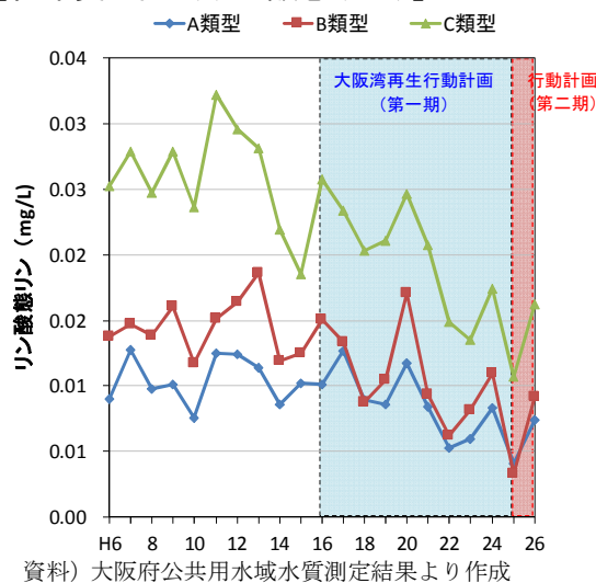
図 1-27 リン酸態リンの経年変化（表層、年平均値）
