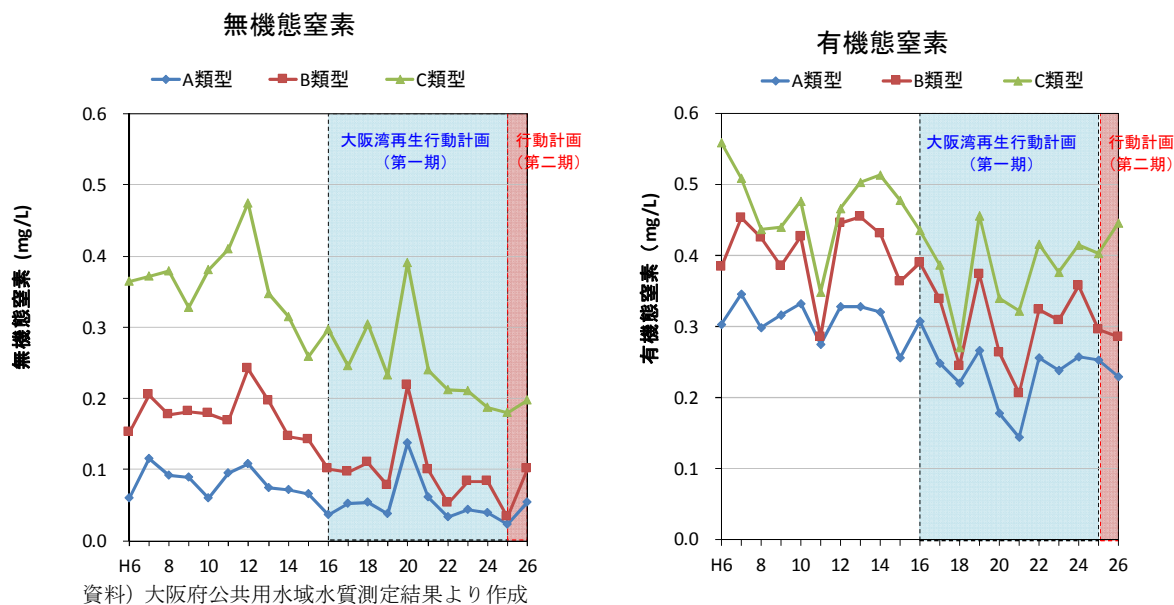
図 1-26 形態別窒素の経年変化（表層、年平均値）
