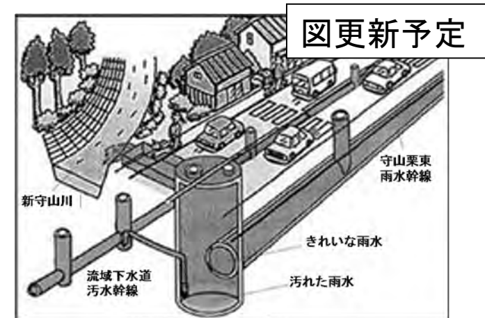
雨水幹線のイメージ
