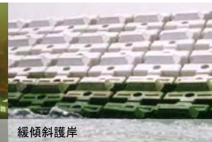
新島の緩傾斜護岸
