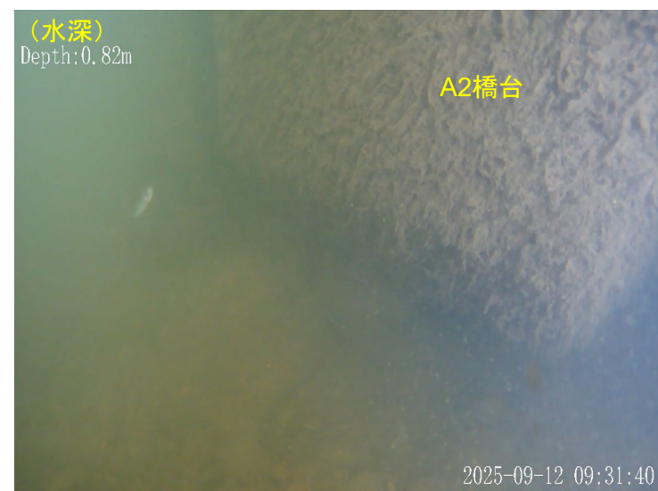
写真-4 A2橋台(護床工)(健全)
