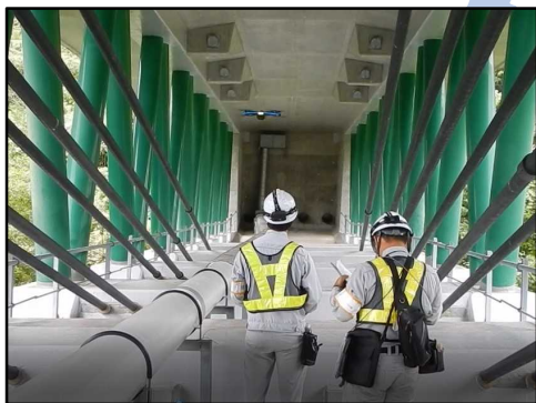
ドローンによる橋梁上部工の点検 国道42号木ノ川高架橋（和歌山県新宮市）
