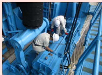
ダム放流設備（ゲート）の点検
