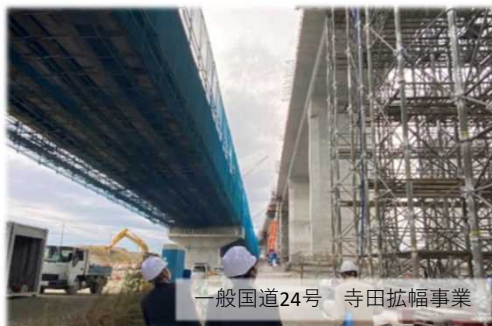
一般国道24号 寺田拡幅事業 2車線から4車線に拡幅するため、高架構造による上り線（2車線）を建設中！
