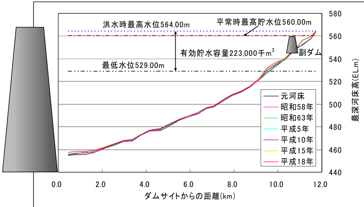
図 4.4-1 堆砂形状縦断図（九頭竜川本川）
