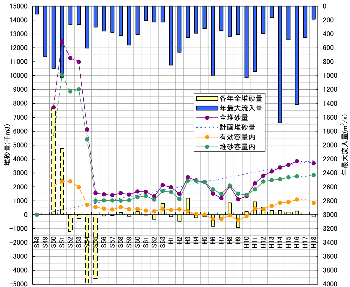
図 4.3-1 堆砂量の経年変化
