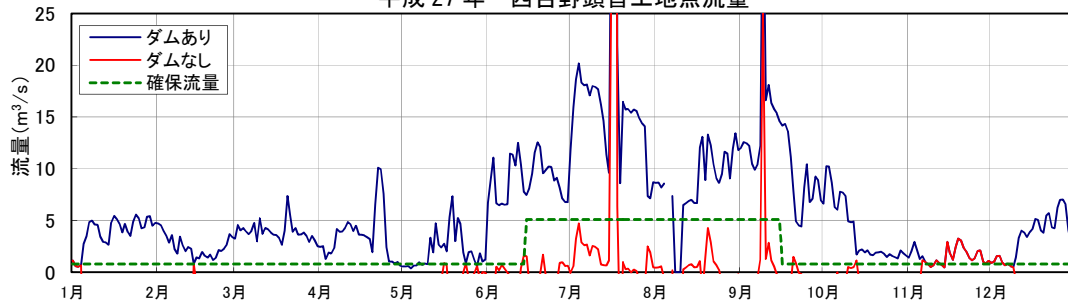
図 3.4.1-22 平成 27 年の猿谷ダムの貯水位・流入量・放流量、西吉野頭首工地点の流量変化
