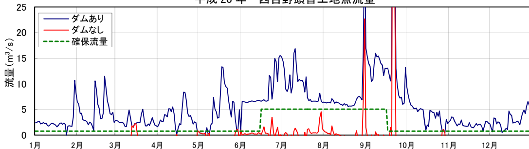
図 3.4.1-23 平成 28 年の猿谷ダムの貯水位・流入量・放流量、西吉野頭首工地点の流量変化
