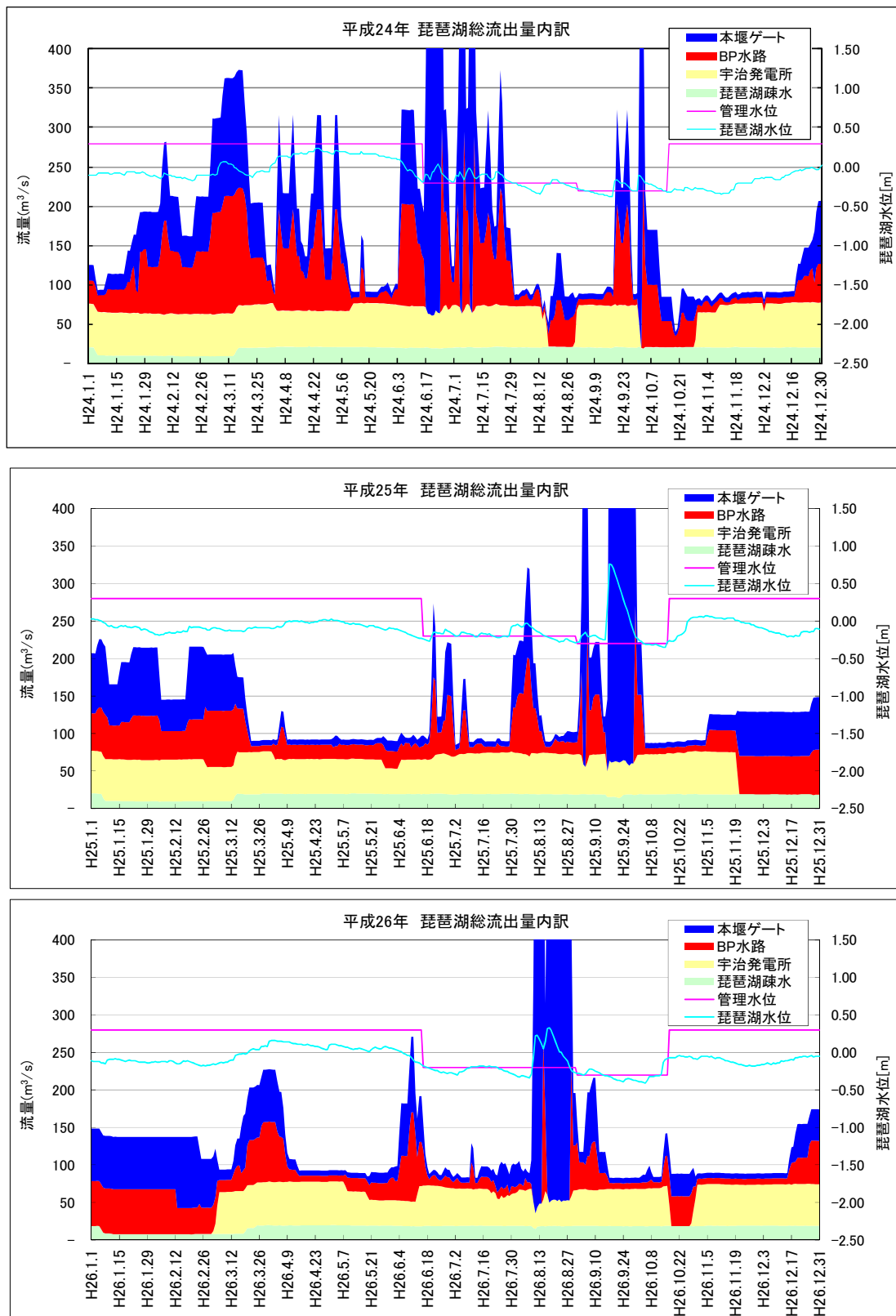
図 3.3-9 琵琶湖水位及び流出量内訳 (2012年(平成24年)～2014年(平成26年))
