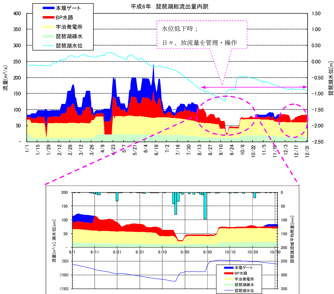
図 3.4.3-1 琵琶湖水位低下時におけるバイパス水路による放流量の微調整(1994年(平成6年))
