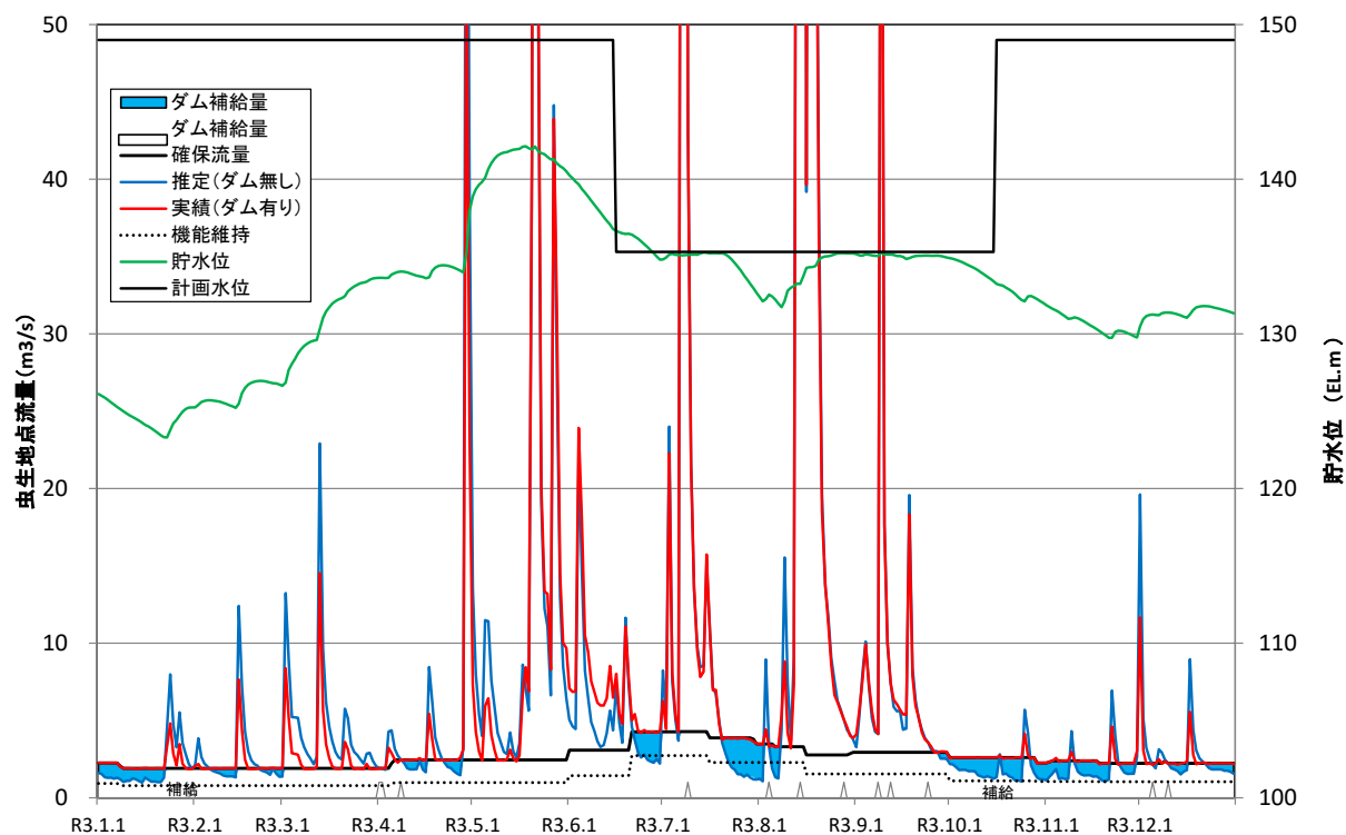
図 3.4-3(8) 虫生地点の確保流量と流量実績ほか(令和3年)
