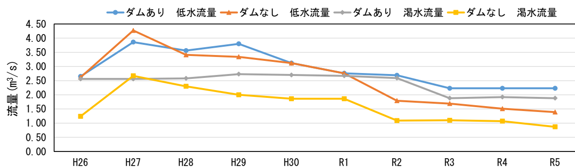
図 3.4-2 虫生地点流況のダムありなしの比較（低水・渇水流量）
