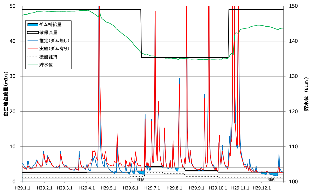
図 3.4-3(4) 虫生地点の確保流量と流量実績ほか(平成 29 年)
