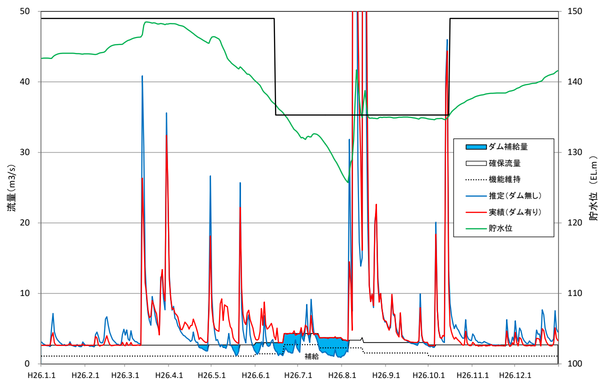
図 3.4-3(1) 虫生地点の確保流量と流量実績ほか(平成 26 年)
