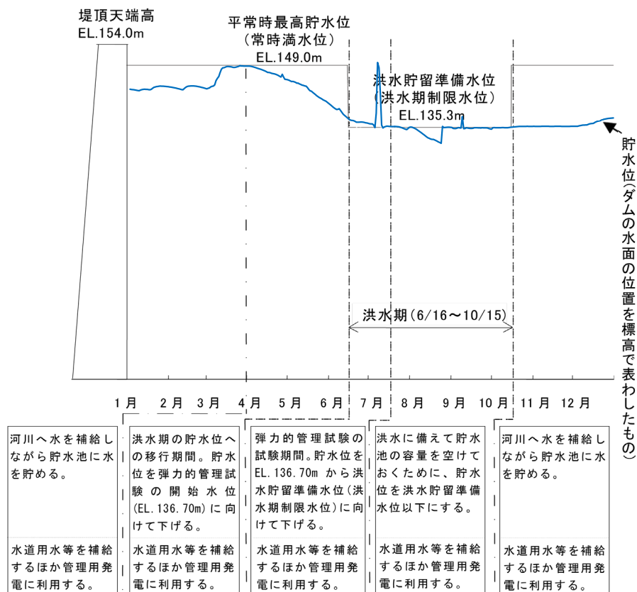
図 3.2-2 貯水池運用計画
