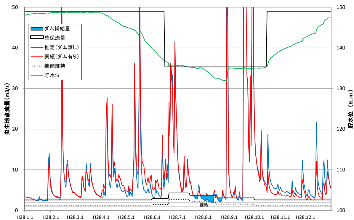
図 3.4-3(3) 虫生地点の確保流量と流量実績ほか(平成 28 年)
