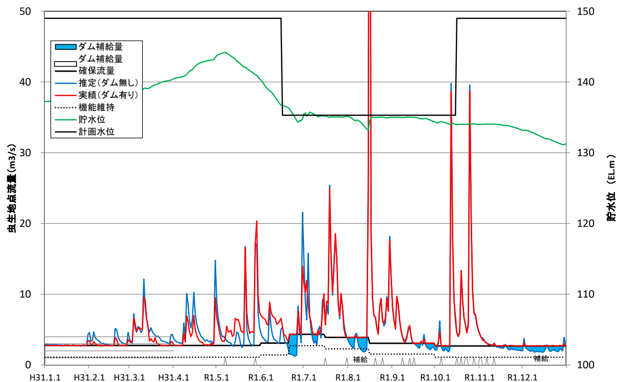
図 3.4-3(6) 虫生地点の確保流量と流量実績ほか(令和元年)
