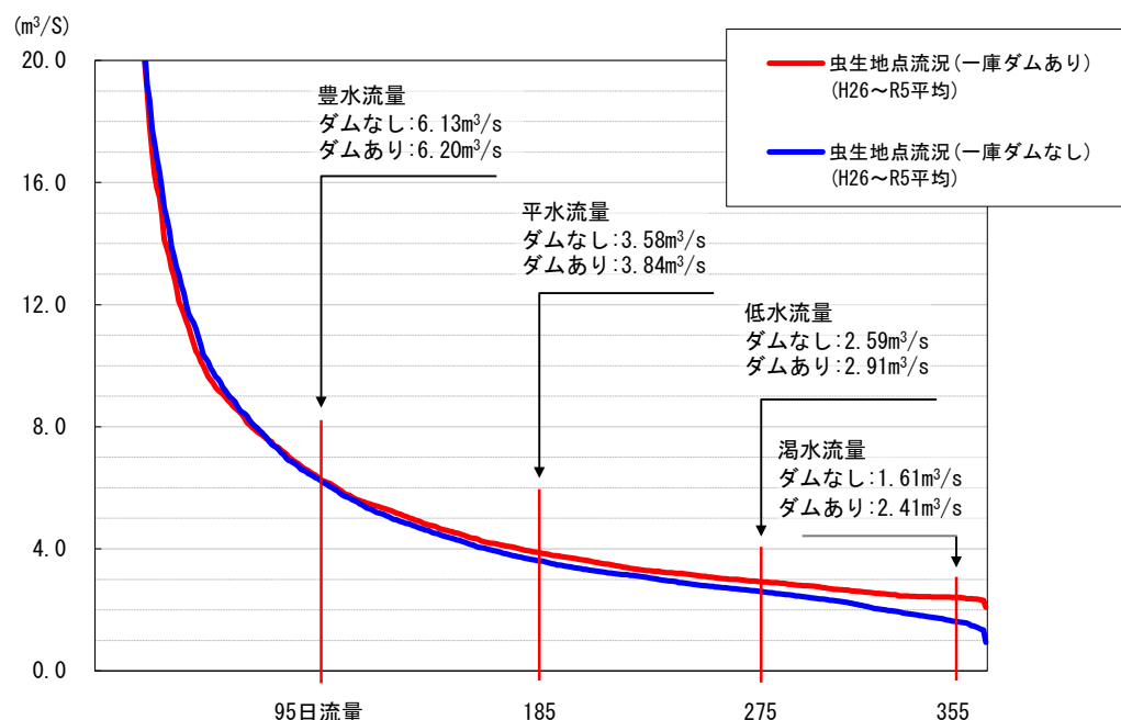
図 3.4-1 虫生地点流況のダムありなしの比較
