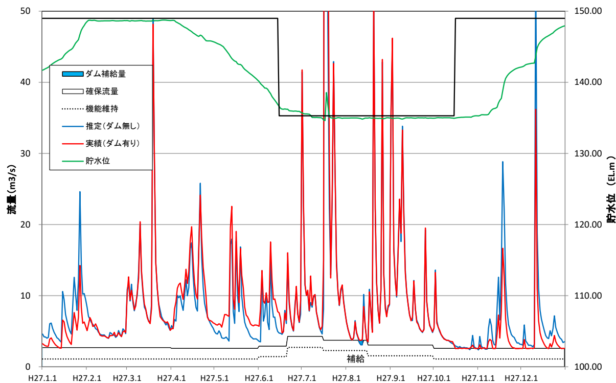
図 3.4-3(2) 虫生地点の確保流量と流量実績ほか(平成 27 年)
