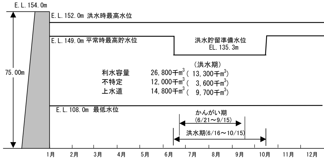
図 3.2-1 貯水池容量配分図
