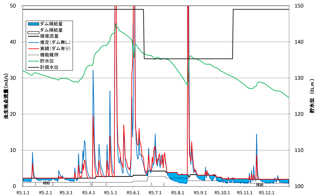
図 3.4-3(10) 虫生地点の確保流量と流量実績ほか(令和5年)
