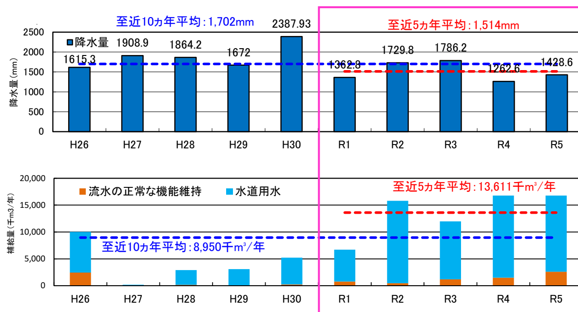
図 3.3-3 一庫ダムの利水補給実績
