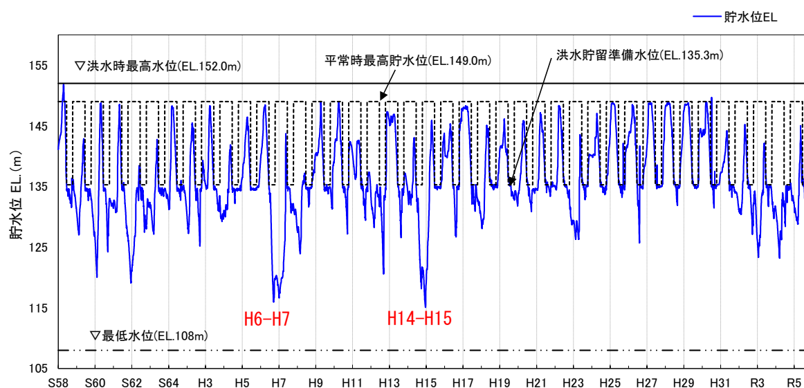
図 3.3-1 一庫ダム貯水池運用実績
