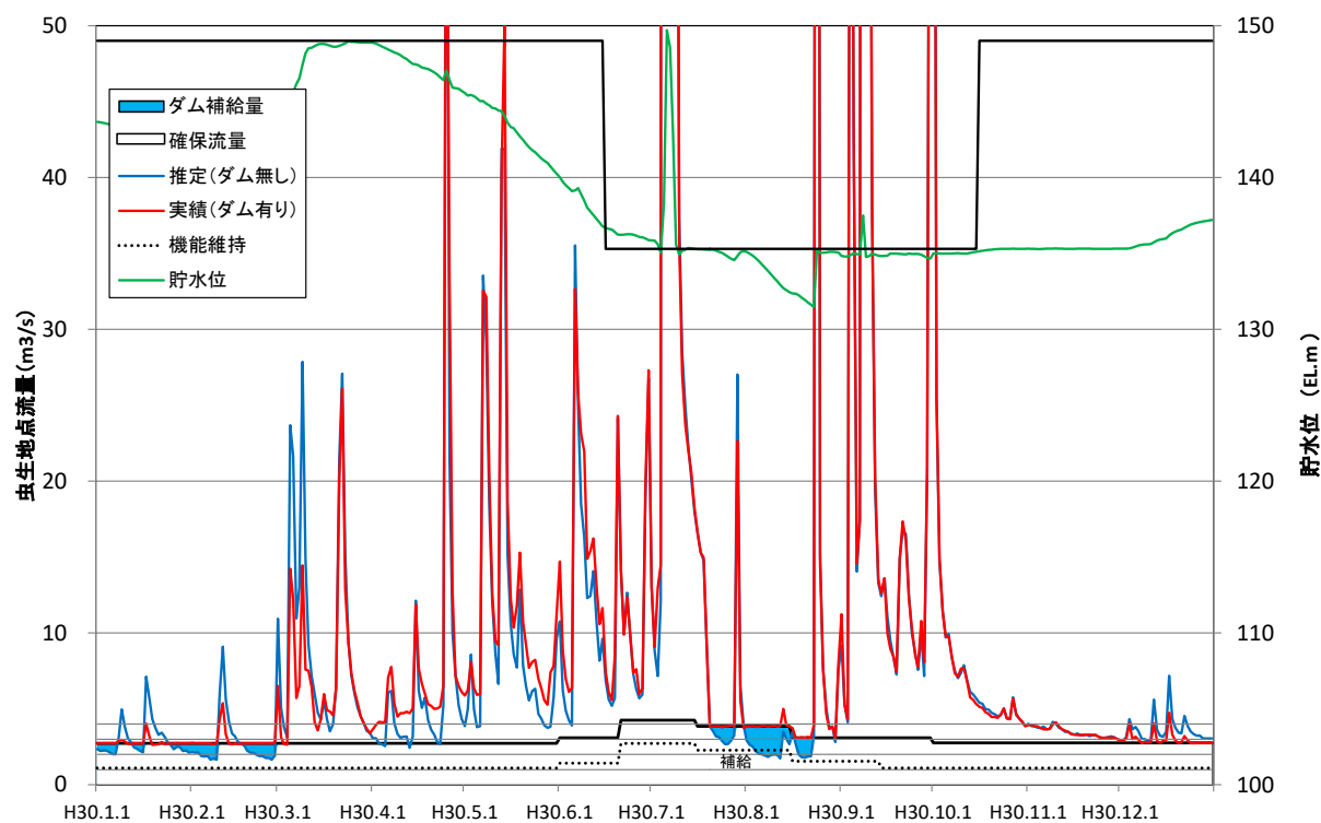
図 3.4-3(5) 虫生地点の確保流量と流量実績ほか(平成 30 年)
