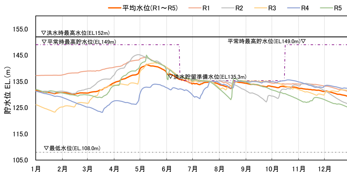
図 3.3-2 一庫ダム貯水池運用状況実績(至近 5 ヲ年 : R1-R5)
