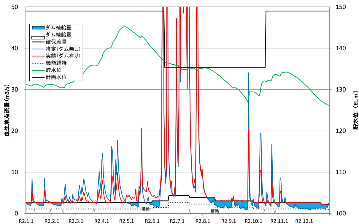
図 3.4-3(7) 虫生地点の確保流量と流量実績ほか(令和2年)
