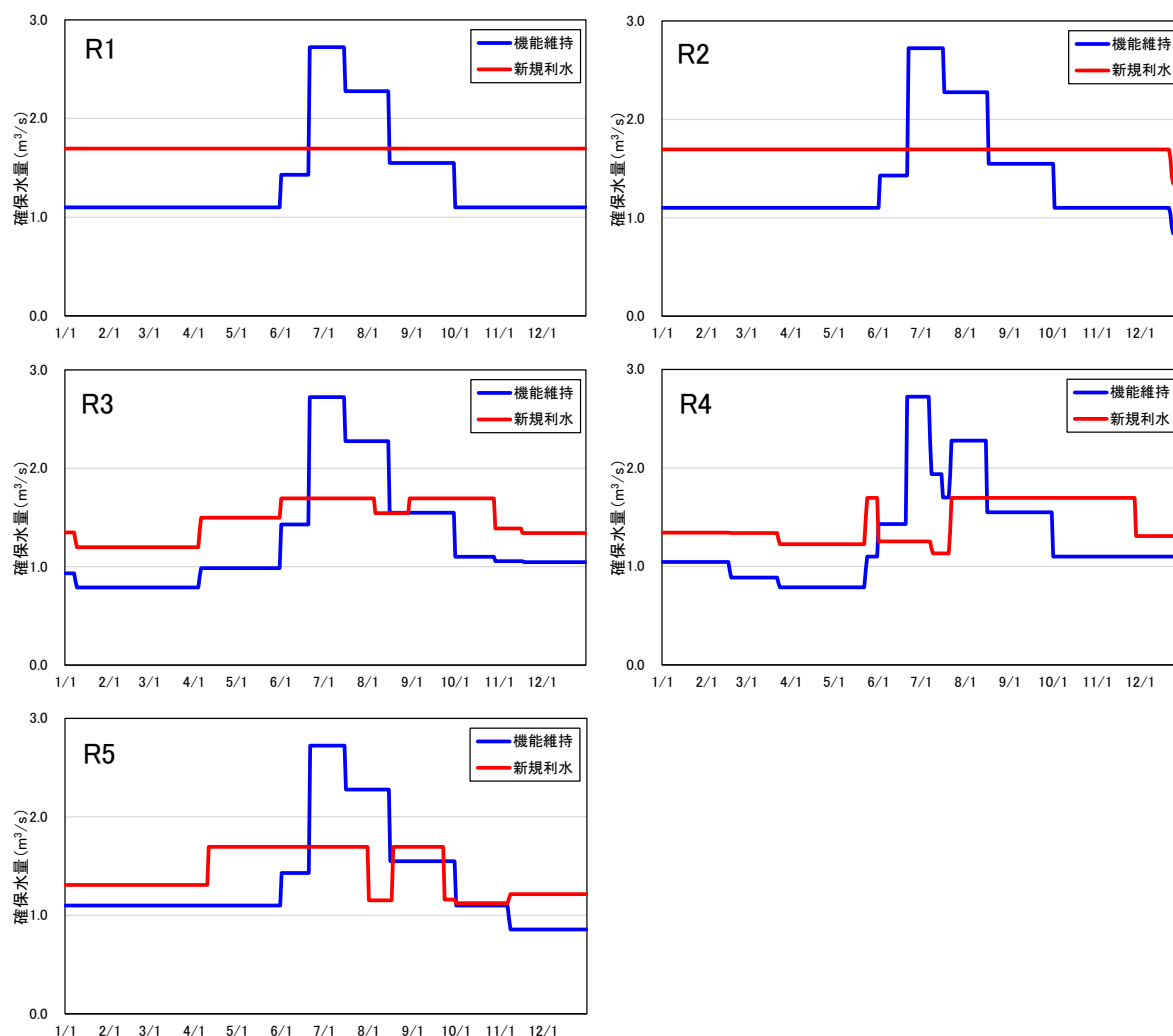
図 3.2-5 一庫ダム下流基準地点(虫生地点)における確保量
