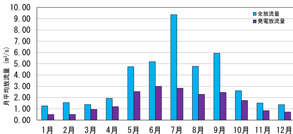
図 3.3-4 一庫ダムの発電実績
