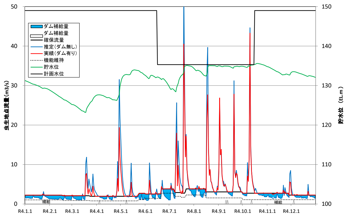
図 3.4-3(9) 虫生地点の確保流量と流量実績ほか(令和4年)
