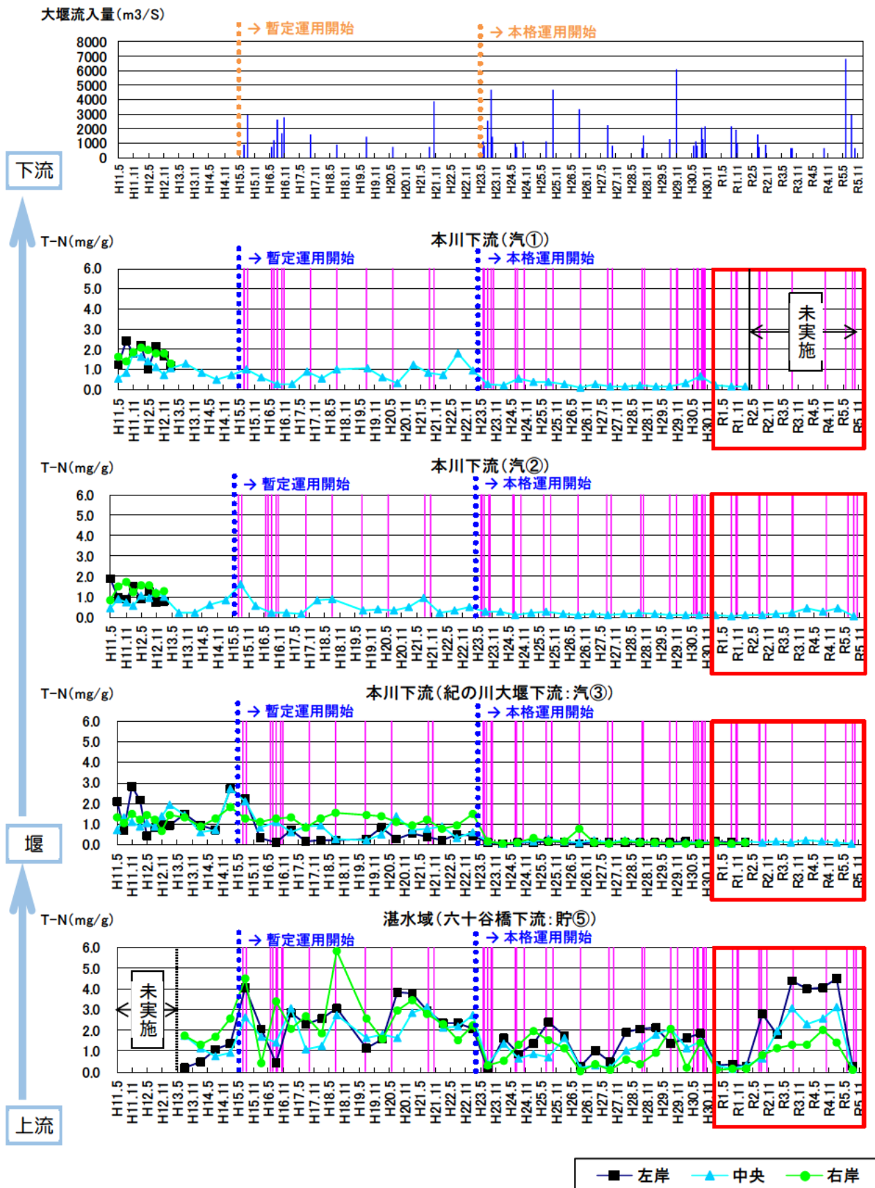
図 5.3-25 (9) 底質分析調査結果 下流～堰～上流 (T-N)
