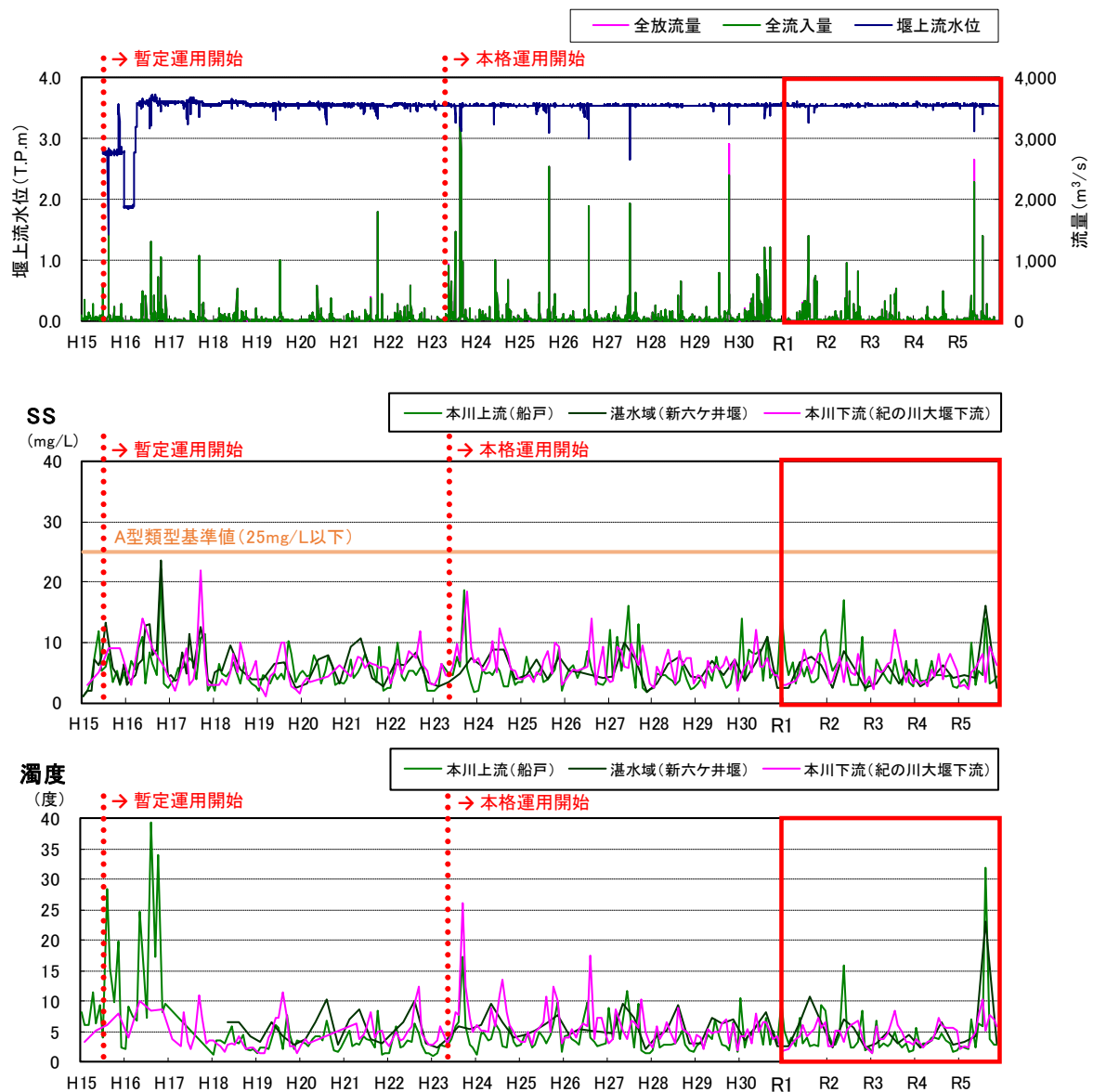
図 5.5-20 本川上流、湛水域、本川下流におけるSSと濁度の経年変化
