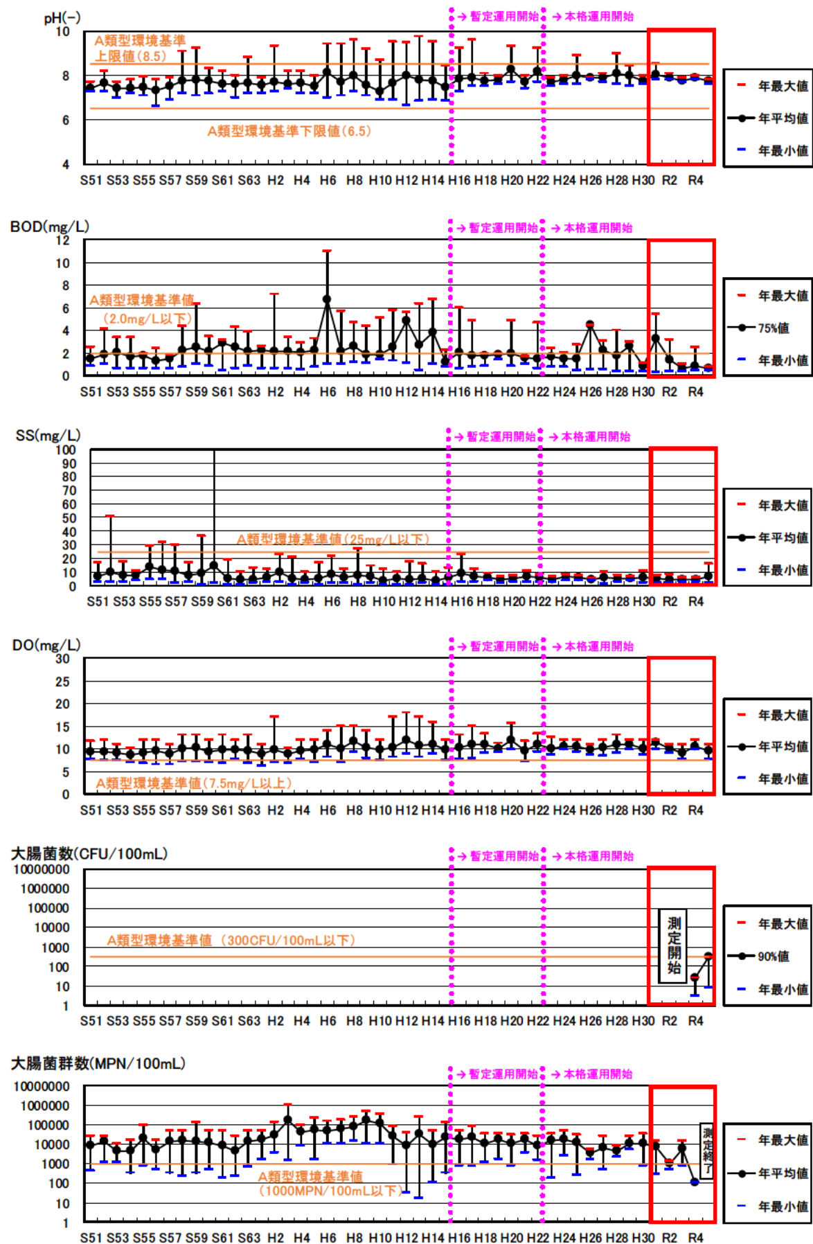
図 5.5-9 (3) 湛水域（新六ヶ井堰）地点における暫定運用開始前後の水質比較
