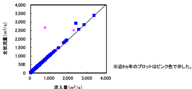
図 5.3-2 放流量・流入量の散布図 (H16～R5)
