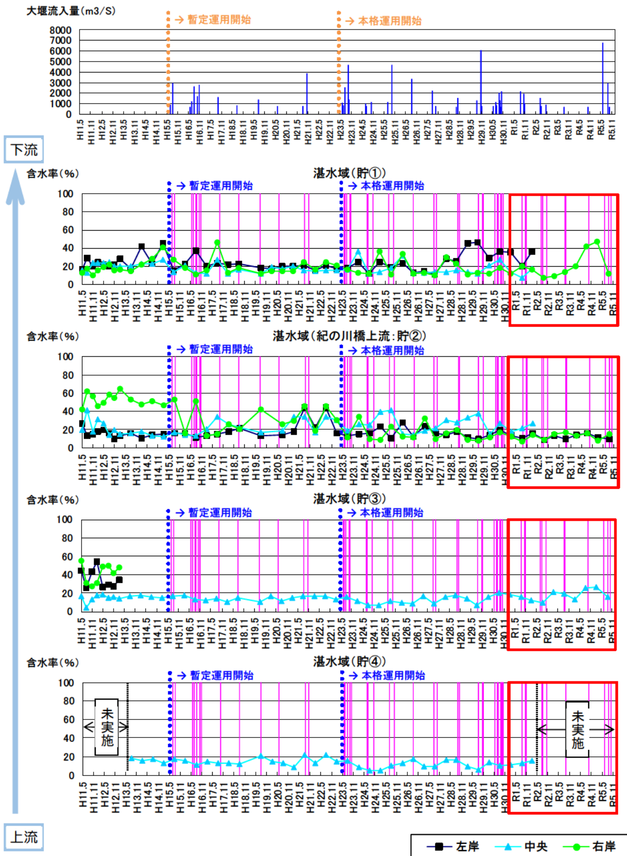
図 5.3-25 (2) 底質分析調査結果 堰～上流 (含水率)
