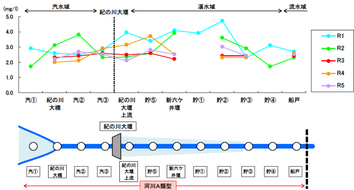
図 5.5-29 年平均CODの縦断変化
