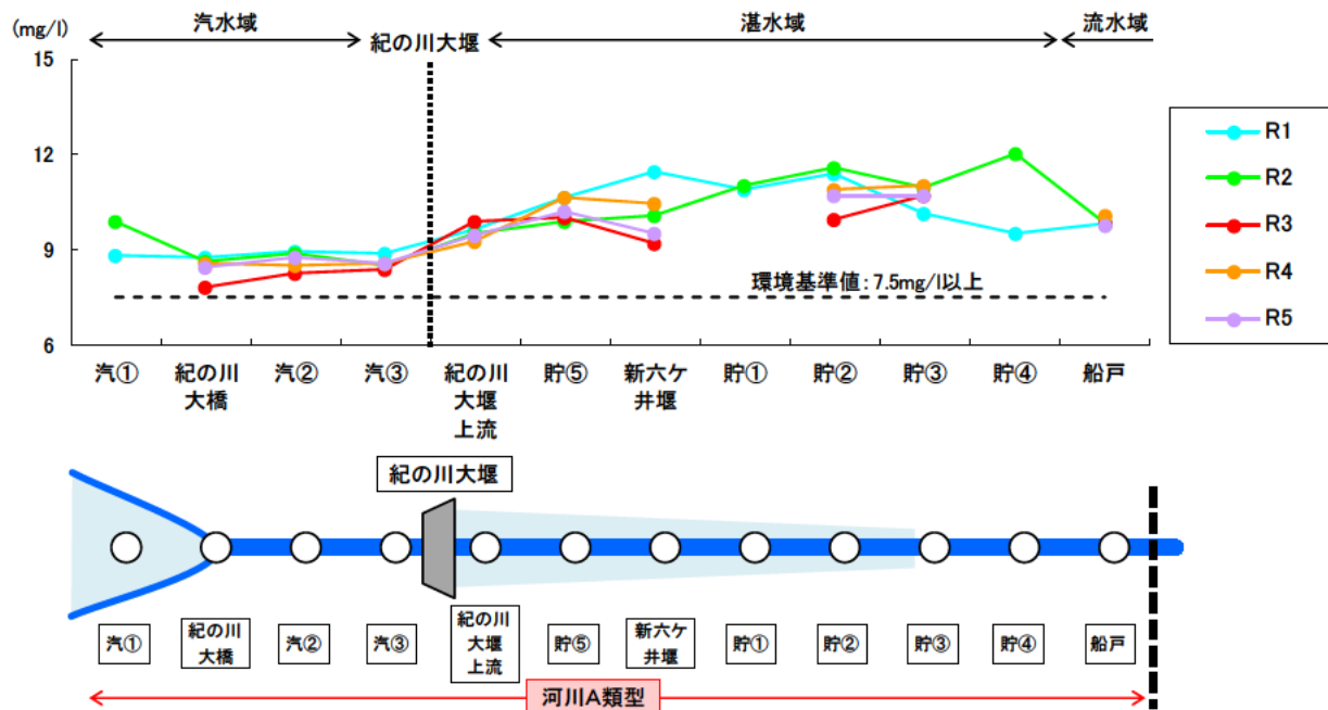
図 5.5-27 年平均D0の縦断変化
