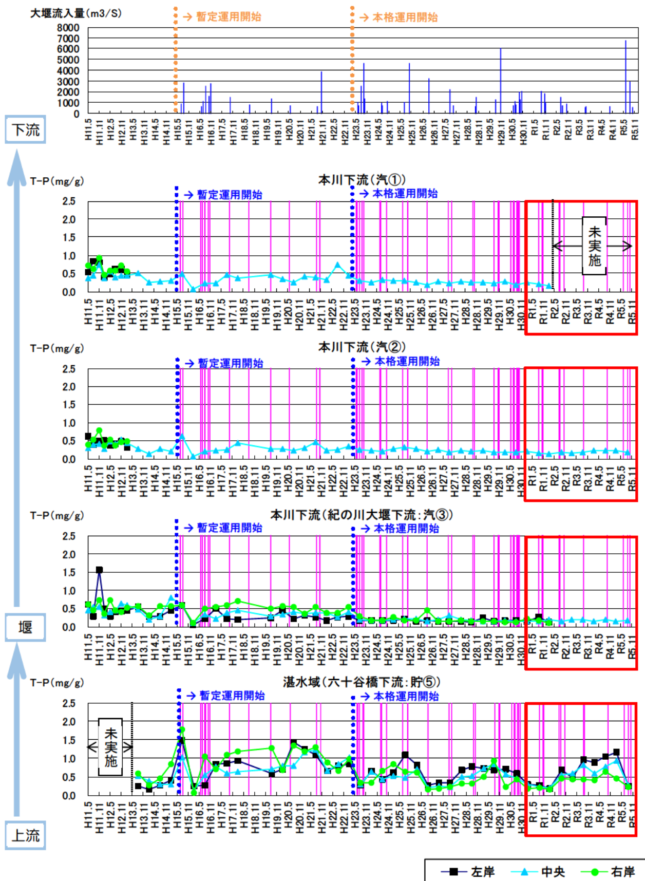
図 5.3-25 (11) 底質分析調査結果 下流～堰～上流 (T-P)
