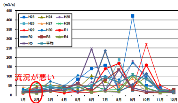
図5.5-35 紀の川大堰の月平均放流量（本格運用開始以降）
