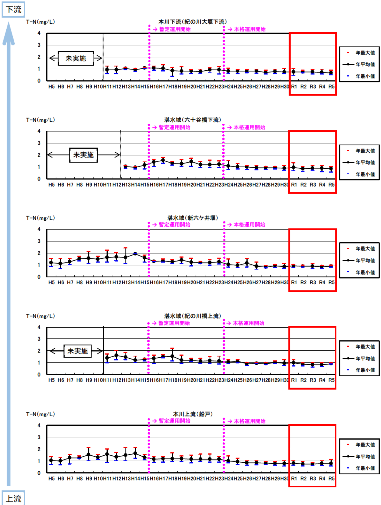
図 5.3-9 (10) 調査地点ごとの T-N 年平均値の経年変化
