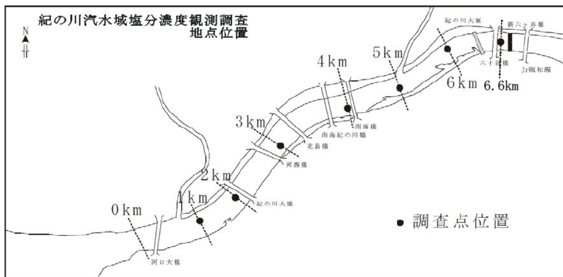
図 5.3-16 紀の川汽水域塩分濃度調査実施地点 (H14、H15、H19)
