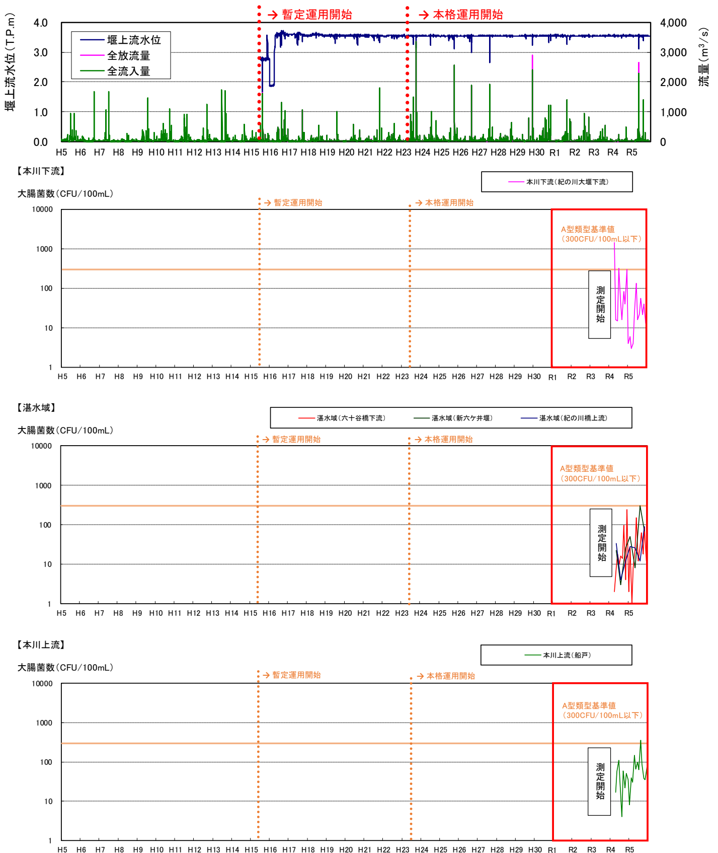
図 5.3-11 (7) 調査地点ごとの大腸菌数の経月変化 (H5～R5)
