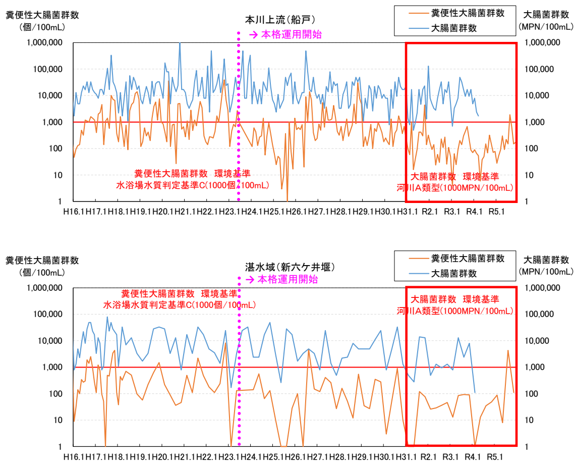
図 5.5-8 大腸菌群数及び糞便性大腸菌群数の推移
