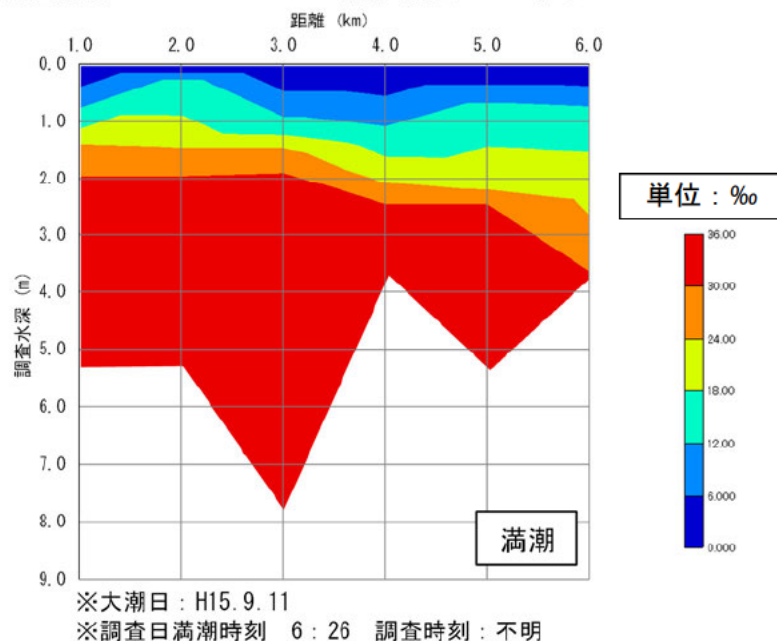
図 5.3-17 (1) 堰運用前後での塩分縦断変化の比較（大潮－満潮）（改変）
