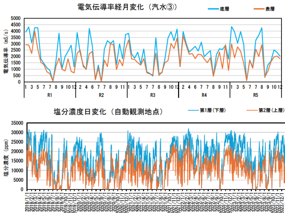
図 5.3-19 紀の川大堰下流汽水域電気伝導率（上図）及び塩分濃度（下図）の変化 (H31 (R1) ~R5)
