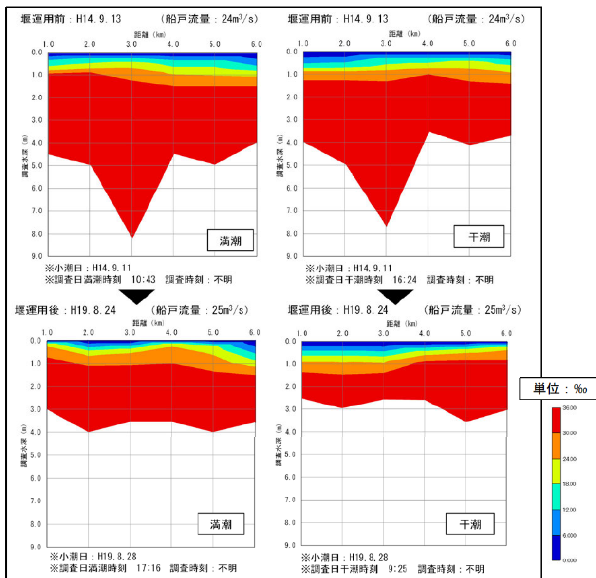
図 5.5-16 大堰運用前後（小潮）の塩分濃度
