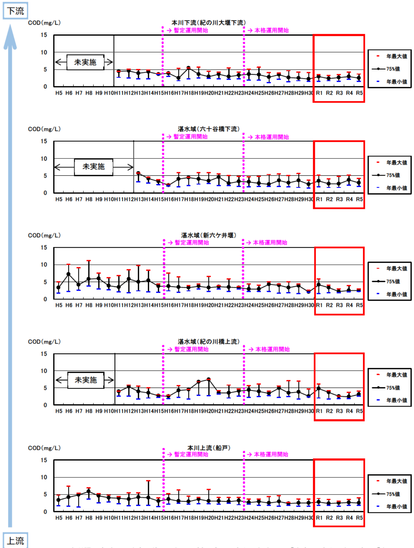
図 5.3-9 (4) 調査地点ごとの COD75%値の経年変化
