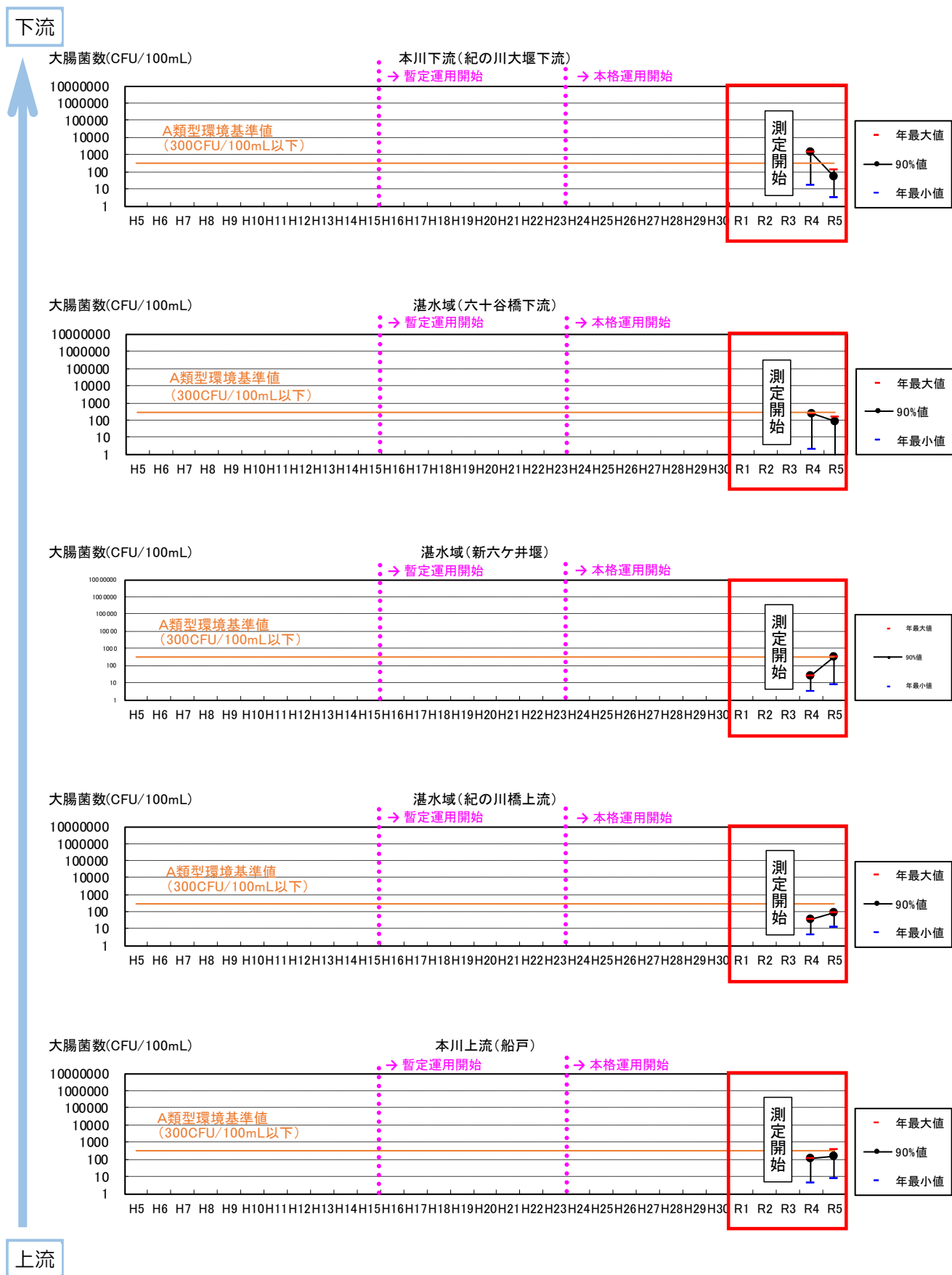
図 5.3-9 (7) 調査地点ごとの大腸菌数 90%値の経年変化
