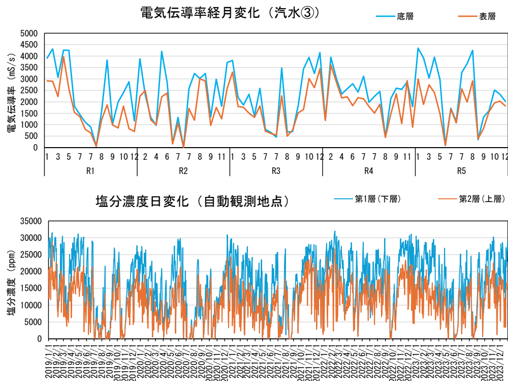
図 5.5-15 紀の川大堰下流における電気伝導率と塩分濃度の変化
