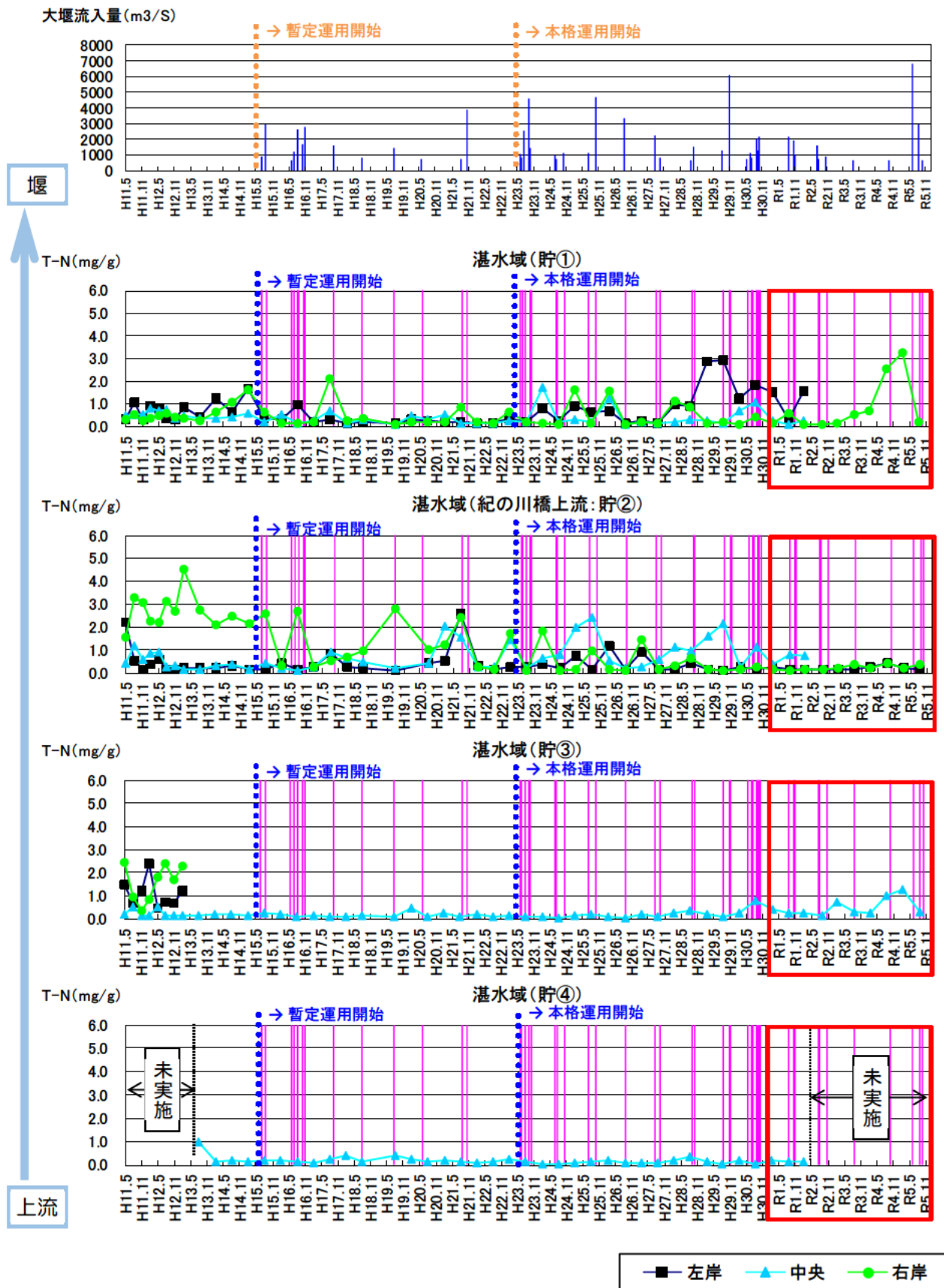
図 5.3-25 (10) 底質分析調査結果 堰～上流 (T-N)
