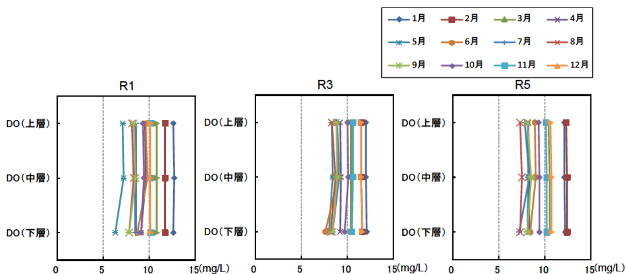
図 5.5-10 (2) 紀の川大堰直上地点の DO の鉛直分布
