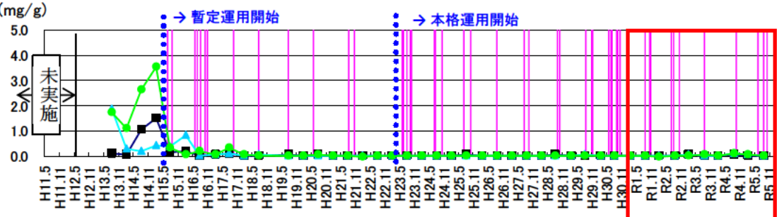
T-S(mg/g)
