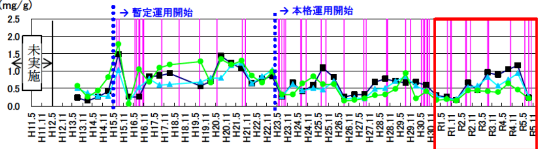
T-S(mg/g)
