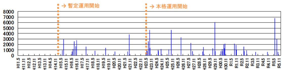
T-N(mg/g)
