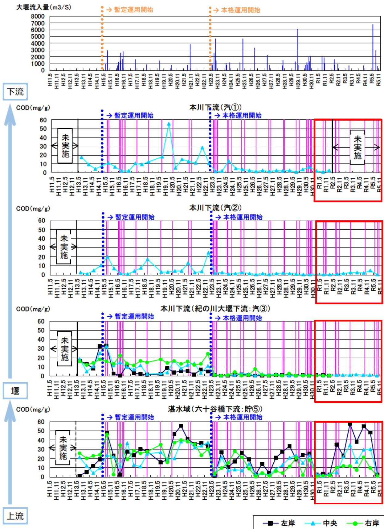
図 5.3-25 (5) 底質分析調査結果 下流～堰～上流 (COD)
