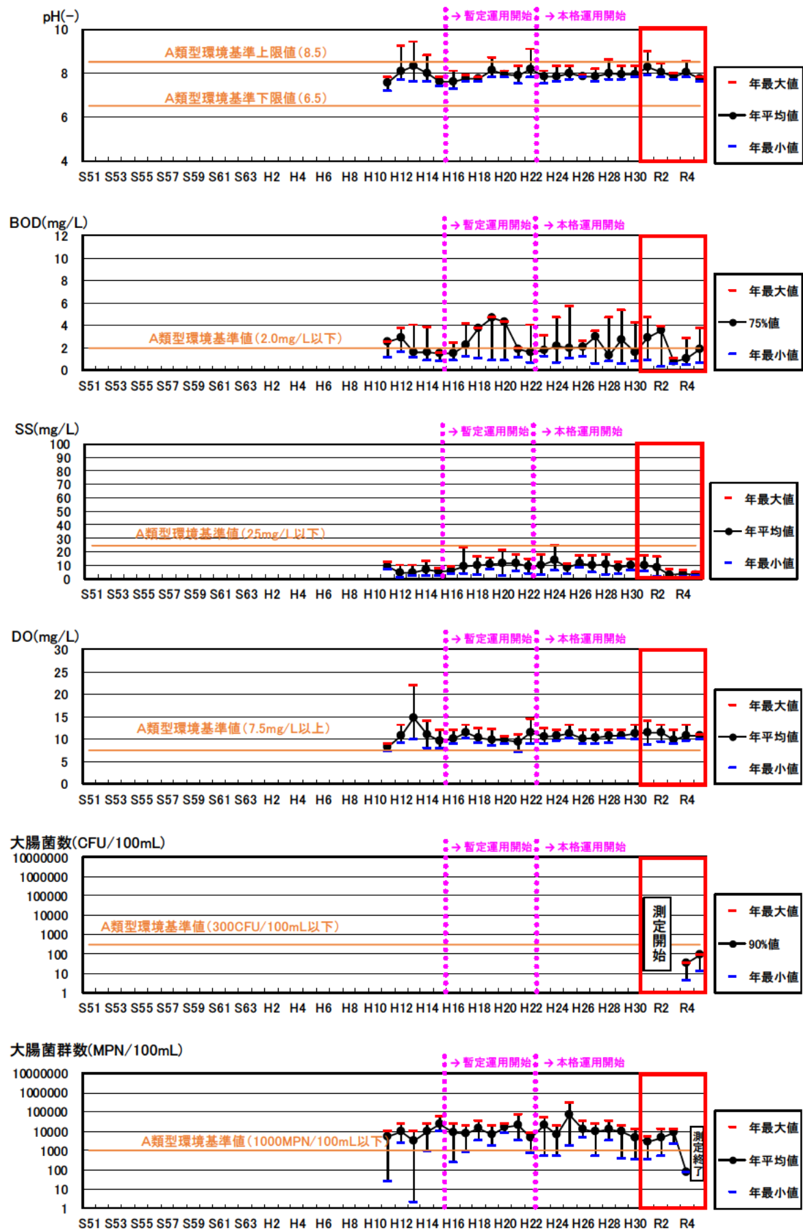
図 5.5-9 (4) 湛水域（紀の川橋上流）地点における暫定運用開始前後の水質比較
