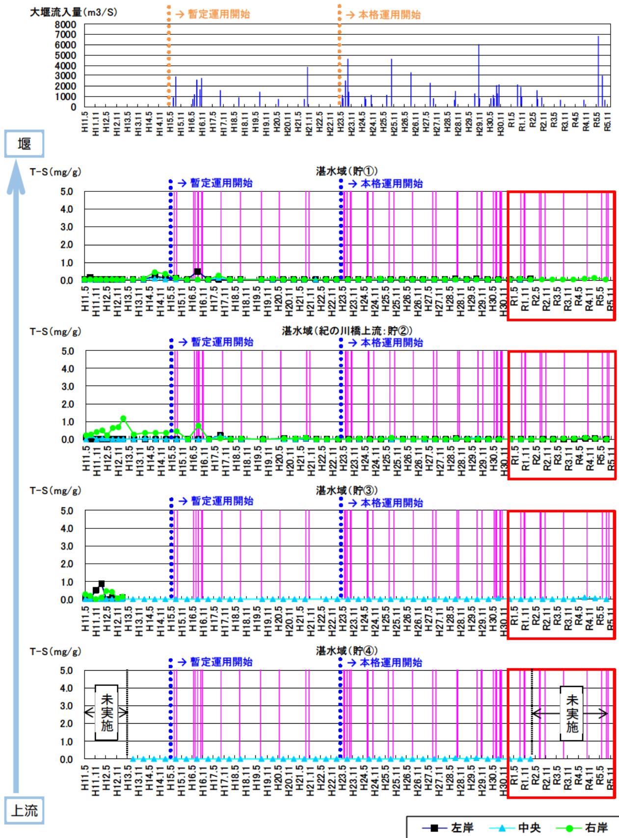
図 5.3-25 (14) 底質分析調査結果 堰～上流 (T-S)
