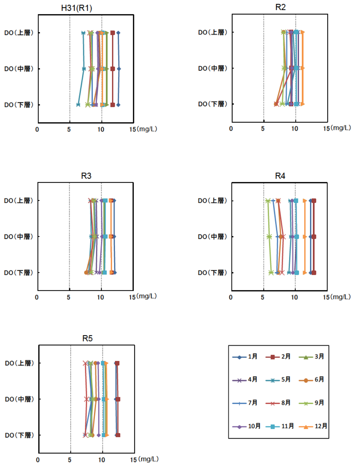
図 5.3-12 (2) 紀の川大堰直上地点の DO の鉛直分布
