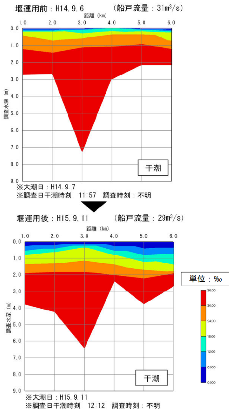
図 5.3-17 (2) 堰運用前後での塩分縦断変化の比較（大潮－干潮）（改変）
