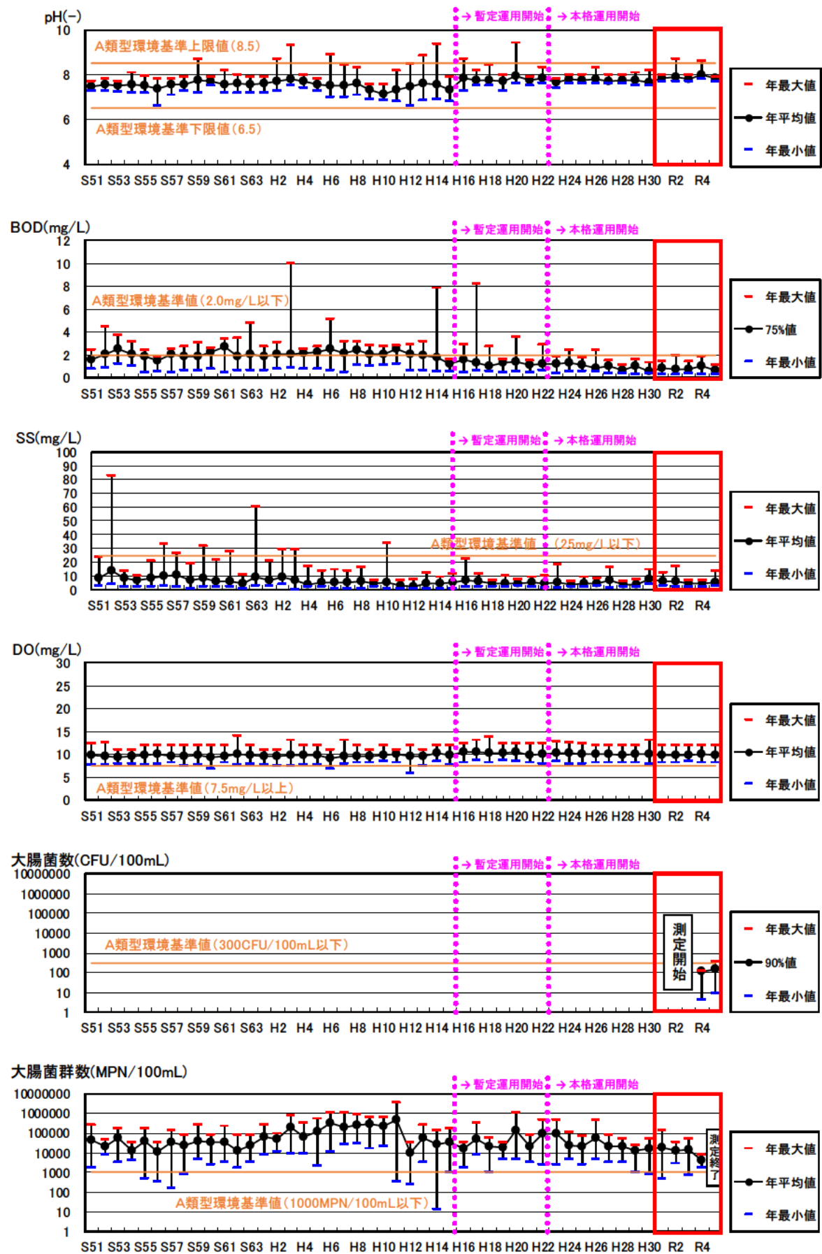
図 5.5-9 (5) 本川上流（船戸）地点における暫定運用開始前後の水質比較
