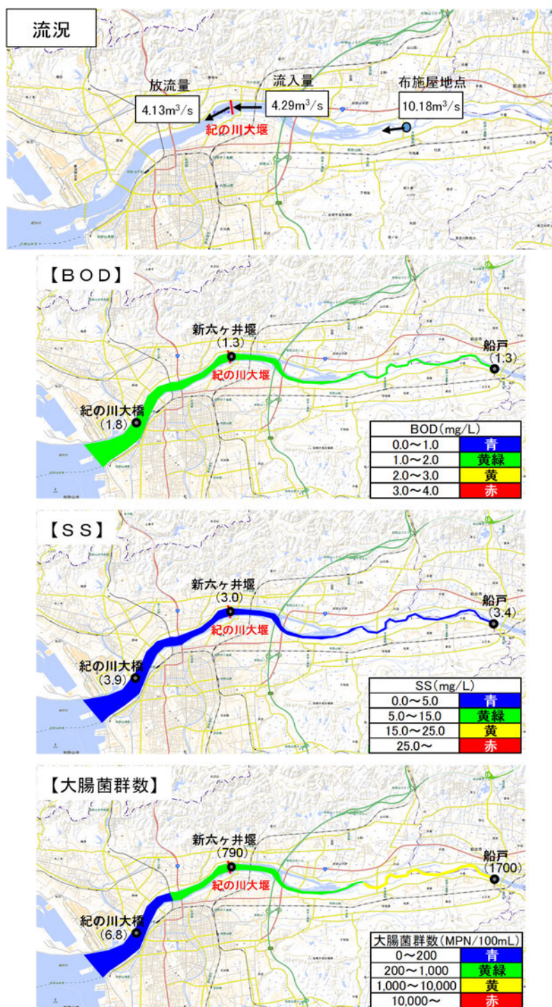
図 5.5-34 流況が悪い月の水質縦断変化図（平成16年1月）
