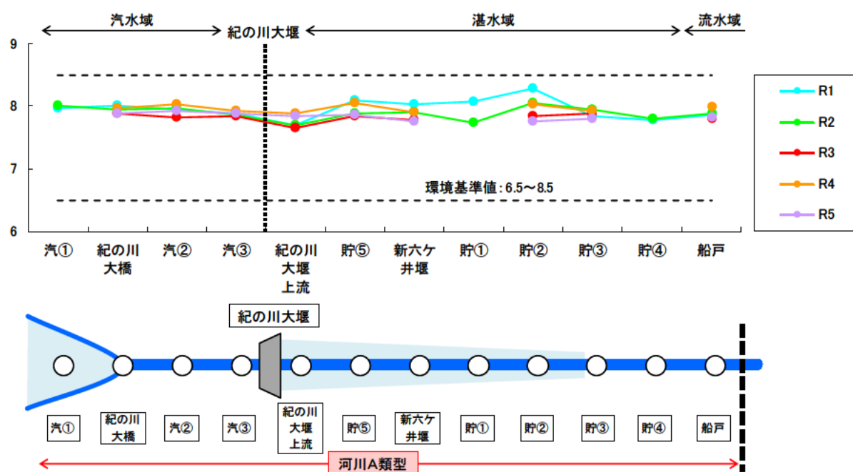
図 5.5-26 年平均pHの縦断変化
