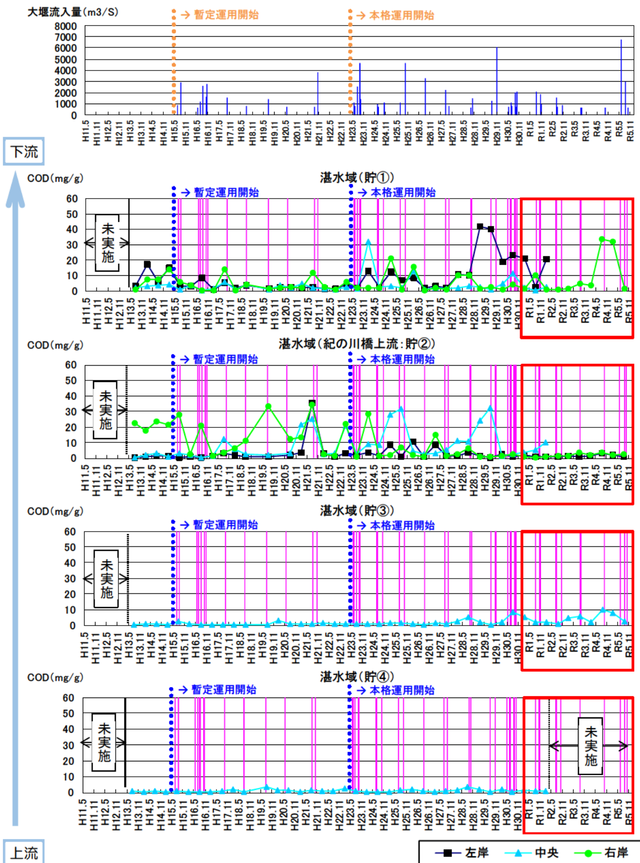
図 5.3-25 (6) 底質分析調査結果 堰～上流 (COD)
