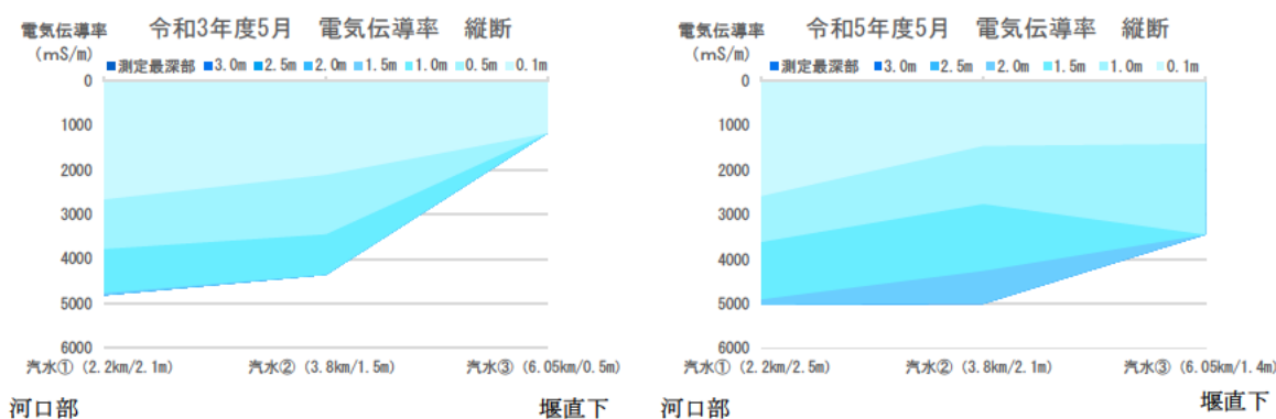
図 5.5-19 電気伝導率の縦断・垂直分布（抜粋）
