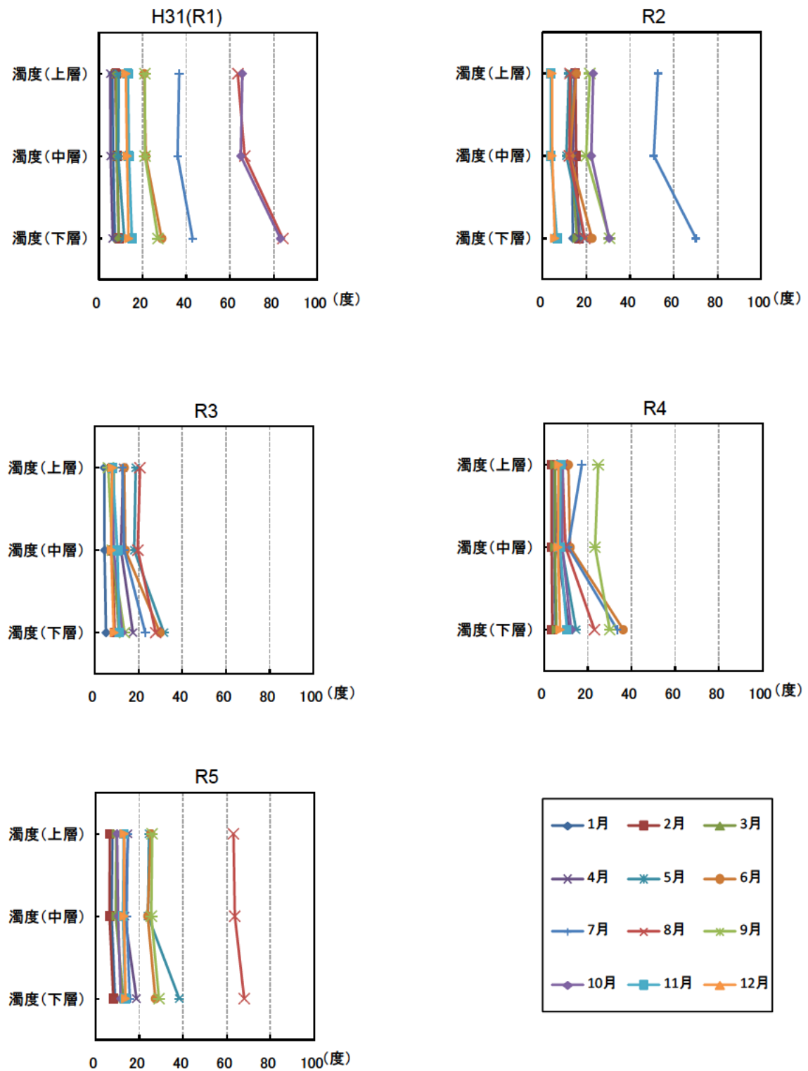
図 5.3-12 (3) 紀の川大堰直上地点の濁度の鉛直分布
