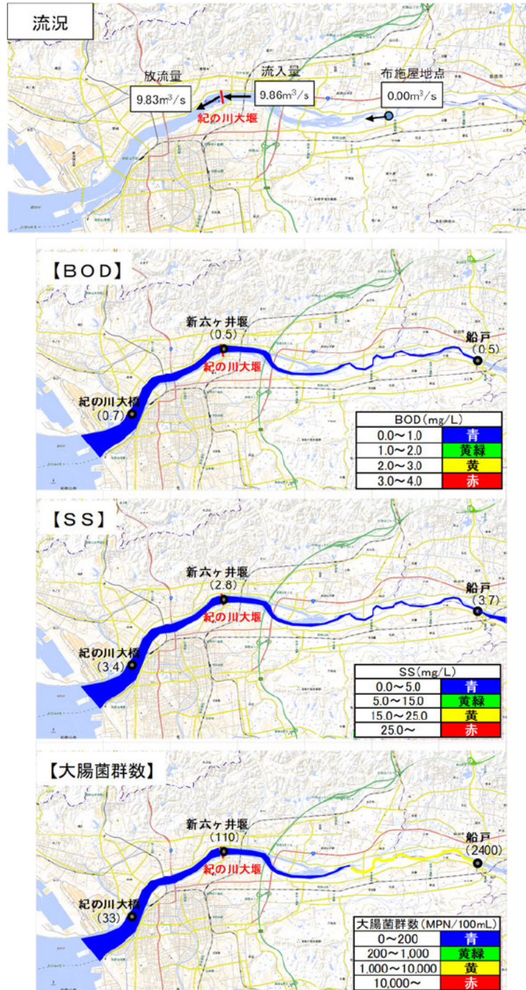
図 5.5-36 流況が悪い月の水質縦断変化図（令和4年2月）
