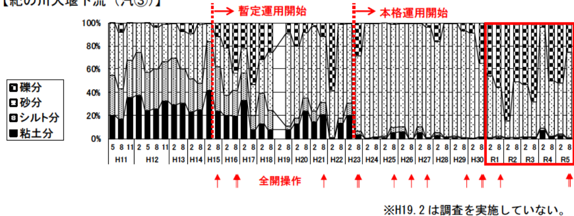
図 5.5-23 底質粒度組成の経年変化
