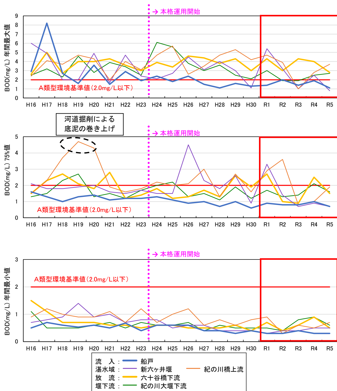
図 5.5-2 BODの経年変化
