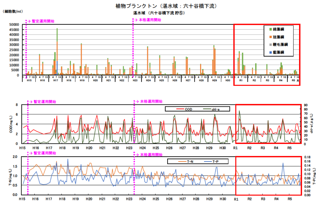
図 5.5-22 湛水域（六十谷橋下流）の植物プランクトン細胞数の推移（H15～R5）
