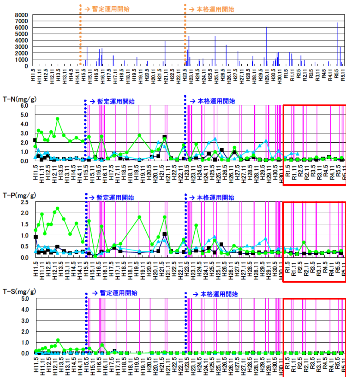
図 5.5-24 (1) 底質濃度の経年変化（紀の川橋上流）
