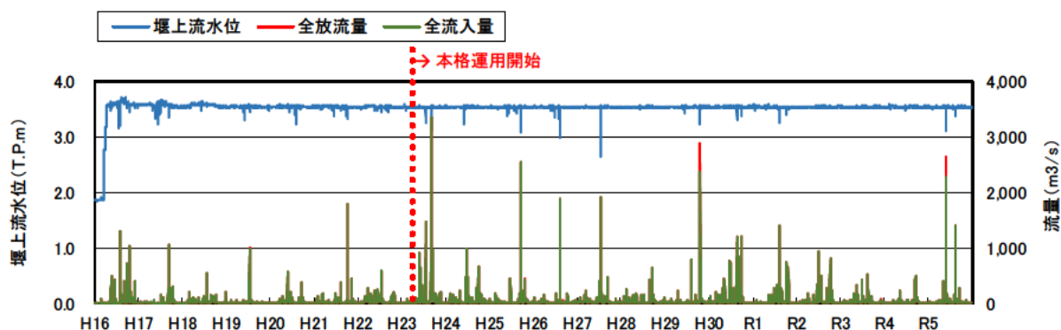
図 5.3-1 紀の川大堰諸量 (H16～R5)
