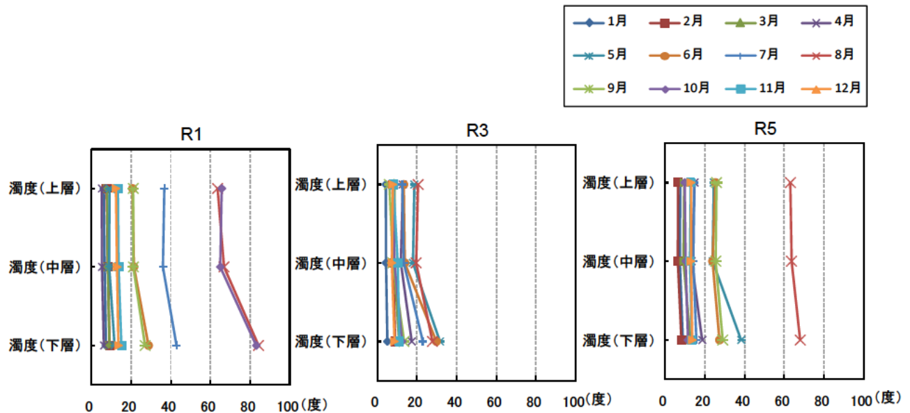
図 5.5-10 (3) 紀の川大堰直上地点の濁度の鉛直分布
