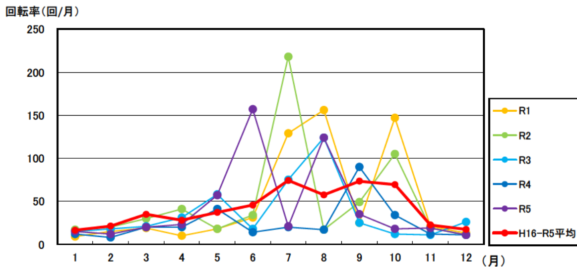
図 5.3-6 月回転率の経月変化
