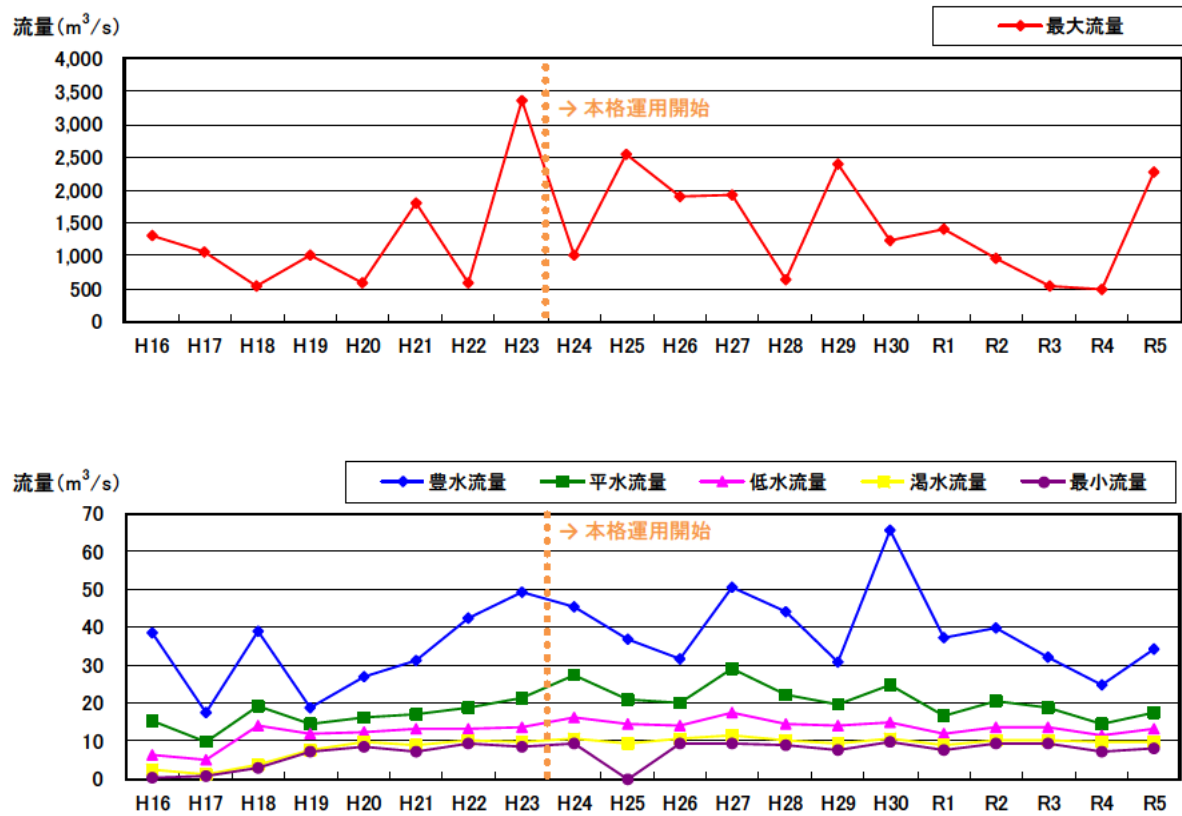
図 5.3-4 紀の川大堰の流入量の推移図
