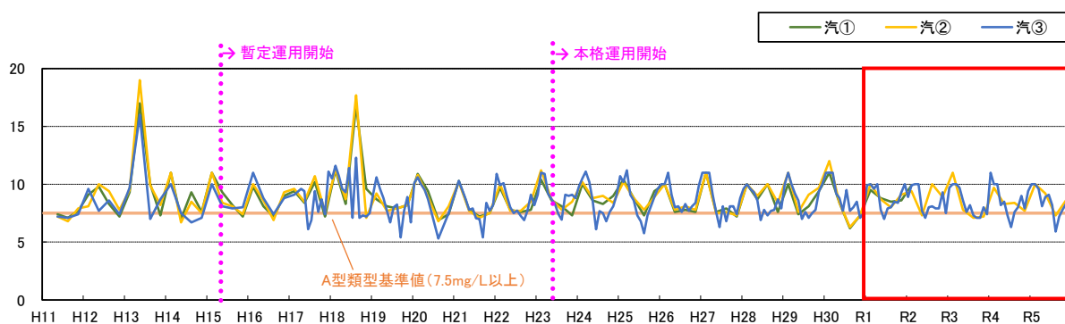
図 5.3-13 紀の川大堰下流の D0 の推移
