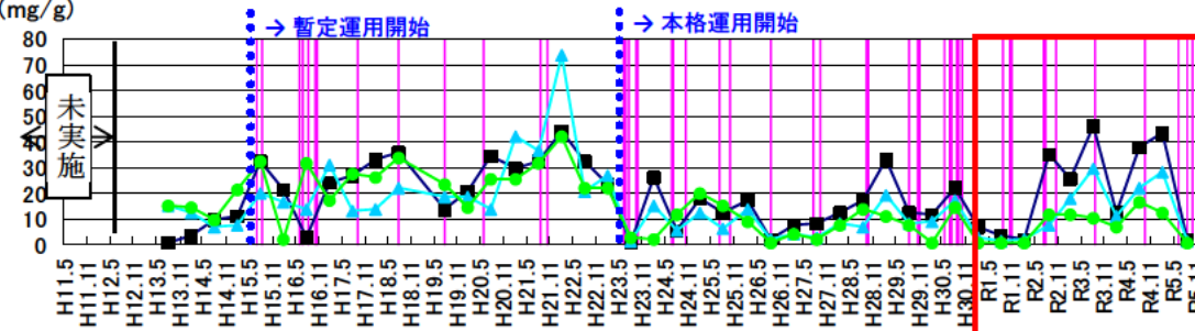
図 5.5-24 (4) 底質濃度の経年変化(六十谷橋下流)
