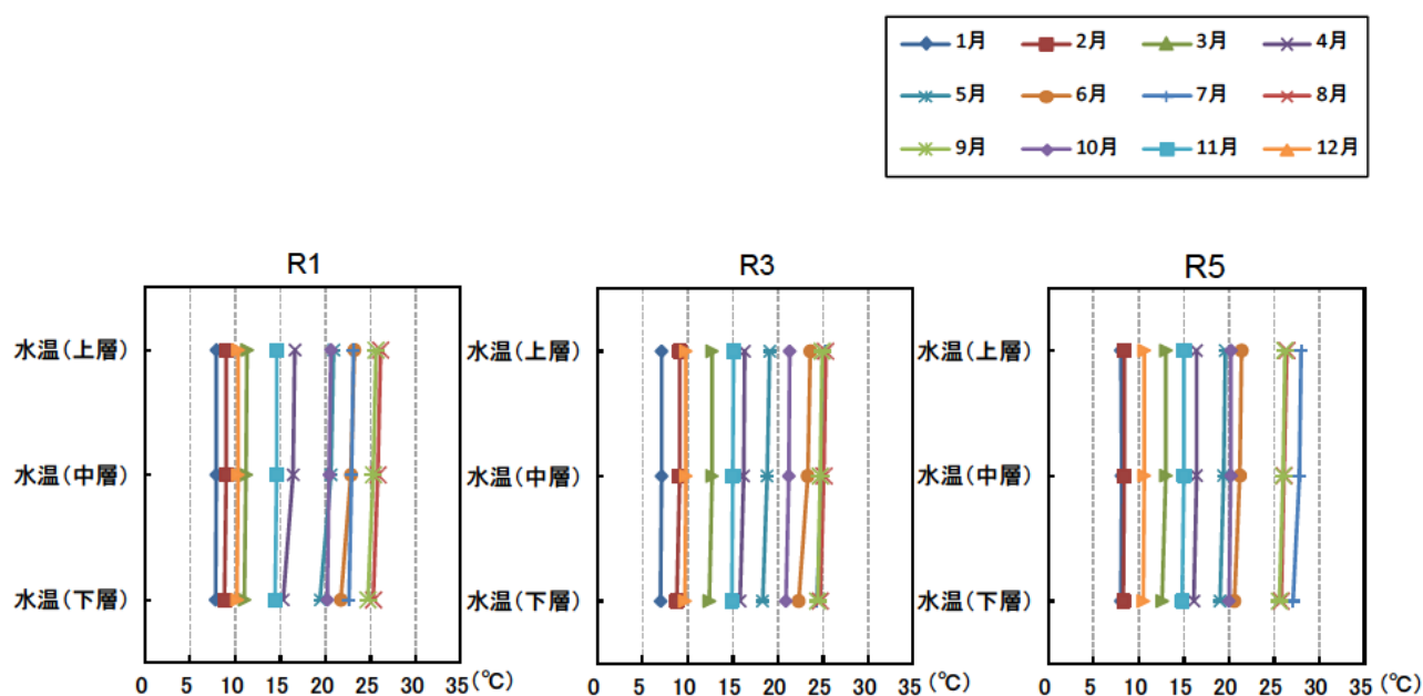
図 5.5-10 (1) 紀の川大堰直上地点の水温の鉛直分布
