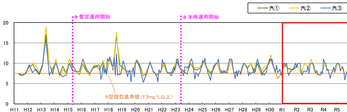
図 5.5-12 紀の川大堰下流のD0の推移
