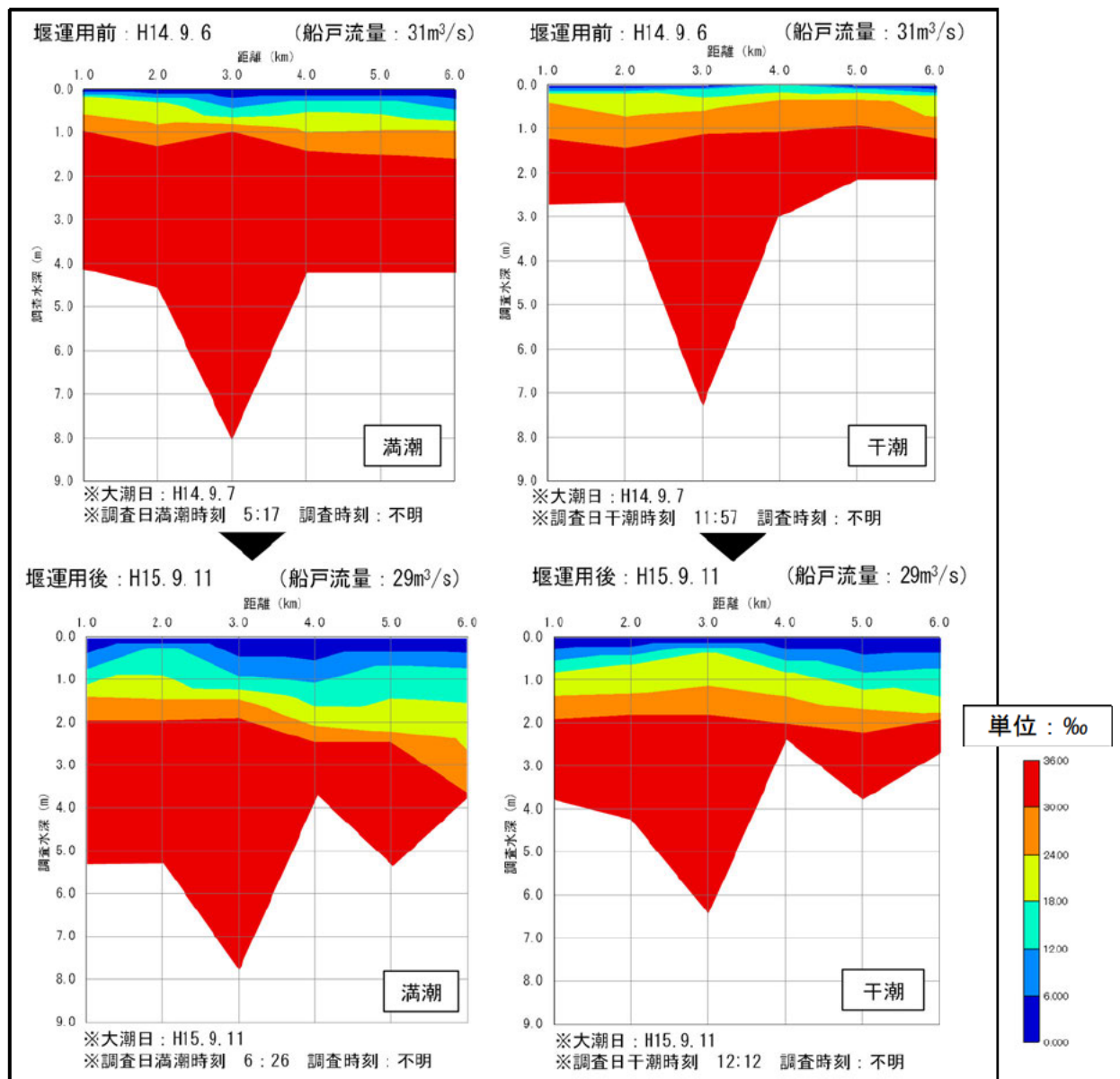
図 5.5-17 大堰運用前後（大潮）の塩分濃度
