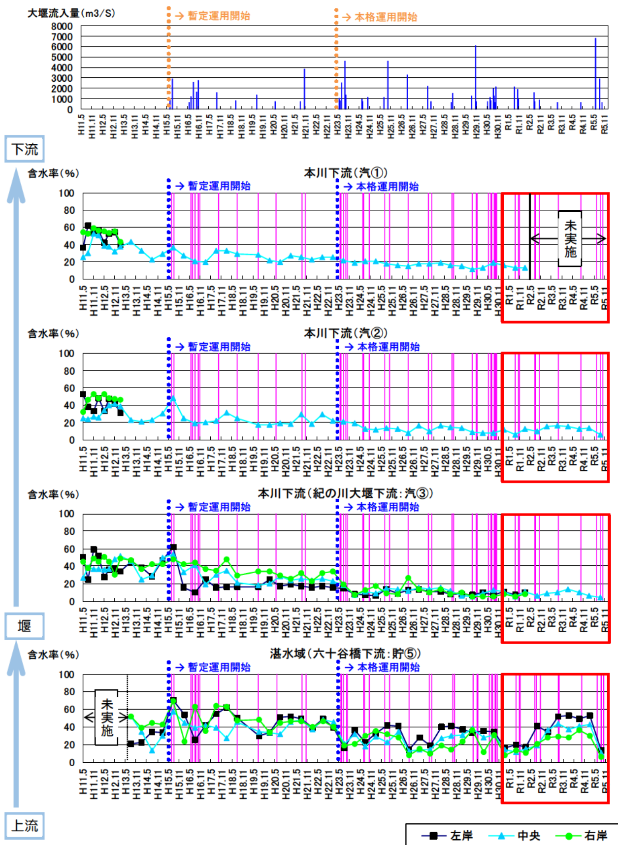
図 5.3-25 (1) 底質分析調査結果 下流～堰～上流 (含水率)
