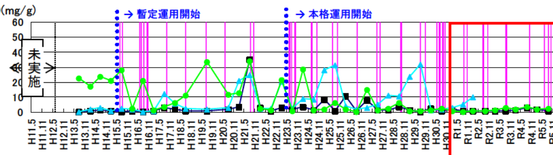
TOC(mg/g)
