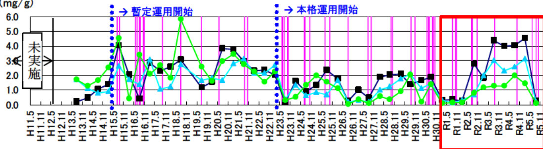
T-P(mg/g)
