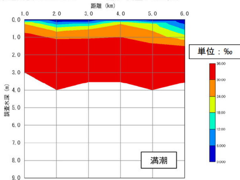
図 5.3-17 (3) 堰運用前後での塩分縦断変化の比較（小潮－満潮）（改変）
