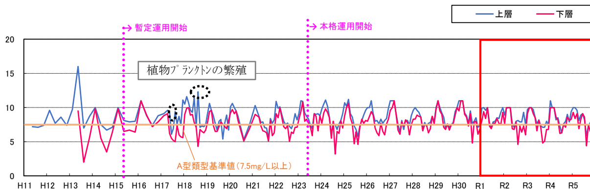
図 5.5-13 大堰直下流(汽③)のD0の鉛直分布
