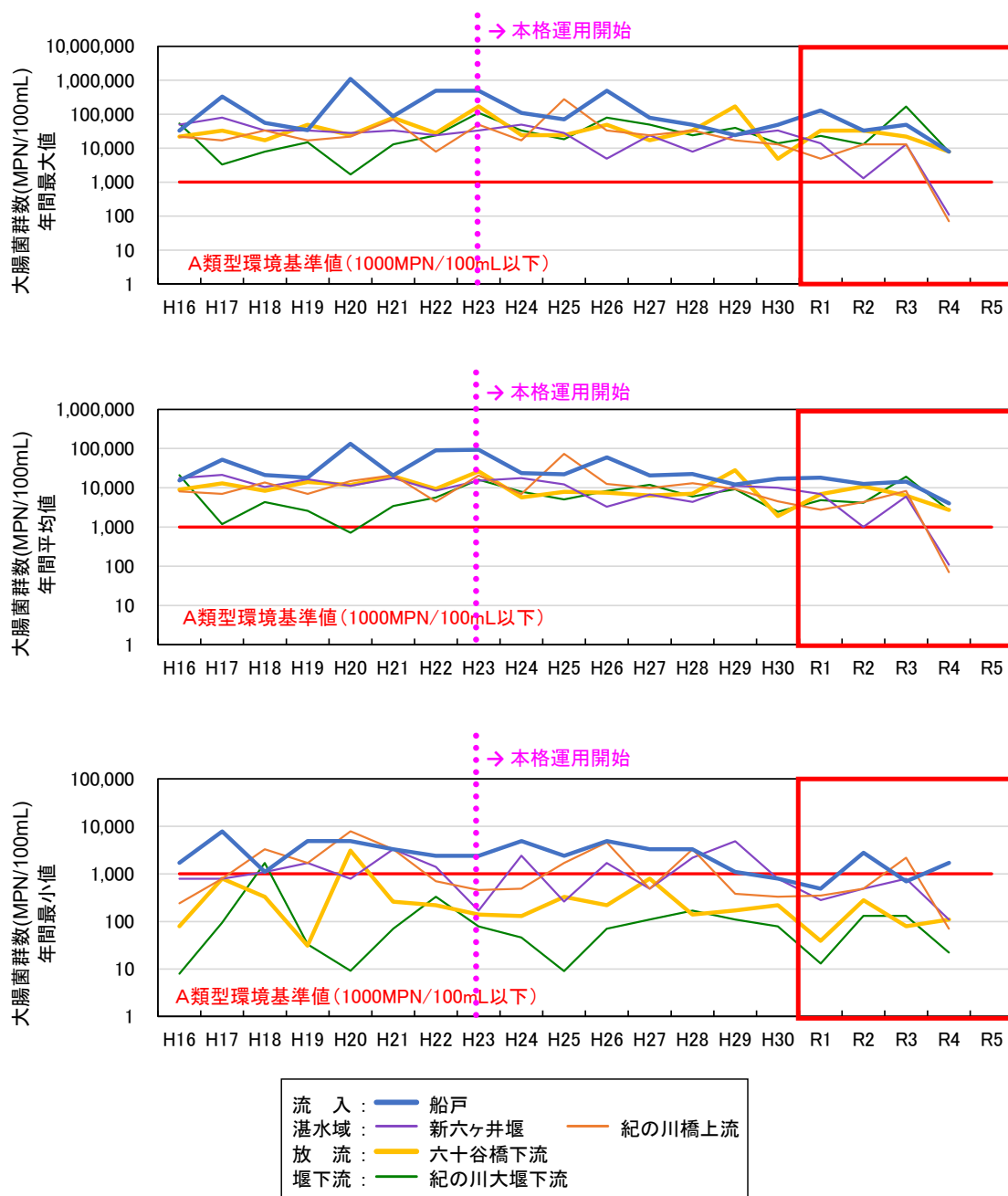
図 5.5-7 大腸菌群数の経年変化
