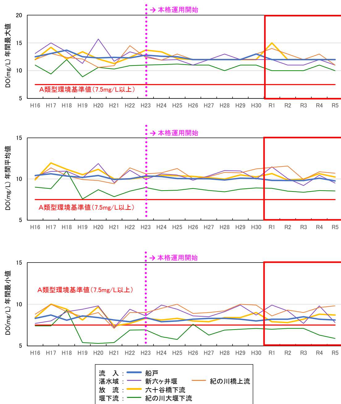
図 5.5-5 D0の経年変化
