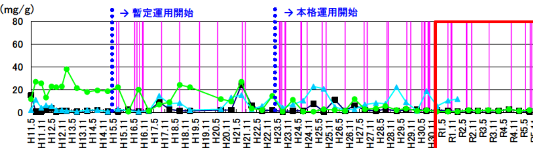
図 5.5-24 (2) 底質濃度の経年変化 (紀の川橋上流)
