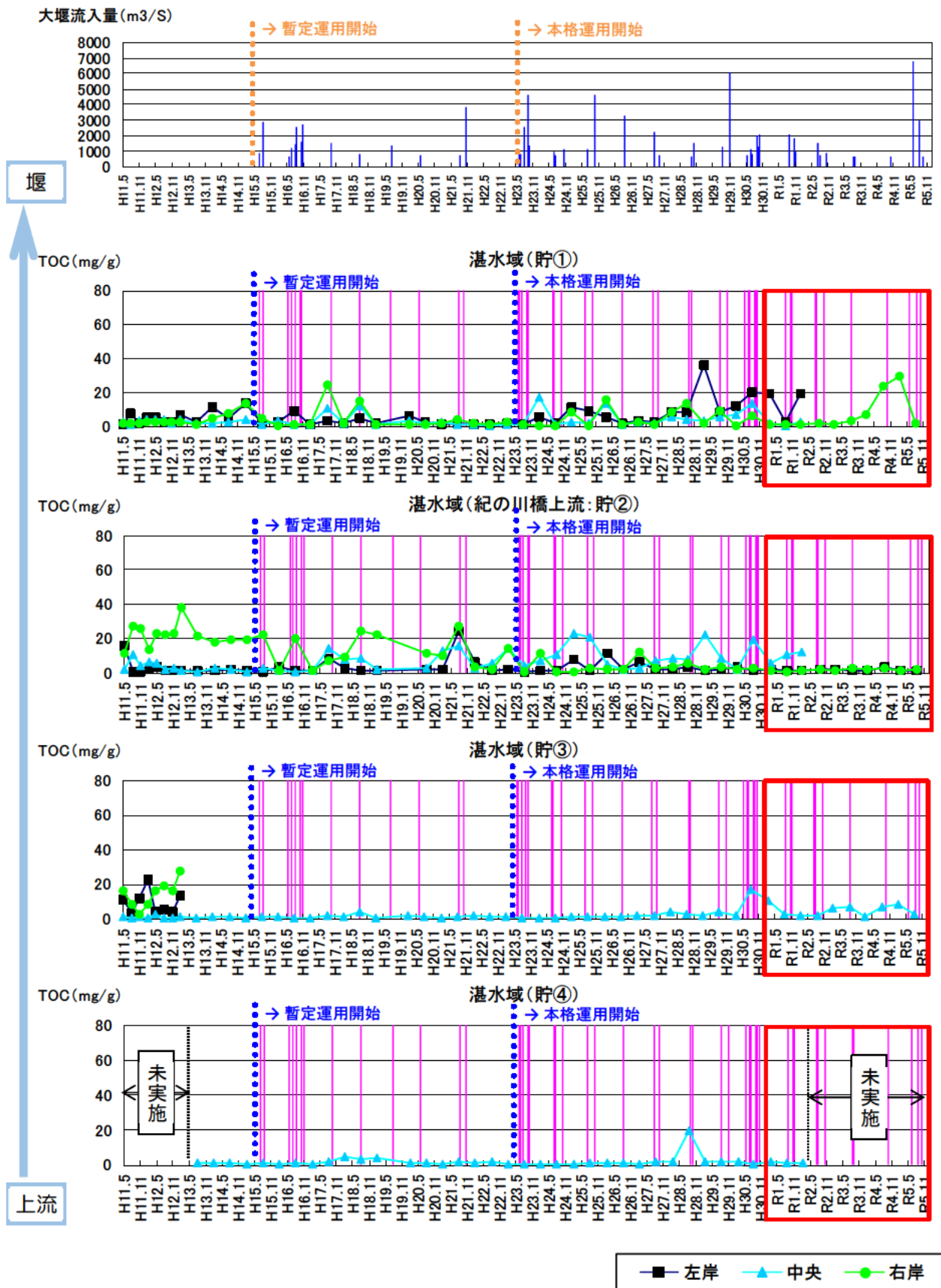
図 5.3-25 (8) 底質分析調査結果 堰～上流 (TOC)
