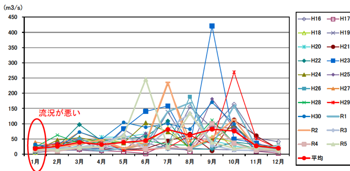
図 5.5-33 月平均放流量 (H16~R5)
