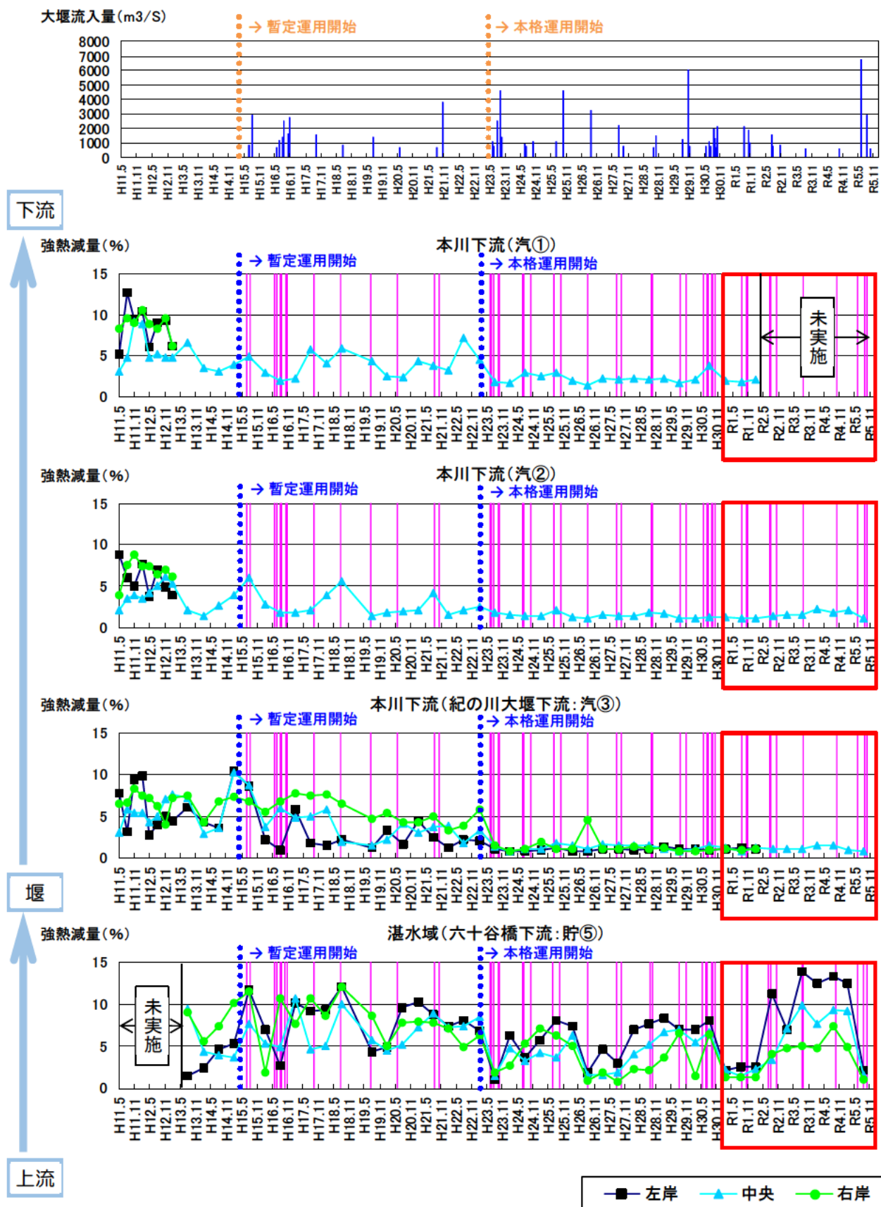
図 5.3-25 (3) 底質分析調査結果 下流～堰～上流(強熱減量)
