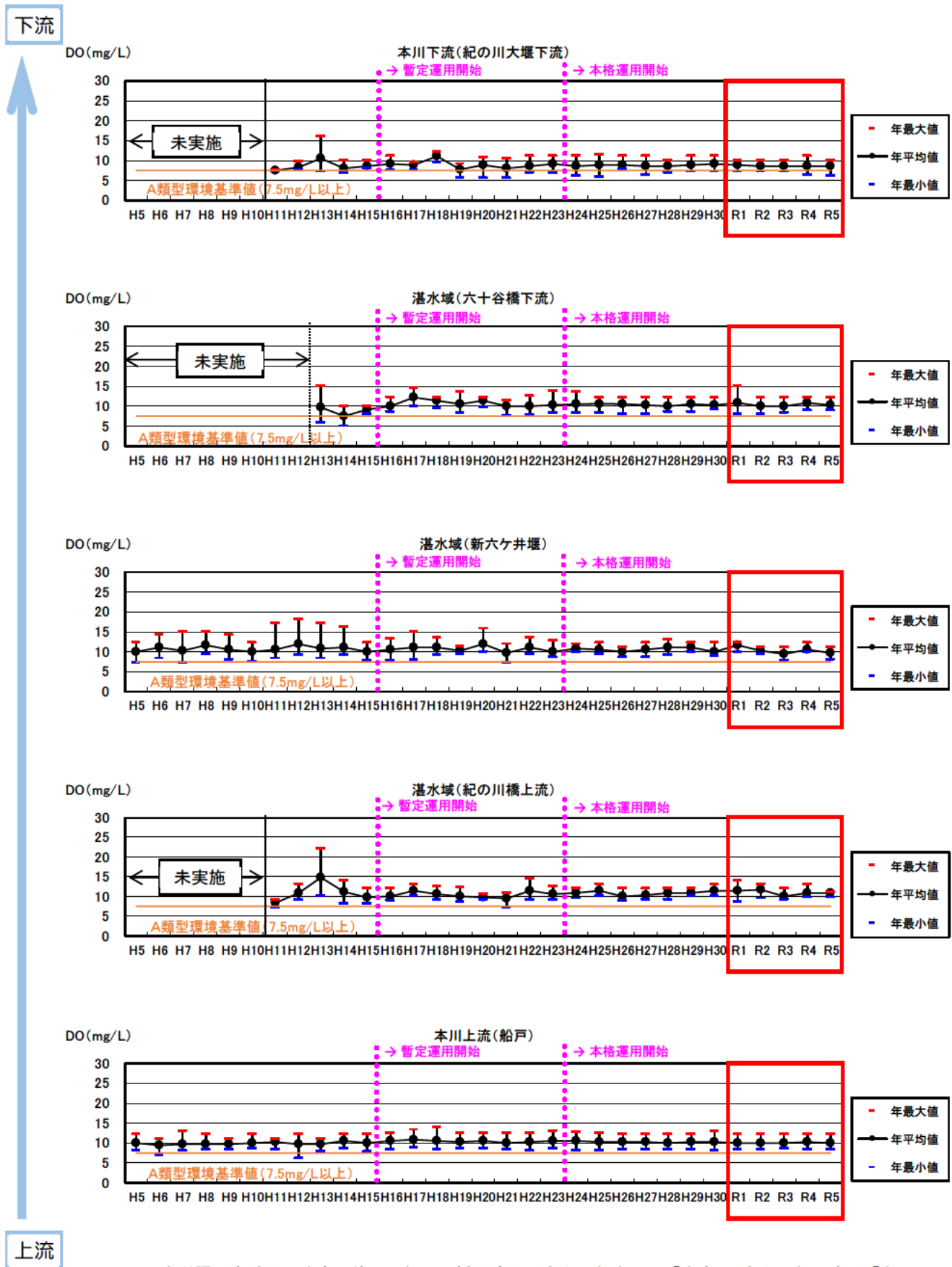
図 5.3-9 (6) 調査地点ごとの DO 年平均値の経年変化
