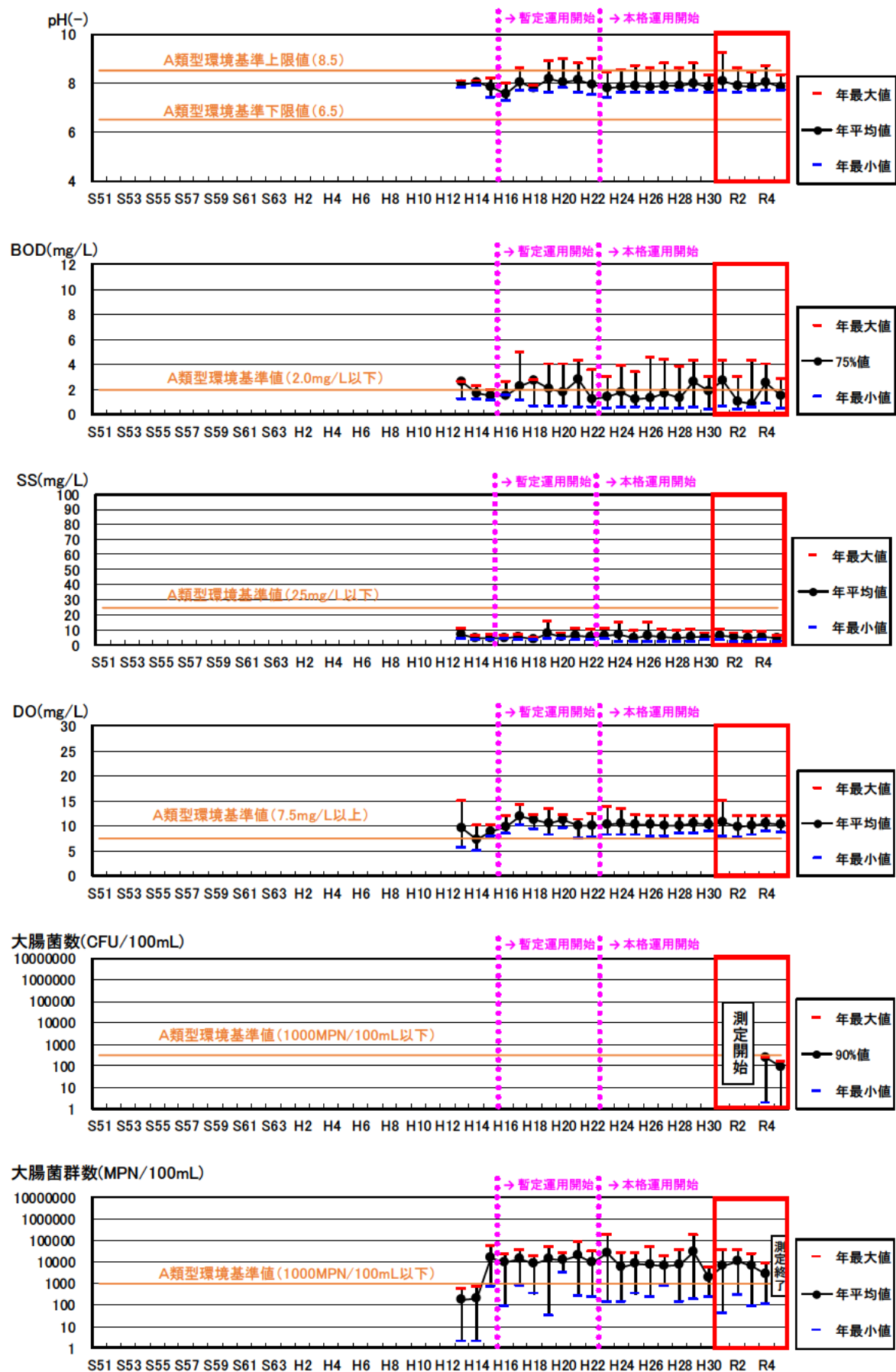
図 5.5-9 (2) 湛水域(六十谷橋下流)地点における暫定運用開始前後の水質比較
