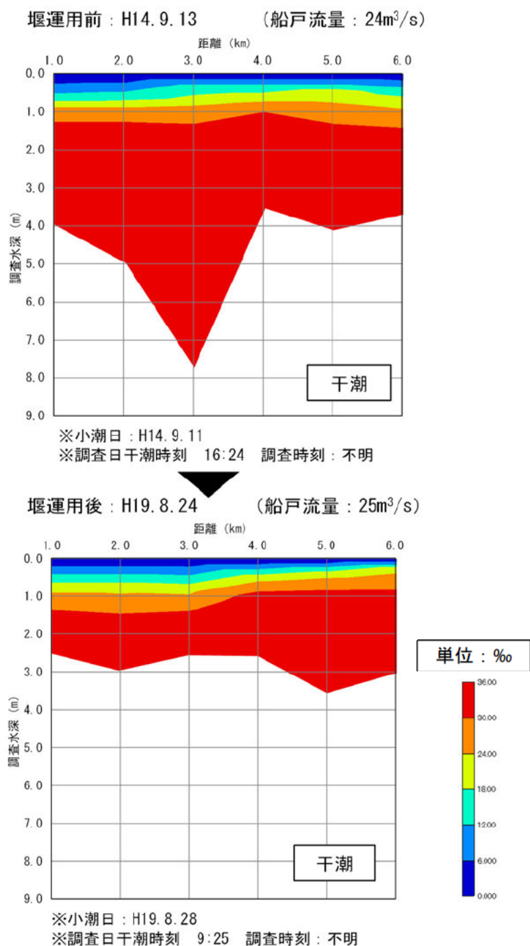
図 5.3-17 (4) 堰運用前後での塩分縦断変化の比較（小潮－干潮）（改変）
