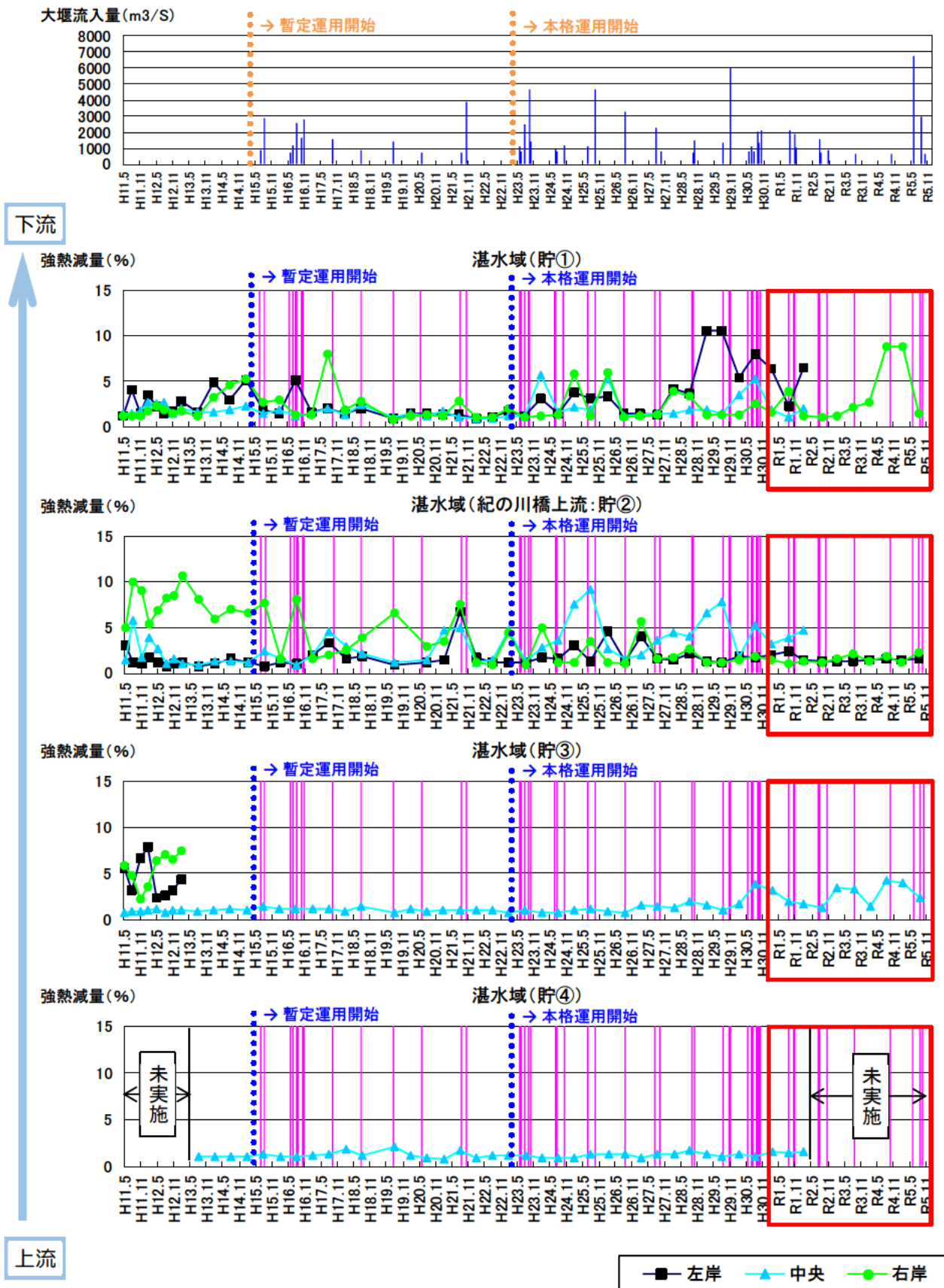
図 5.3-25 (4) 底質分析調査結果 堰～上流 (強熱減量)
