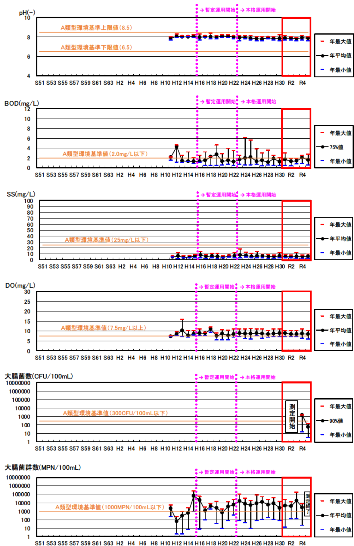
図 5.5-9 (1) 本川下流（紀の川大堰下流）地点における暫定運用開始前後の水質比較
