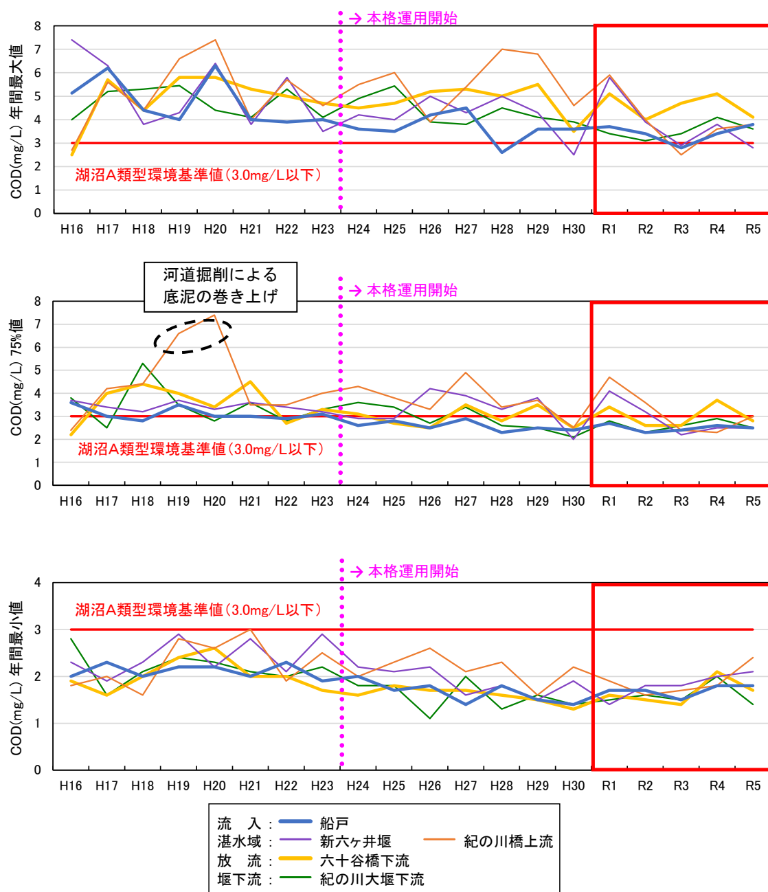
図 5.5-3 CODの経年変化
