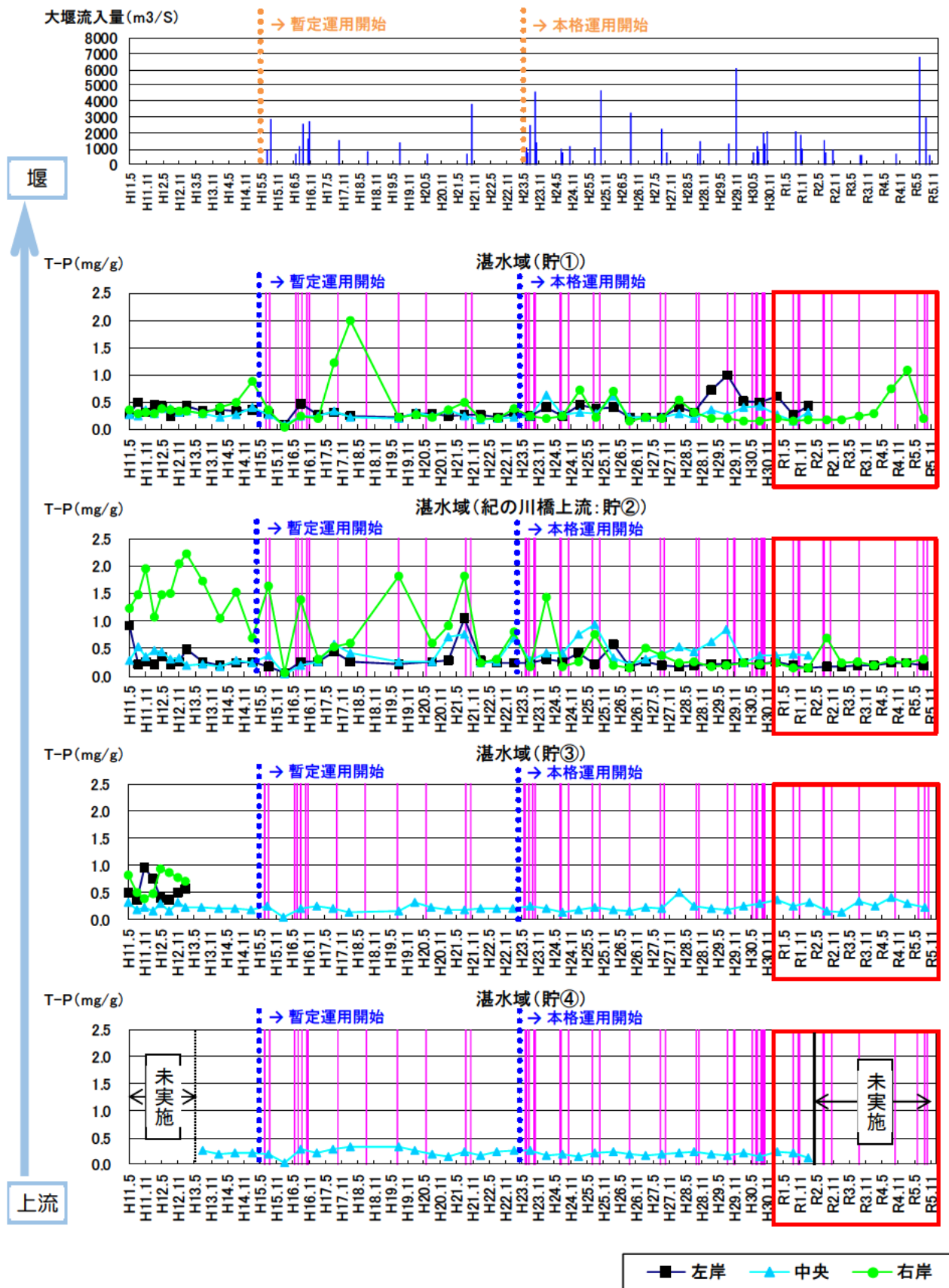
図 5.3-25 (12) 底質分析調査結果 堰～上流 (T-P)
