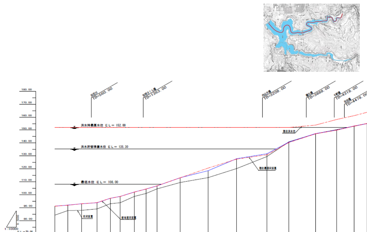
図 4.4-2 堆砂断面図（一庫大路次川）
