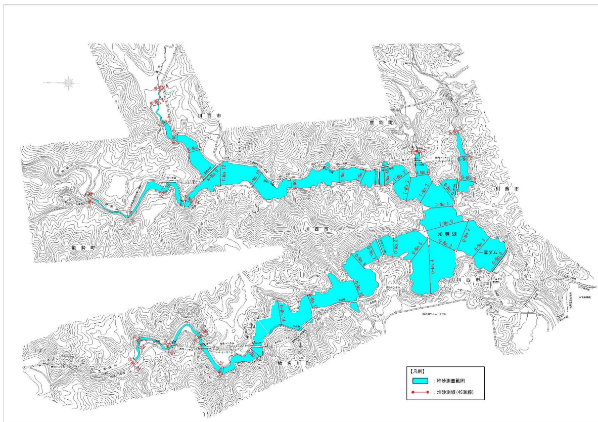
図 4.2-1 一庫ダム堆砂測量平面図(測線図)
