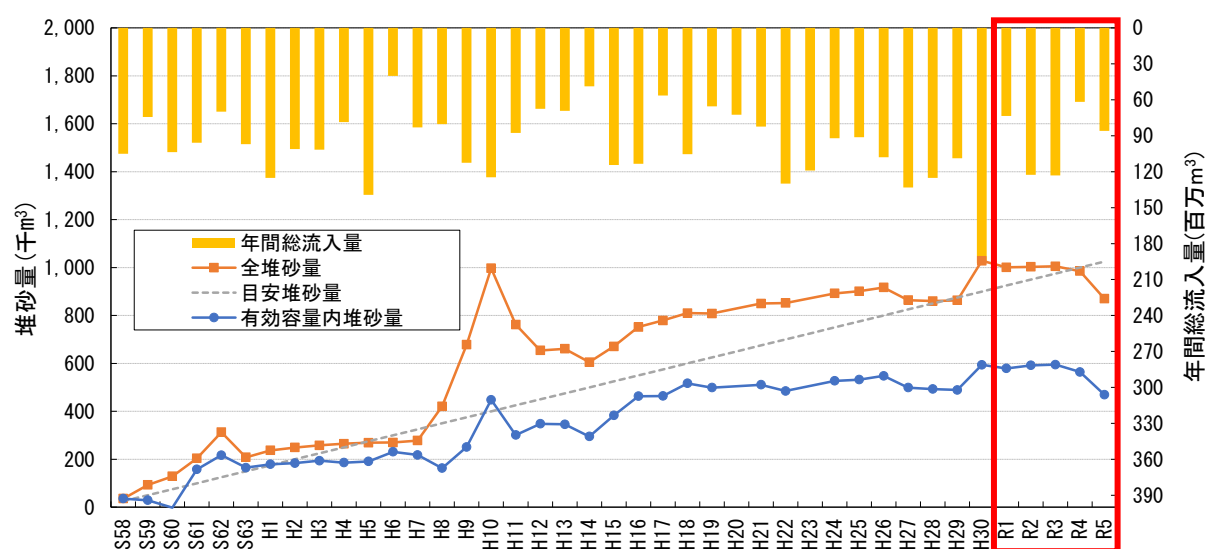
図 4.4-1 一庫ダム堆砂経年変化
