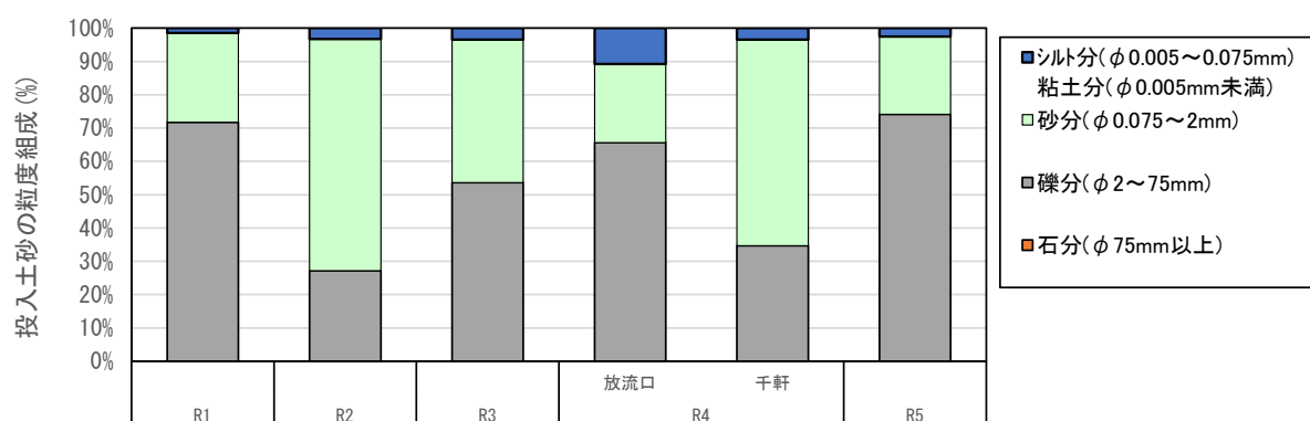
図 4.6-1 投入土砂の粒度組成
