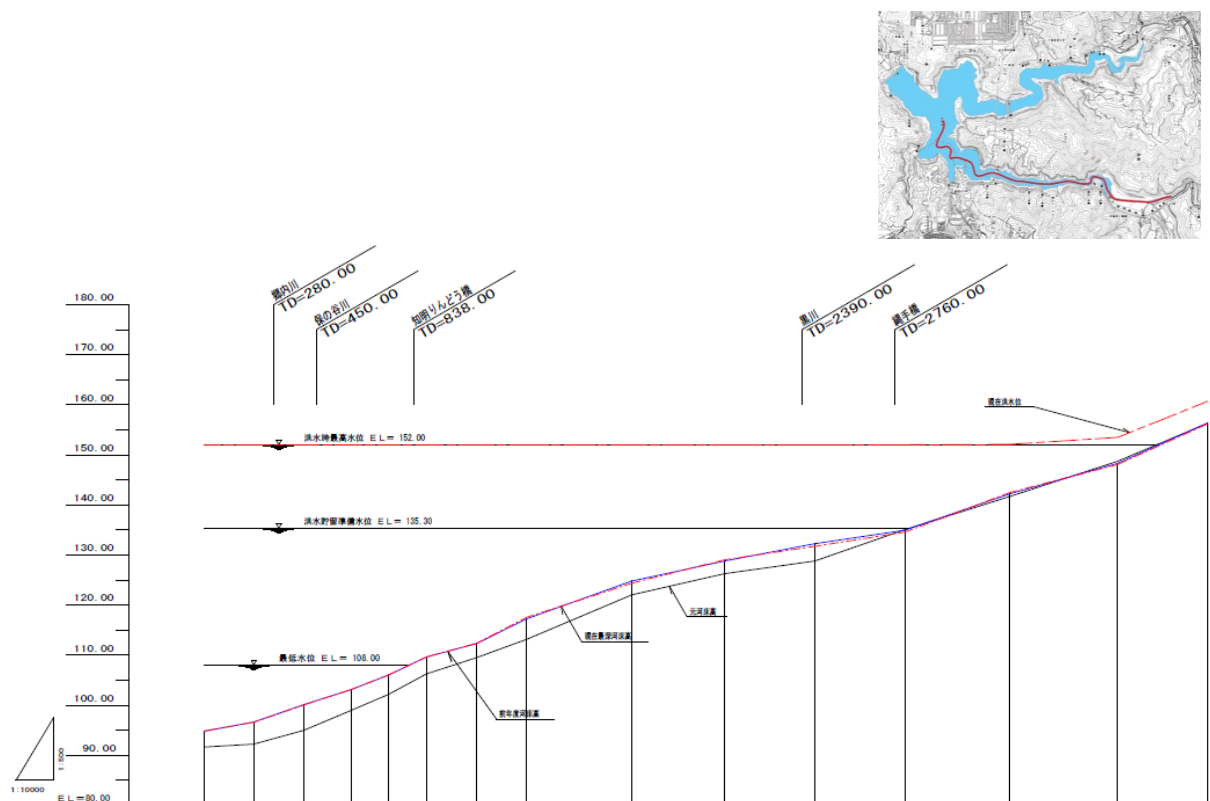
図 4.4-3 堆砂断面図（田尻川）
