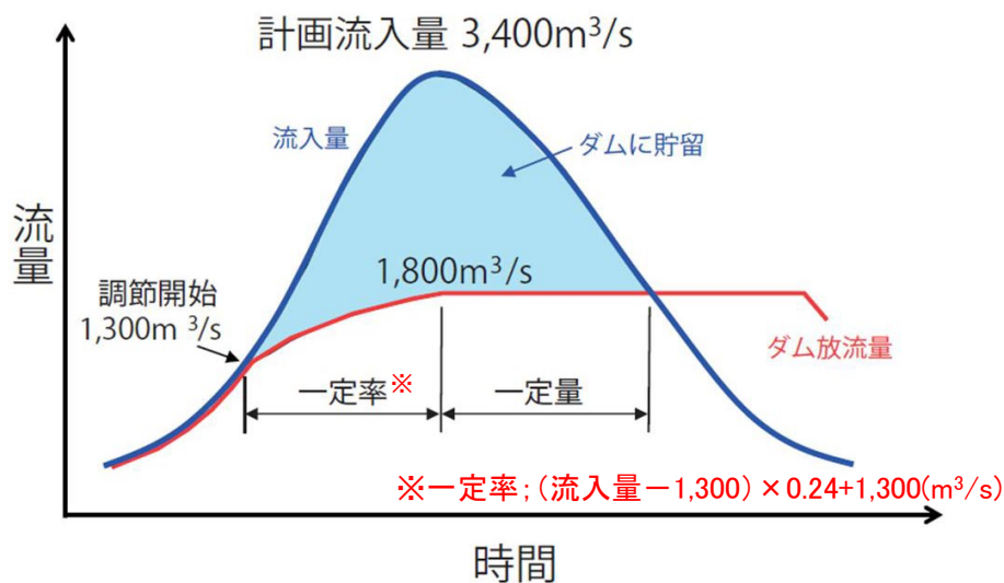
図 1.4.2-1 高山ダムの洪水調節計画
