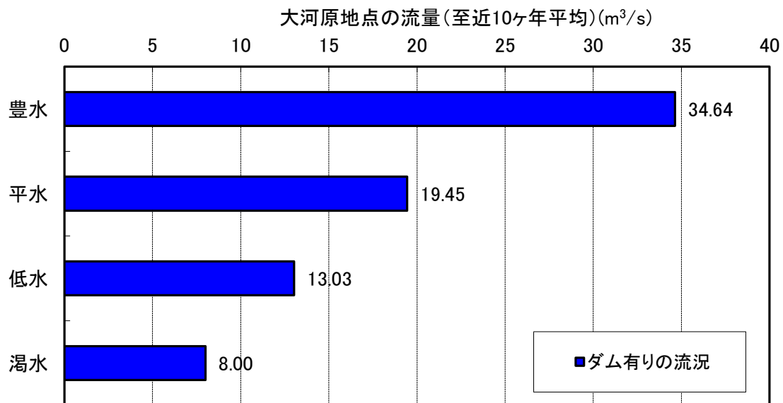
図 1.3.3-1 至近10ヶ年の大河原地点における流況
