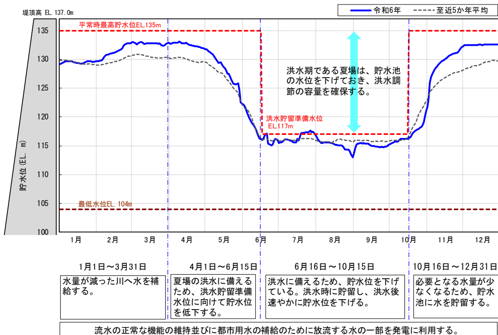
図 1.4.1-2 貯水池運用計画と実績
