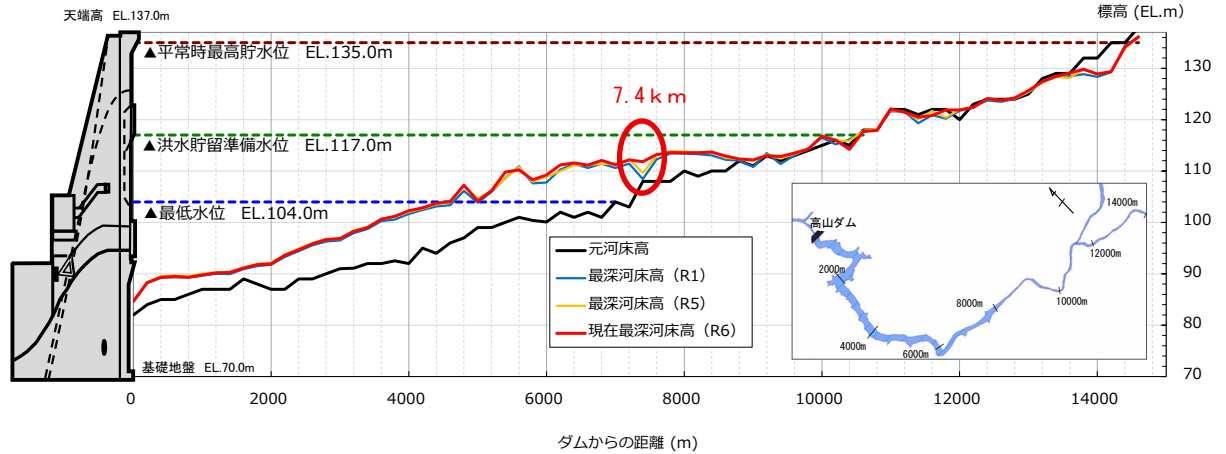
図 4.3.1-1 令和元年～令和6年の高山ダム最深河床高の比較
