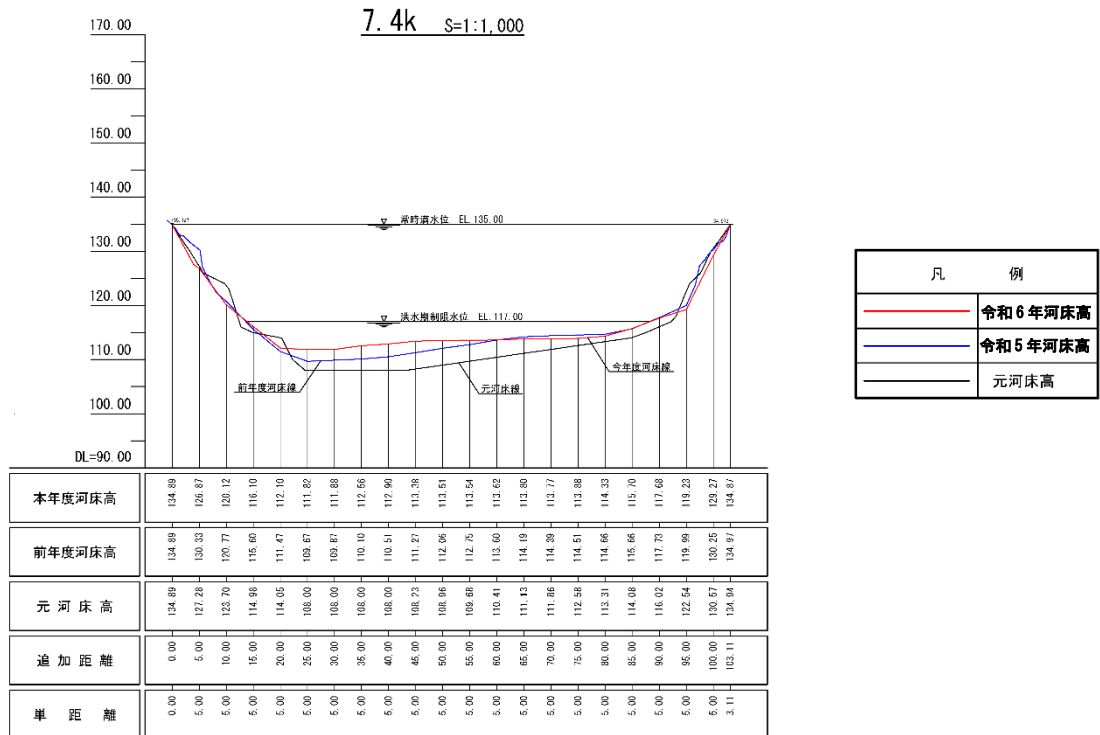
図 4.3.1-2 7.4km 横断面図 (令和6年度)
