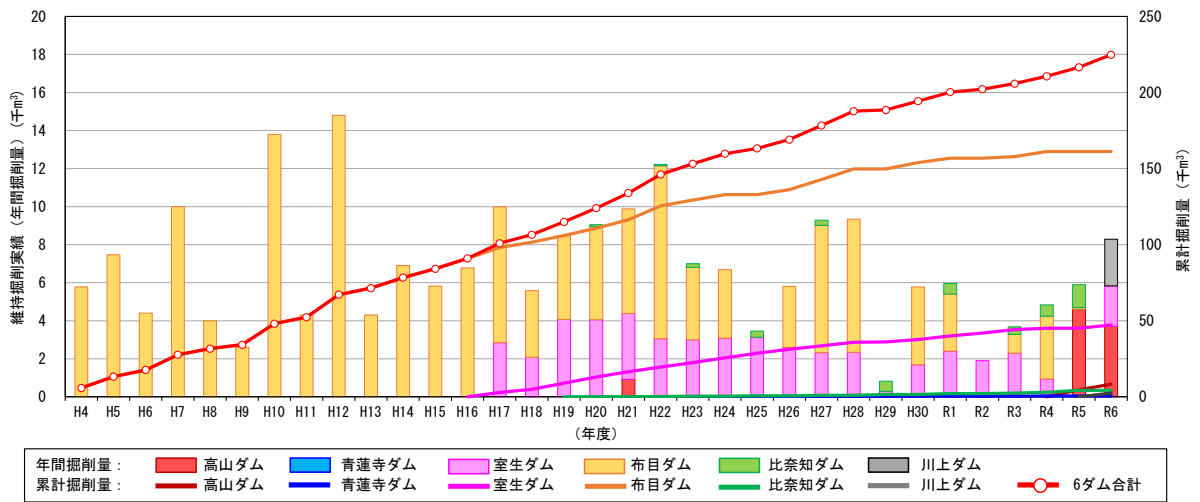
図 4.5.2-2 木津川上流ダム群 維持掘削実績
