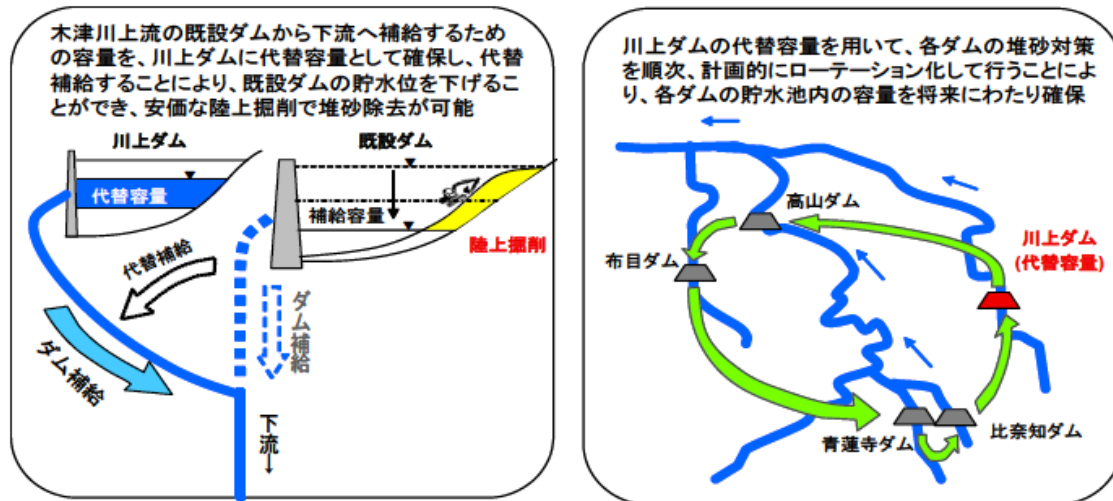
図 4.5.2-1 川上ダムの代替容量を活用した木津川上流ダム群の効率的な堆砂の除去
