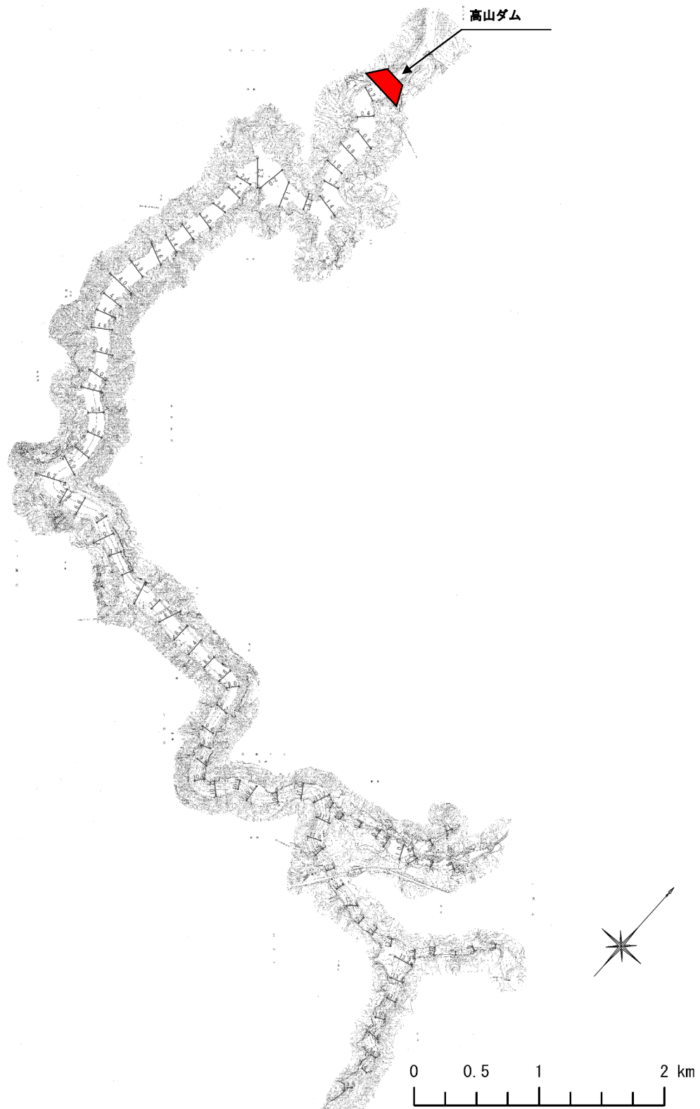
図 4.2.1-1 堆砂測量位置
