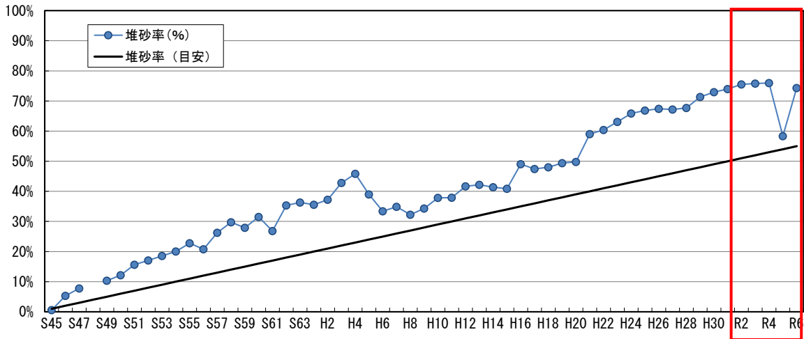
図 4.4-4.4.1-2 高山ダム堆砂率
