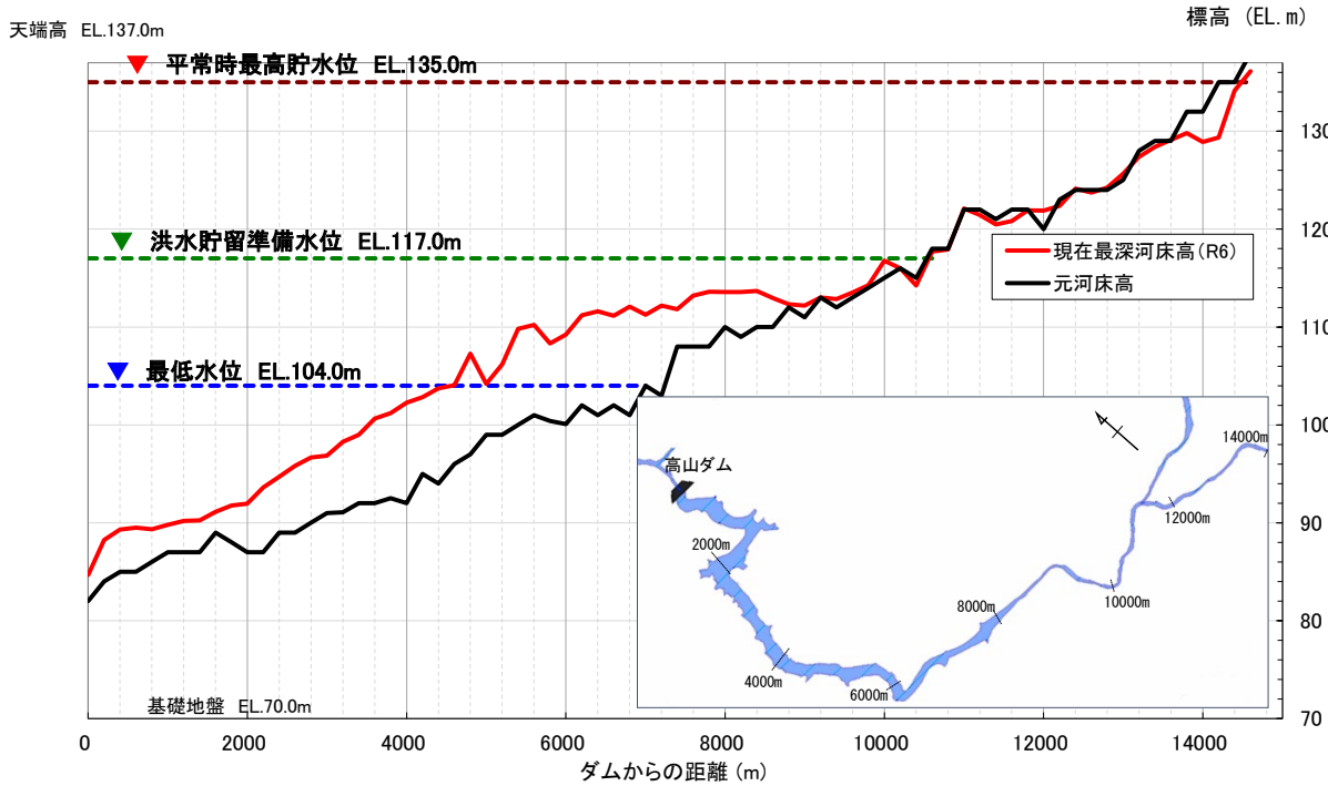
図 4.4-4.4.1-3 高山ダム貯水池内河床断面図
