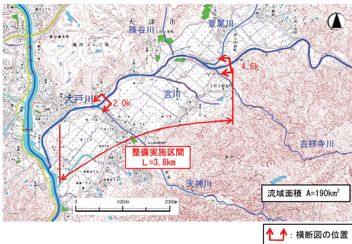
図 2.4-7 大戸川平面図
