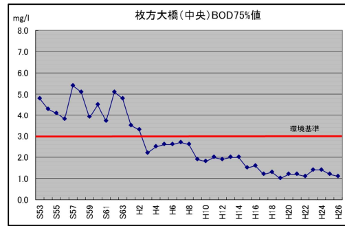
図 2.3-5 枚方大橋地点のBODの経年変化
