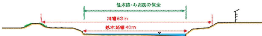
図 2.4-8 大戸川横断図
